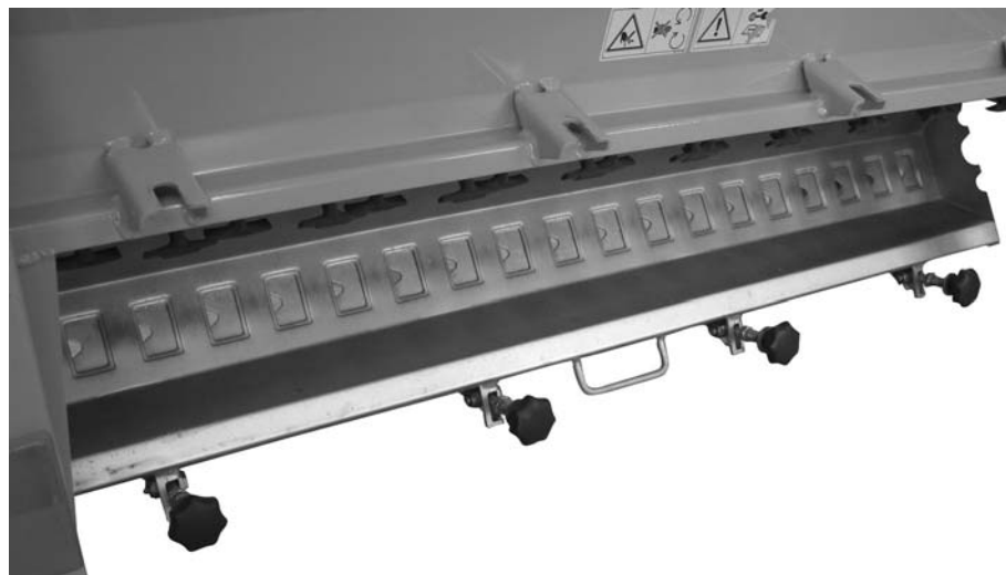
Figura 9.1: Svuotamento rapido dello spanditore per servizio invernale UKS
