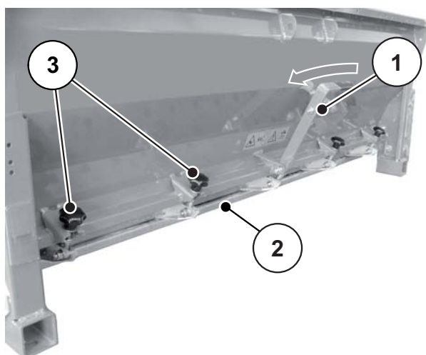
Figura 9.2: Svuotamento rapido, spandiconcime UKS GB, svitare le impugnature a stella
