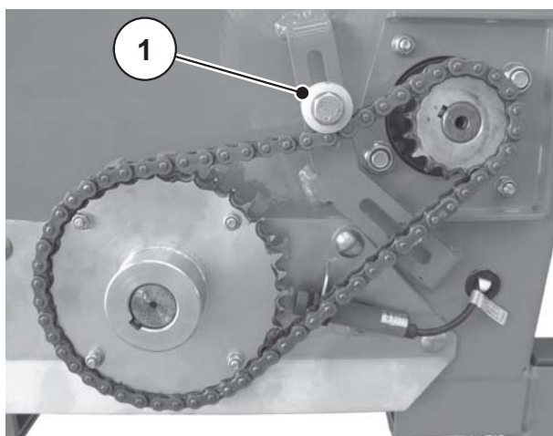
Figura 6.2: Montaggio rullo tendicatena (avviamento prese di forza a rotazione sinistra)
