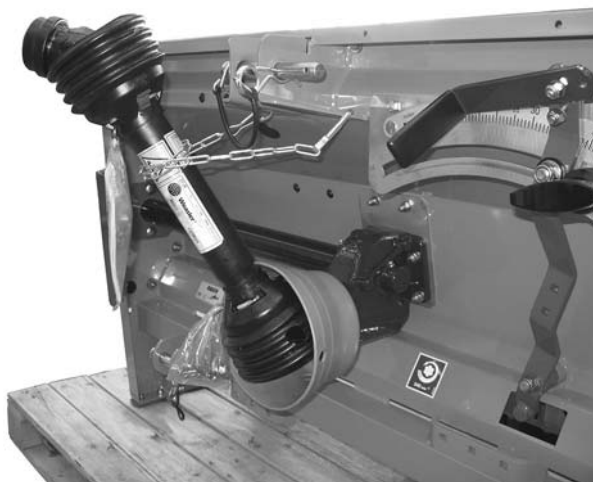
Figura 6.7: Sostenere l'albero cardanico
