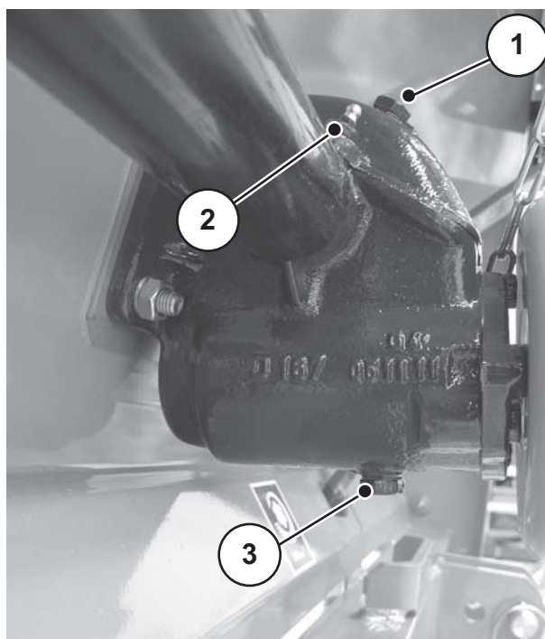
Figura 10.2: Punti di rifornimento e scarico dell'olio del riduttore
