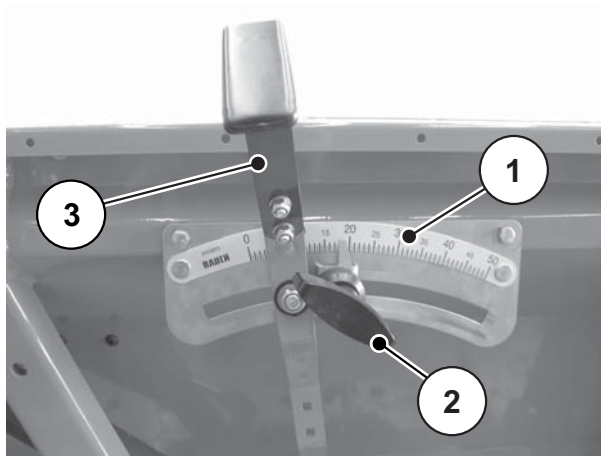
Figura 7.1: Regolazione dei dosatori
