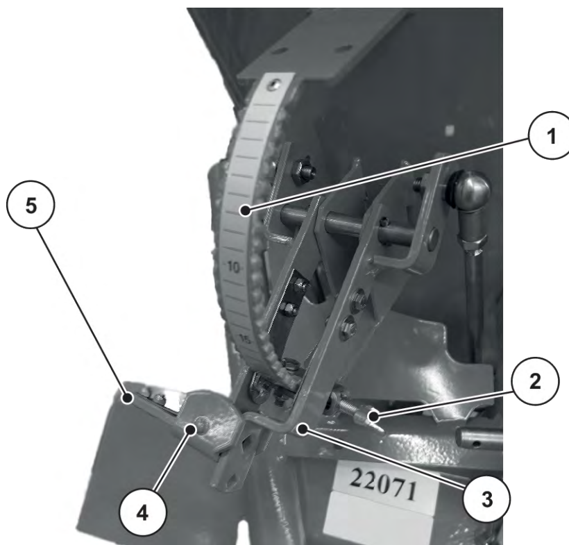
III. 25: Scala per la regolazione della dose
