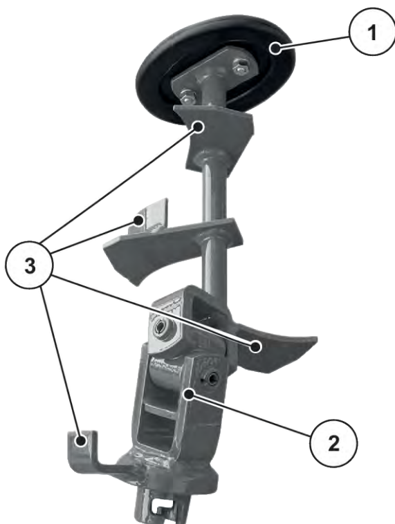
III. 29: Agitatore RWK 10
