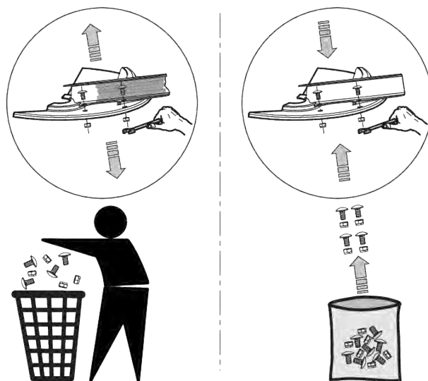
III. 33: Utilizzo di dadi autobloccanti nuovi
