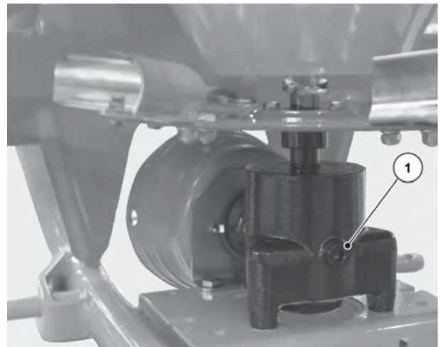
Ill. 34: Vite per il controllo del livello olio del cambio
