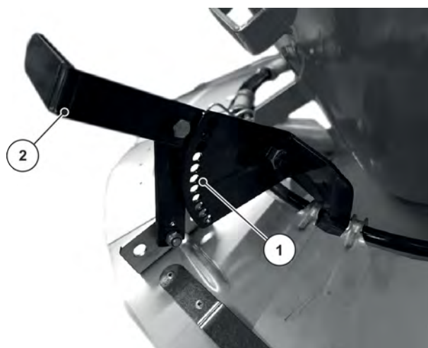
Att. 32: Izkliešanas platuma ierobežojums
