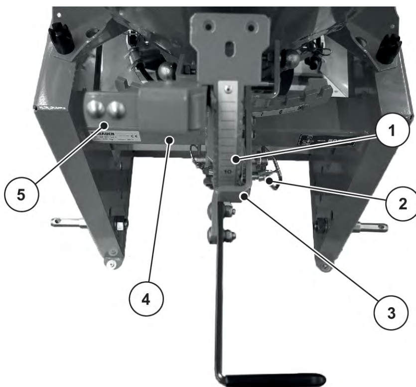
Att. 29: Izkliedēšanas daudzuma iestatījums
