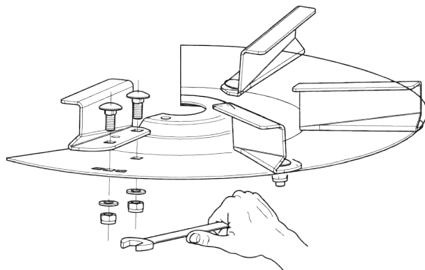
Att. 40: Atbrīvojiet izsviedējlāpstiņu skrūves.
