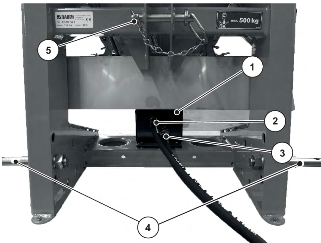
Att. 8: Konstruktijas grupu pārskats - priekšpuse
