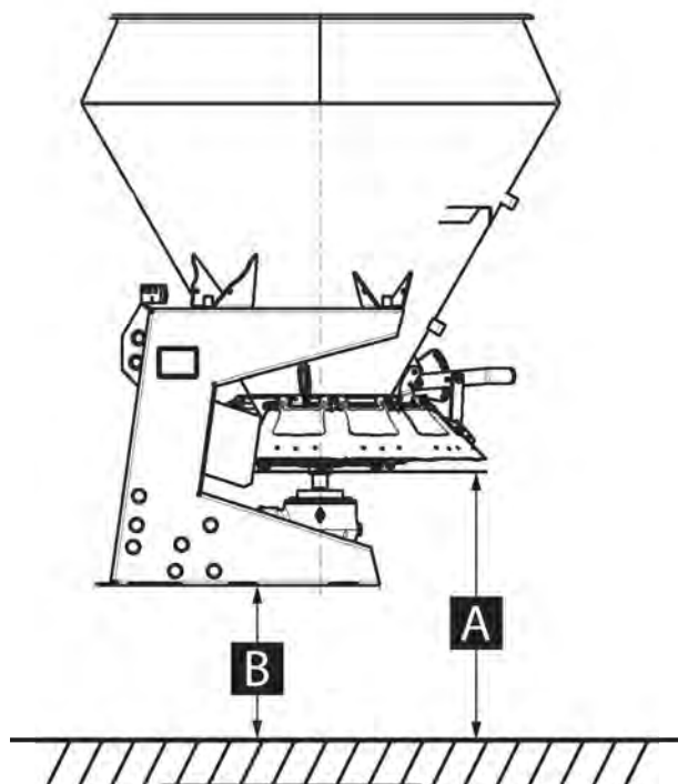
Att. 21: Uzķabināšanas augstuma noteikšana
