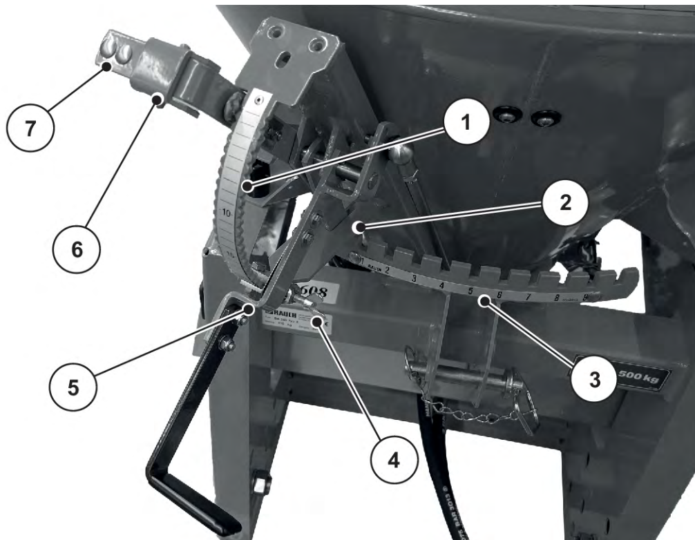
Att. 27: Mašīnas iestatīšanas elementi, priekšpuse
