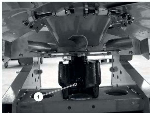
Att. 42: Transmisijas eļļas līmeņa kontrolskrūve
