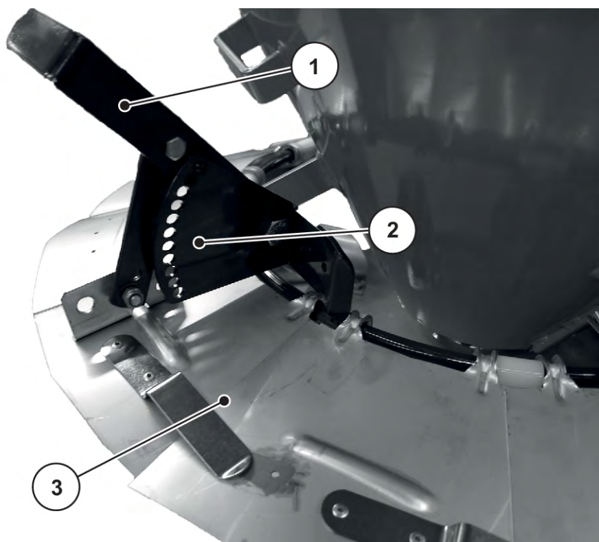
Obr. 26: Omezení šířky rozmetání
