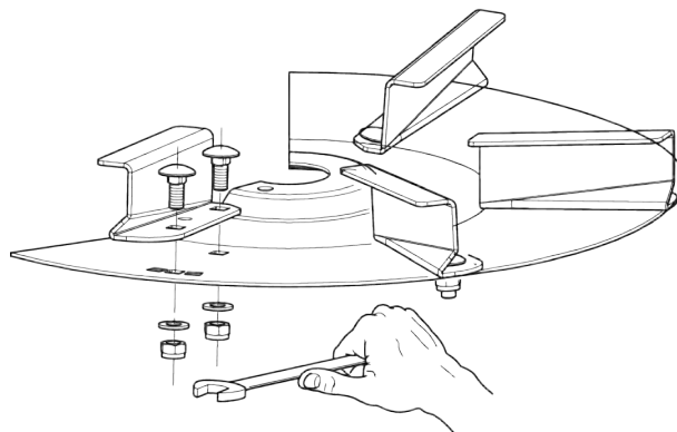
Obr. 32: Povolte šrouby rozmetací lopatky.
