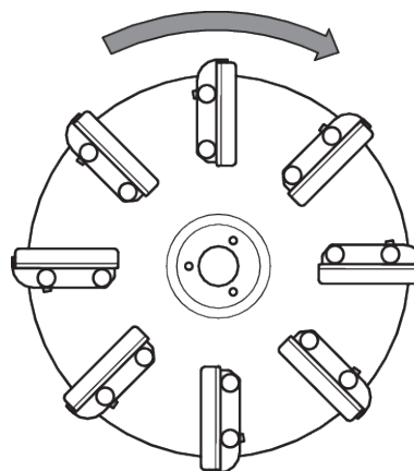
Obr. 21: Směr otáčení rozmetacího disku
