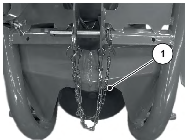
Obr. 27: Držák kloubového hřídele - dlouhý řetěz
