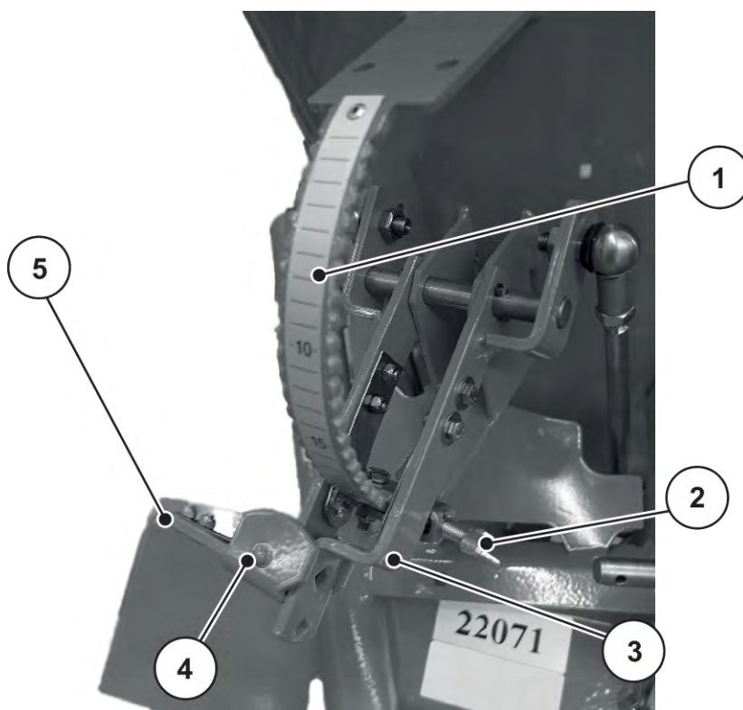
Fig. 25: Skala för inställning av utmatningsmängd
