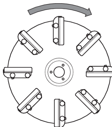
Fig. 21: Sens de rotation du disque d'épandage
