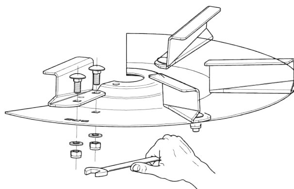
Fig. 32: Dévisser les vis de la palette
