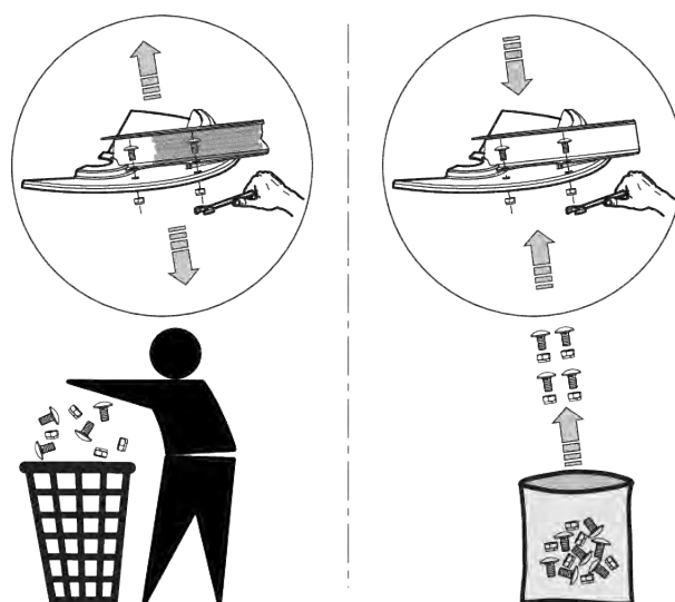
Fig. 33: Utiliser de nouveaux écrous autobloquants
