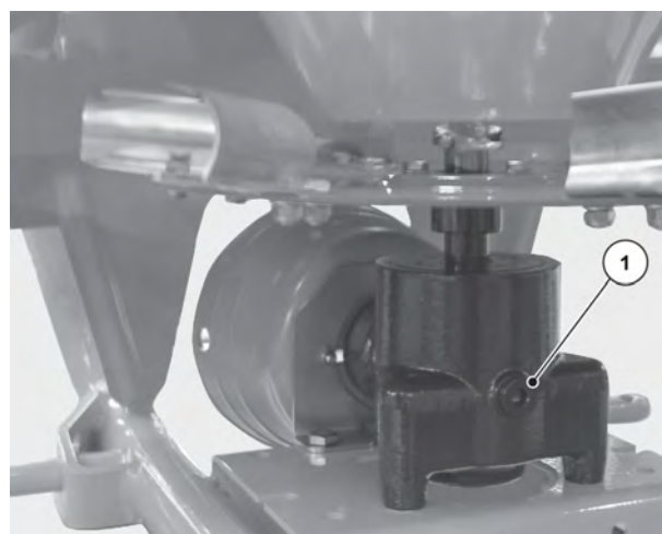
Fig. 34: Vis de contrôle pour faire le niveau d'huile
