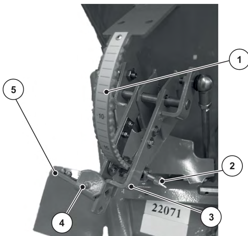
Fig. 25: Échelle graduée pour le réglage de la dose d'épandage
