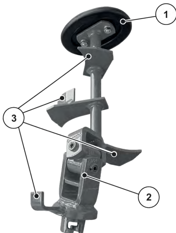
Fig. 29: Agitateur RWK 10
