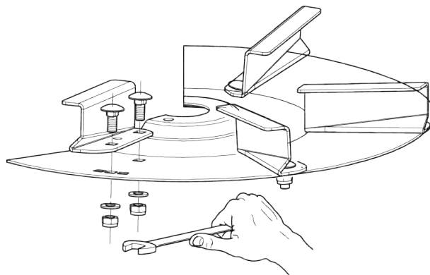
Fig. 40: Løsning af skruerne på spredvingen
