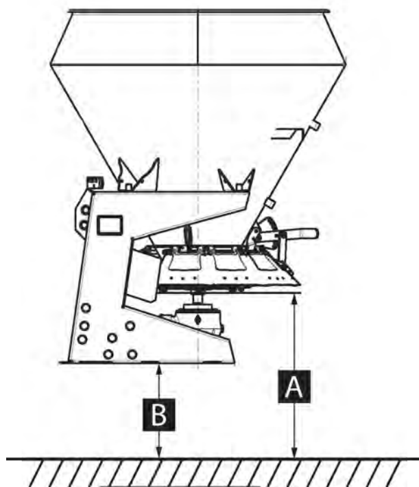
Fig. 21: Bestemmelse af monteringshøjden
