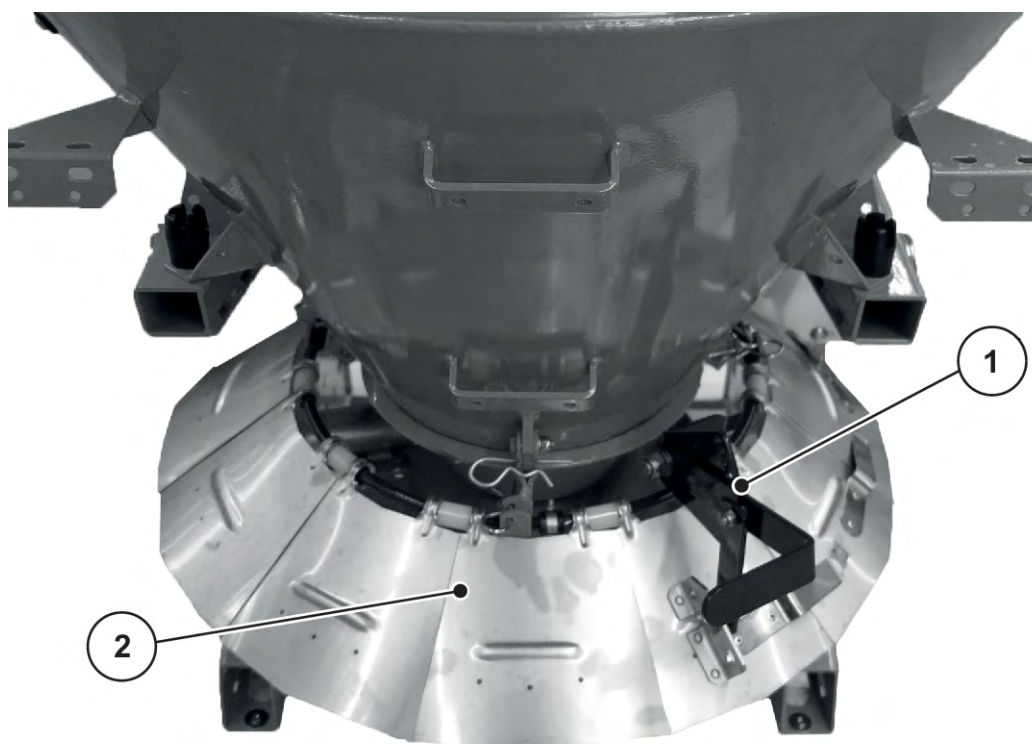
Fig. 28: Indstilling af spreddebreddebegrænsningen
