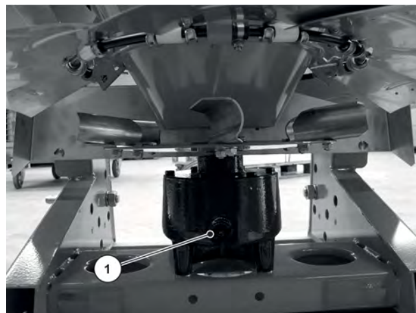
Fig. 42: Kontrolskrue oliestand gearolie
