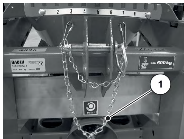
Fig. 37: Kardanaxselholder, lang kæde
