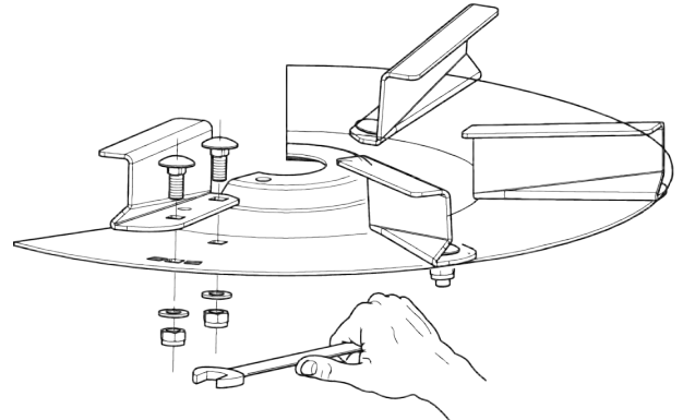
Kuva 40: Levityssiiven ruuvien irrotus
