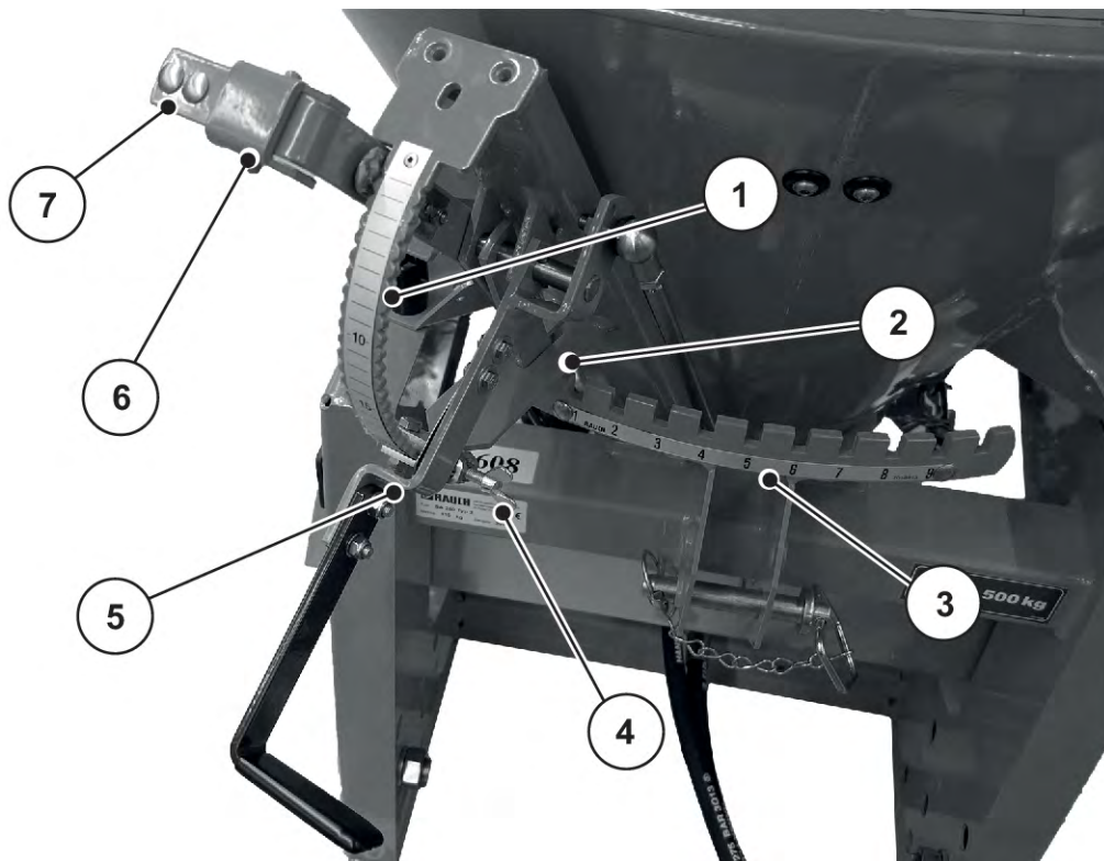
Kuva 27: Koneen säätöosat etuosassa
