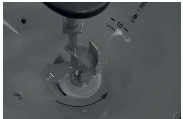
Kuva 23: Sekoitin asennettuna
