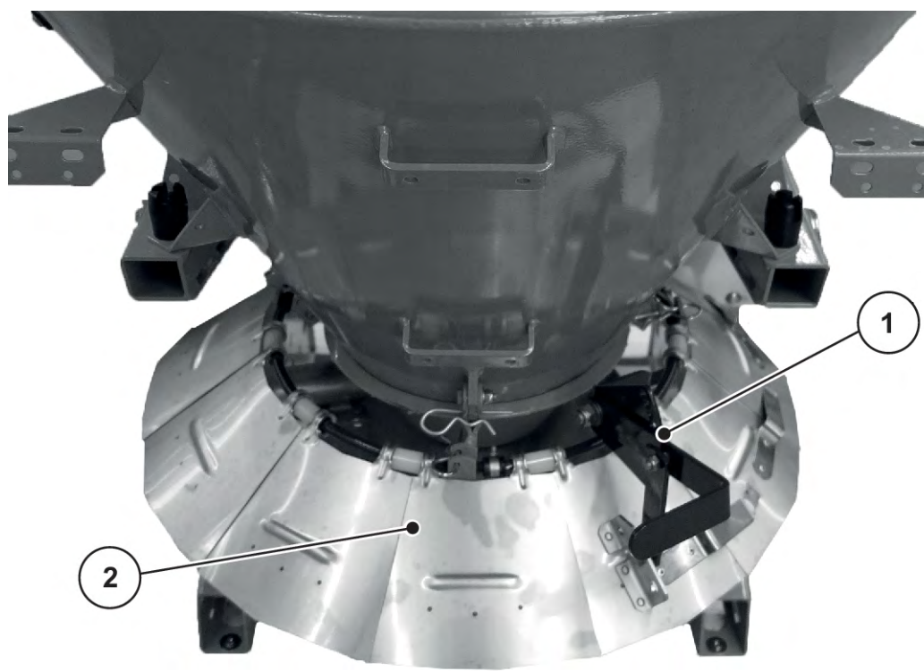
Kuva 28: levityslevyden rajoituksen säätö
