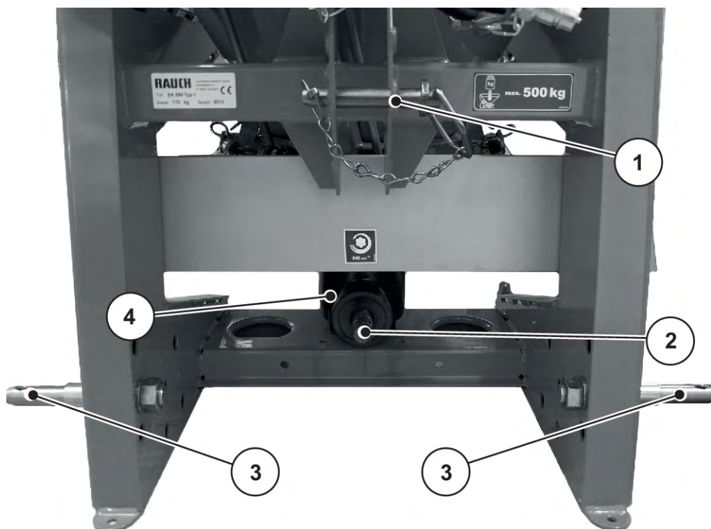
Kuva 7: Rakenneryhmäkuva – takaosa
