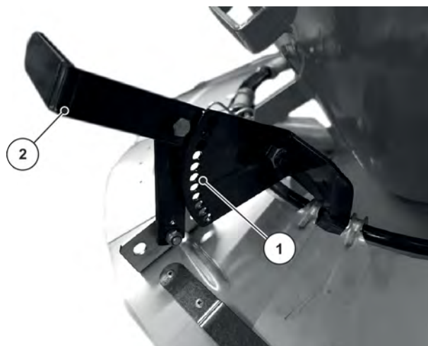
Kuva 32: Levitysleveyden rajoitus
