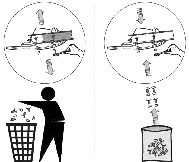
Kuva 41: Uusien itselukittuvien mutterien käyttö
