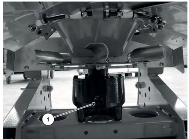
Kuva 42: Vaihteistoöljyn öljymäärän tarkistusruuvi
