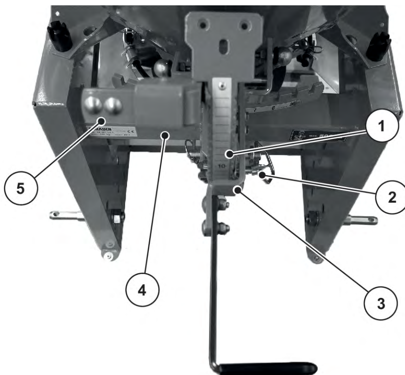
Kuva 29: Levitysmäärän asetus
