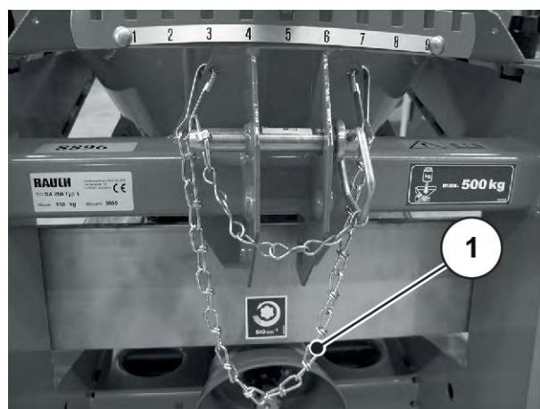
Kuva 37: Nivelakselin säilytyspaikan pitkä ketju
