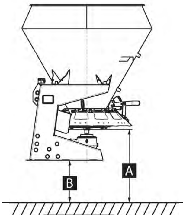
Kuva 21: Asennuskorkeuden määrittäminen
