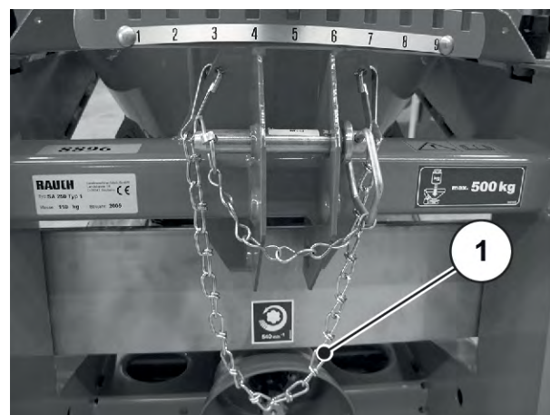
III. 37: Catena lunga supporto albero cardanico
