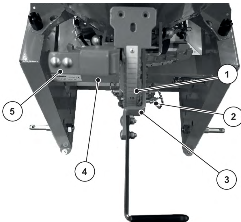
Ill. 29: Regolazione della quantità di spargimento
