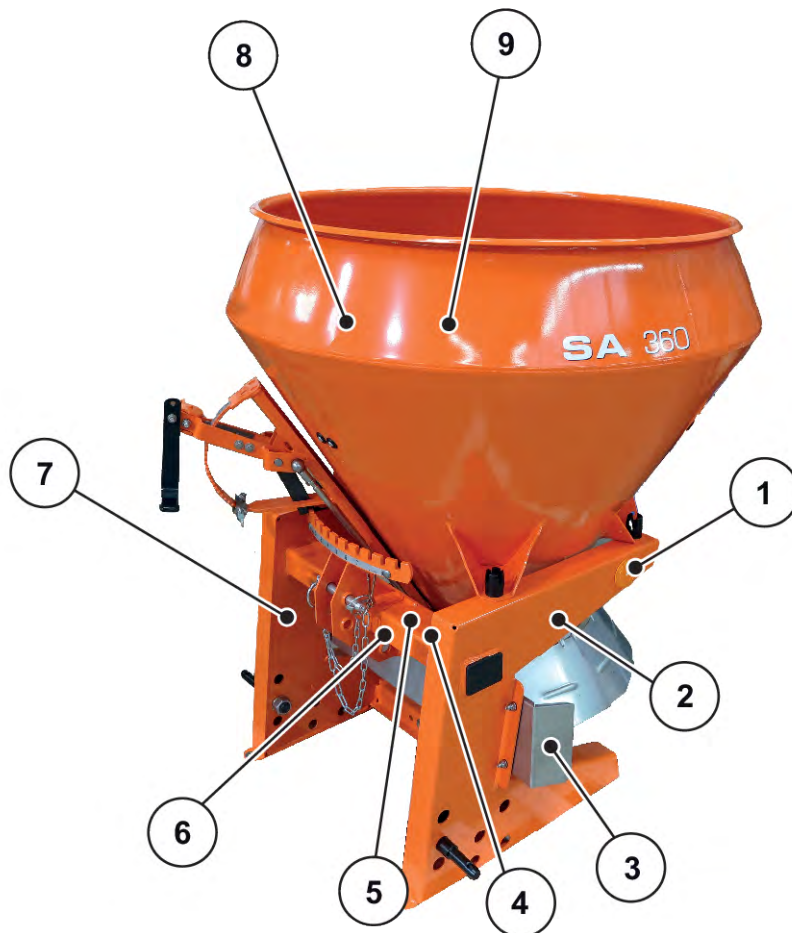
III. 2: Posizione dei dispositivi di protezione e degli adesivi con avvertenze e istruzioni
