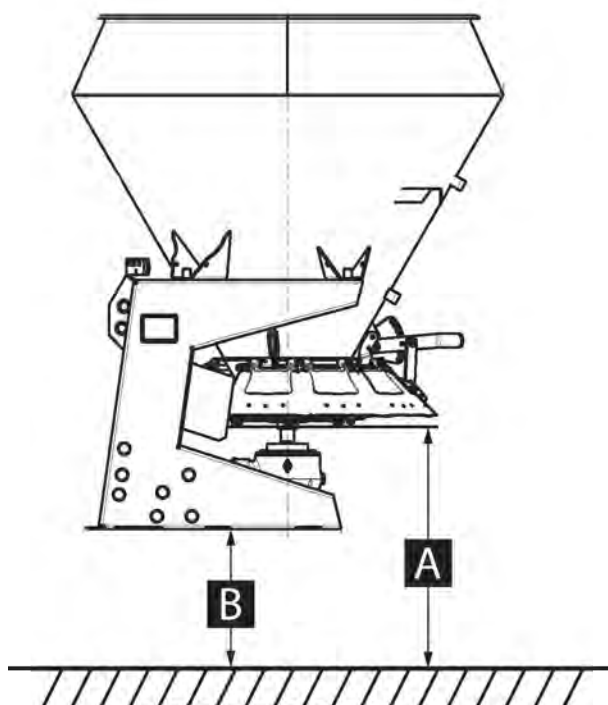
III. 21: Determinare l'altezza di montaggio
