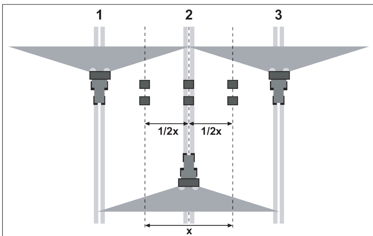
III. 35: Disposizione per tre traversate
