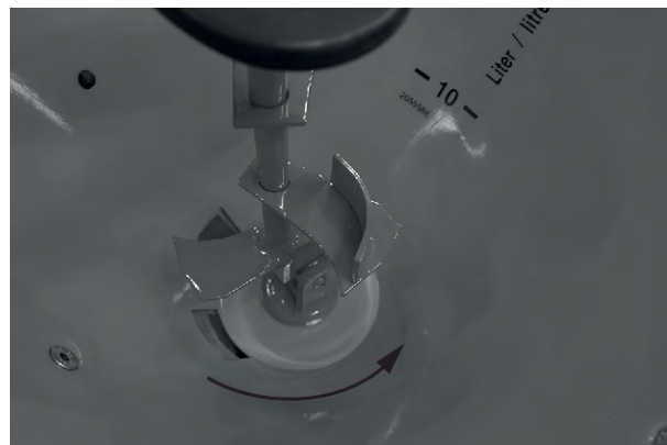
III. 23: Agitatore montato
