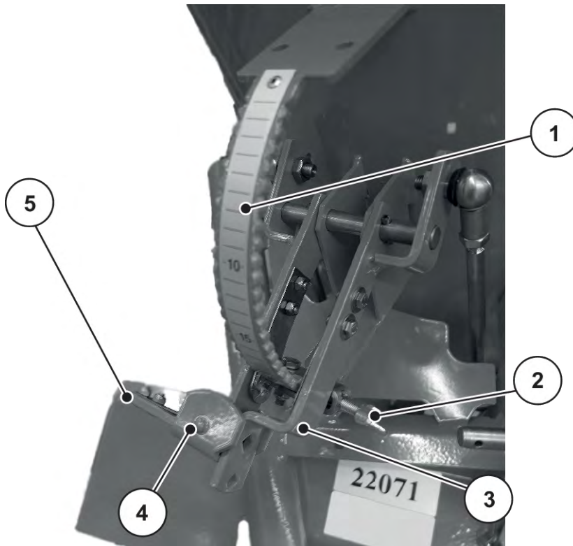
Abb. 25: Skala zur Einstellung der Ausbringmenge
