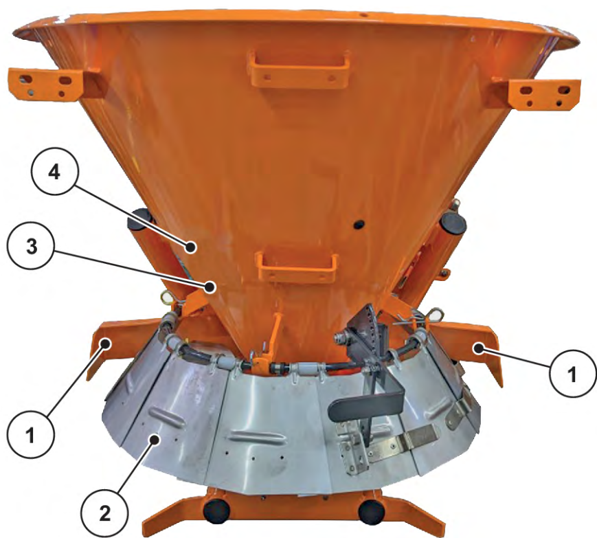
Abb. 4: Schutzeinrichtungen, Aufkleber Warn- und Instruktionshinweise, Rückseite
