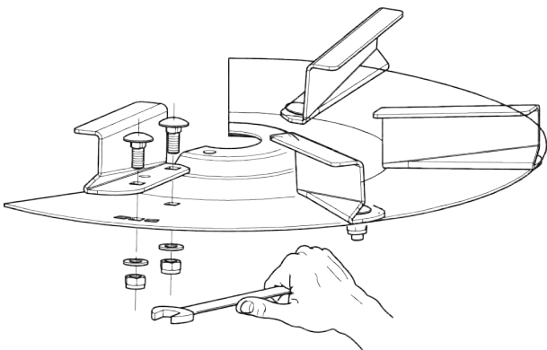
Abb. 32: Schrauben der Wurfflügel lösen
