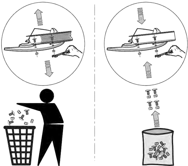
Abb. 33: Neue selbstsichernde Muttern verwenden
