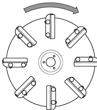
Abb. 21: Drehrichtung der Wurfscheibe
