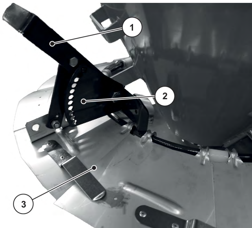
Abb. 26: Streubreitenbegrenzung
