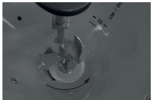
Abb. 20: Rührwerk montiert
