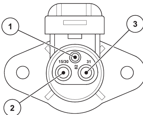
Kuva 9: PIN-käyttö virtapistoke
