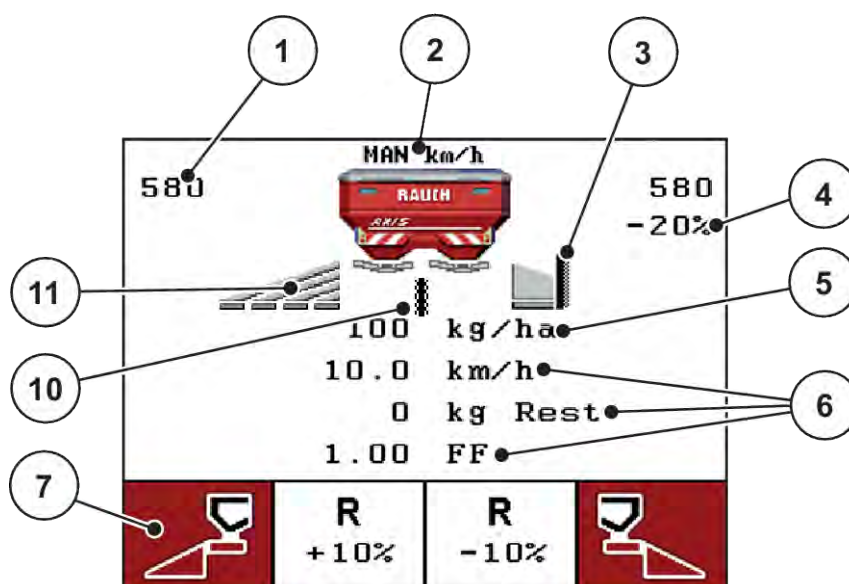
Sl. 3: Zaslon upravljačke jedinice – primjer radnog zaslona na AXIS-M
