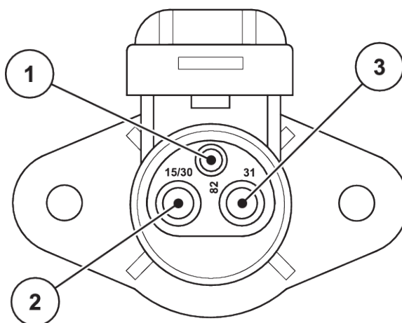
Рис. 9: Назначение PIN в штепсельной розетке питания
