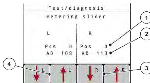
Afb. 43: Test/diagnose; voorbeeld: Doseerschuij
