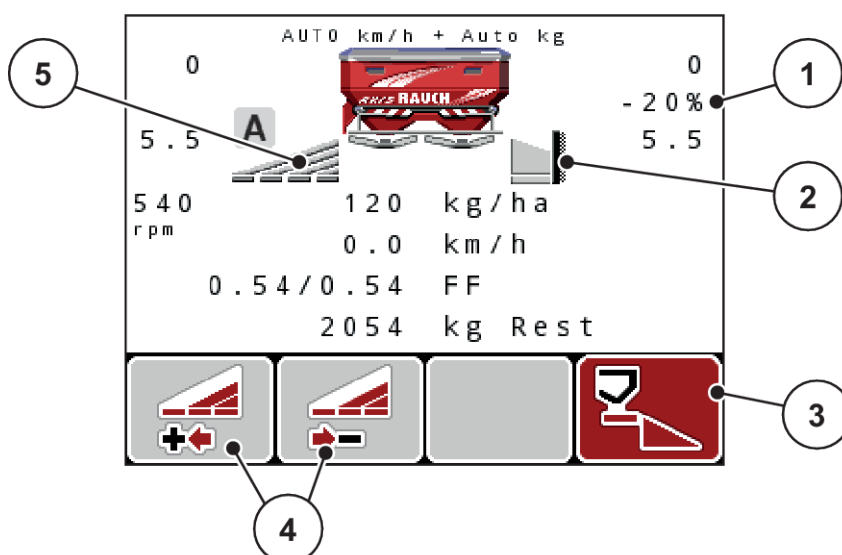
Afb. 53: Werkscherm een deelbreedte links, grensstrooizijde rechts
