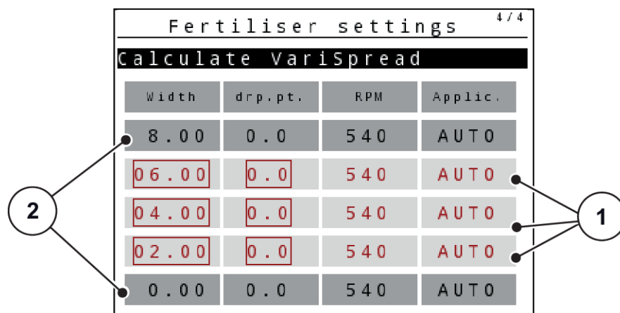
Afb. 30: VariSpread berekenen, voorbeeld met 8 deelbreedtes (4 aan elke zijde)
