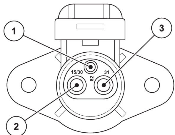
Abb. 9: PIN-Belegung Stromsteckdose
