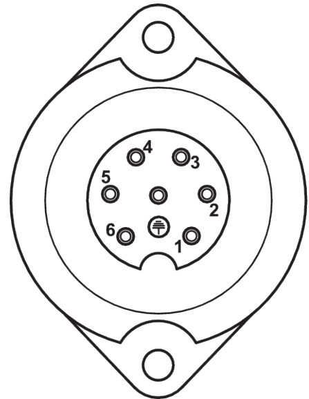
Abb. 10: PIN-Belegung der 7-poligen Steckverbindung
