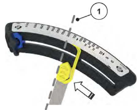
그림 70: 위치 표시기 이동
