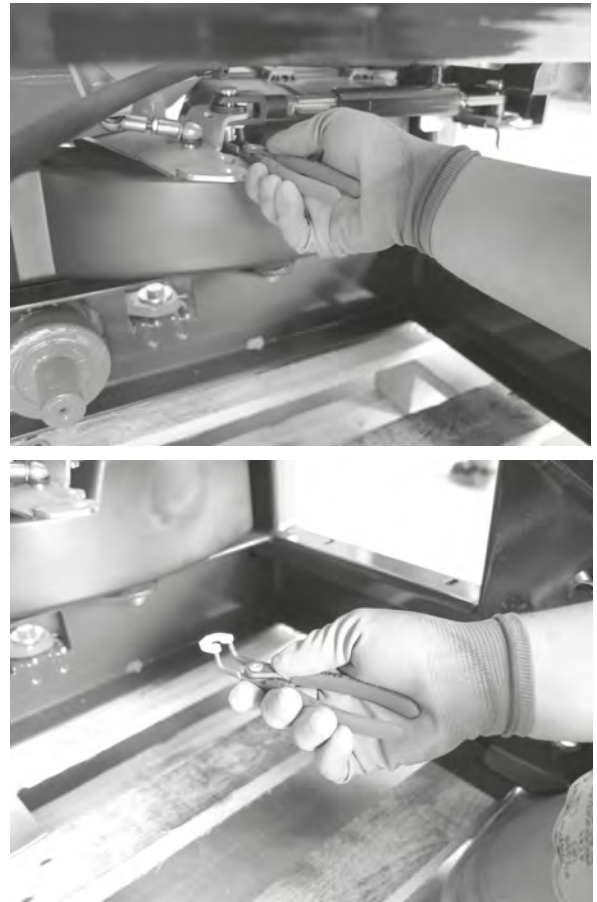
그림 68: 실린더를 분리합니다.
