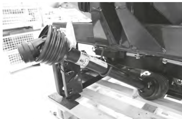
그림 18: 카르단 축 홀더
