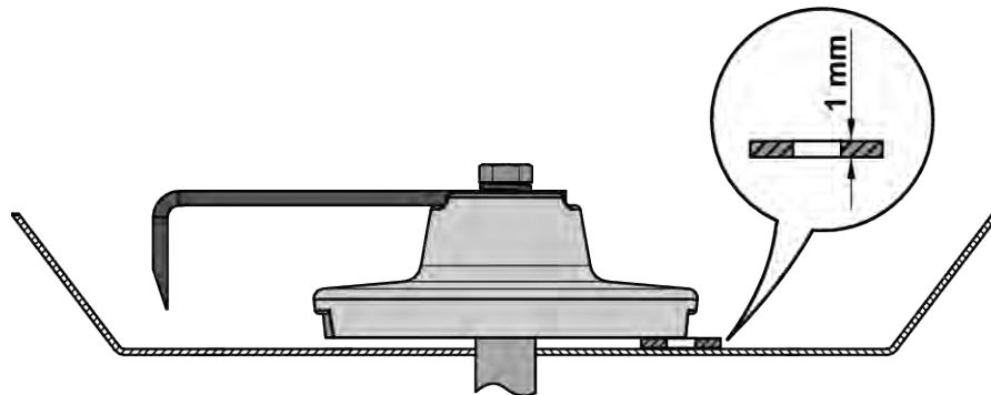
그림 76: 교반기 설정
