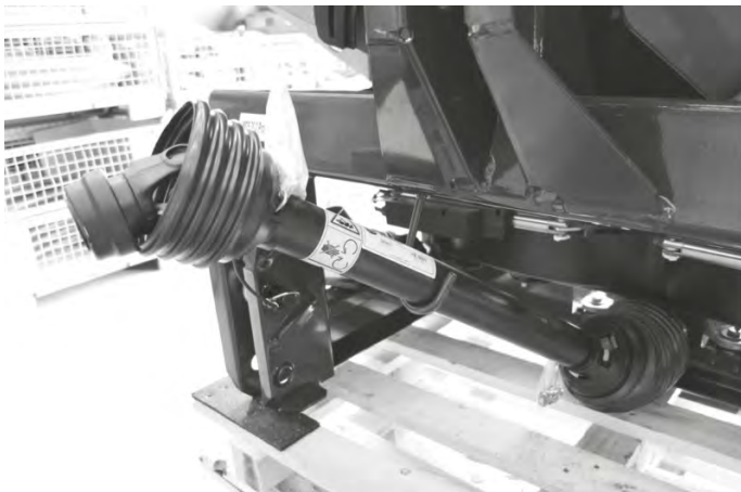
그림 60: 카르단 축, 케이블 및 유압 호스 보관하기
