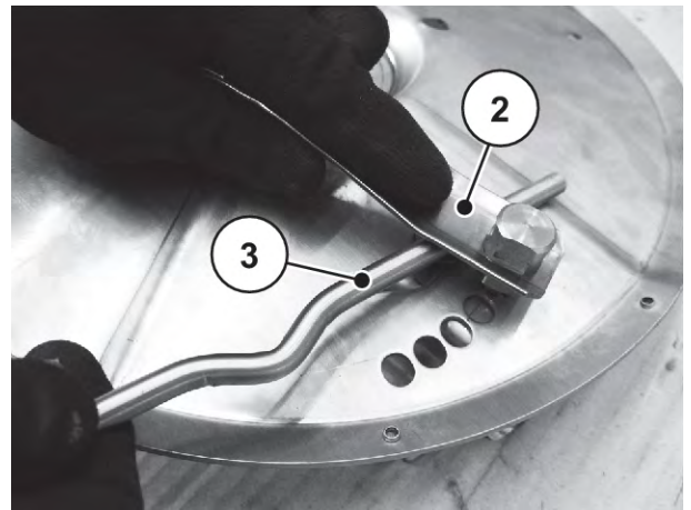
그림 79: 판 스프링 풀기
