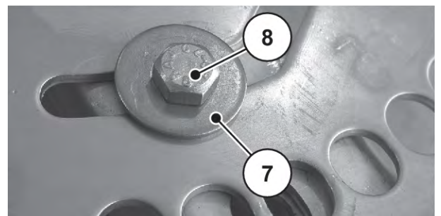
그림 82: 투척 블레이드의 고정점
