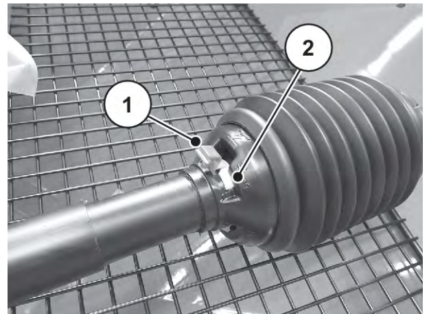
그림 13: 카르단 축 보호 커버를 엽니다.
