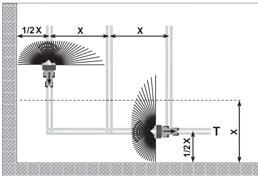
그림 55: 경계 살포
