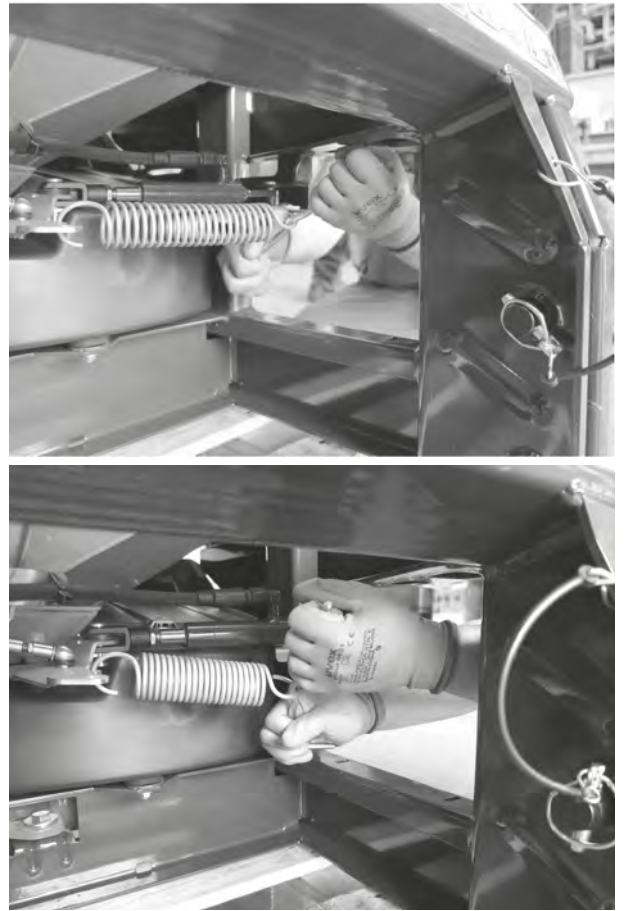
그림 67: 스프링 풀기
