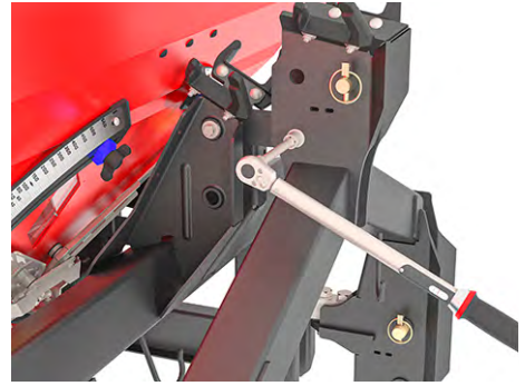
그림 62: 텐션 로드를 계량 프레임에 고정하기
