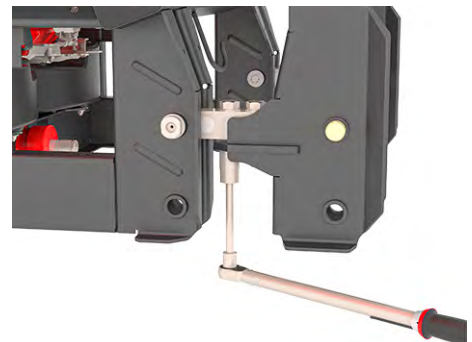
그림 61: 로드셀 고정(주행 방향 오른쪽)
