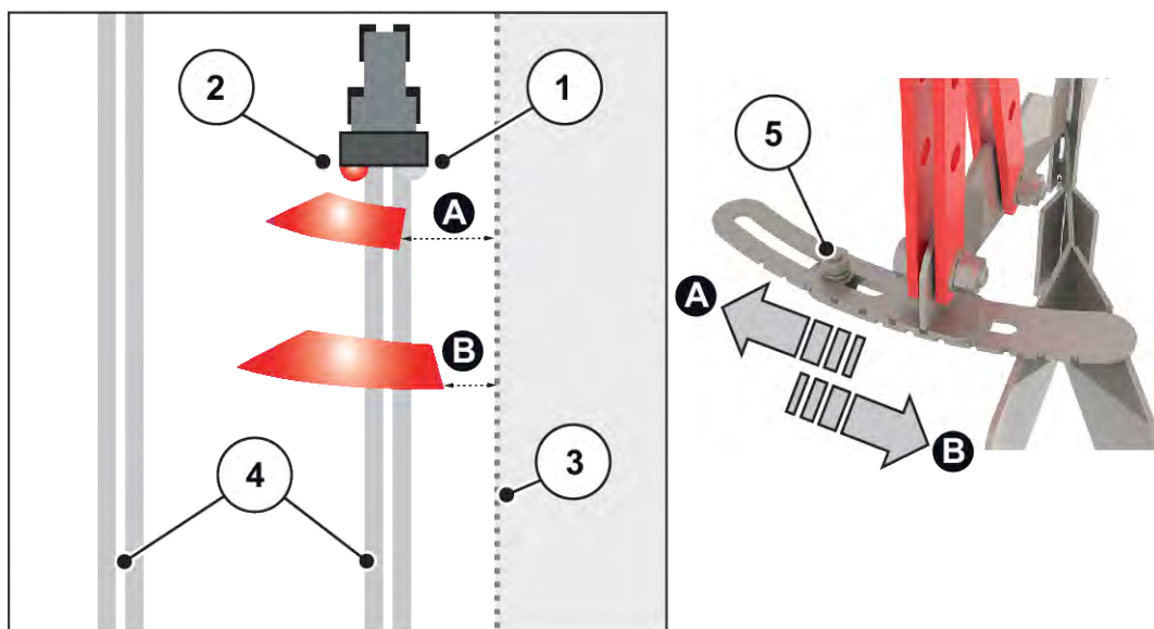
그림 52: 경계 살포 장치의 설정
