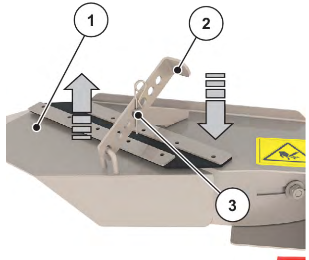
그림 59: 줄 살포장치에서 조정
