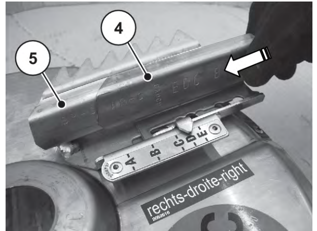
그림 81: 새 연장 블레이드
