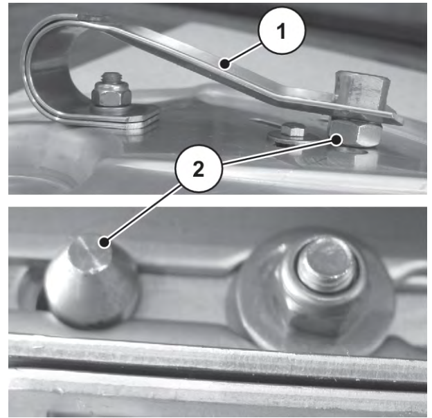
그림 75: 잠금 볼트 올바른 고정
