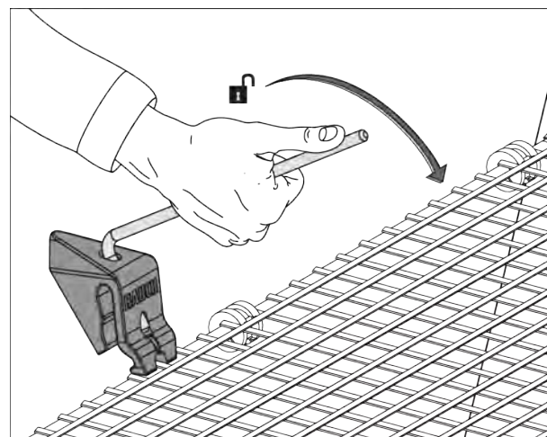
그림 64: Opening the protective grid lock
