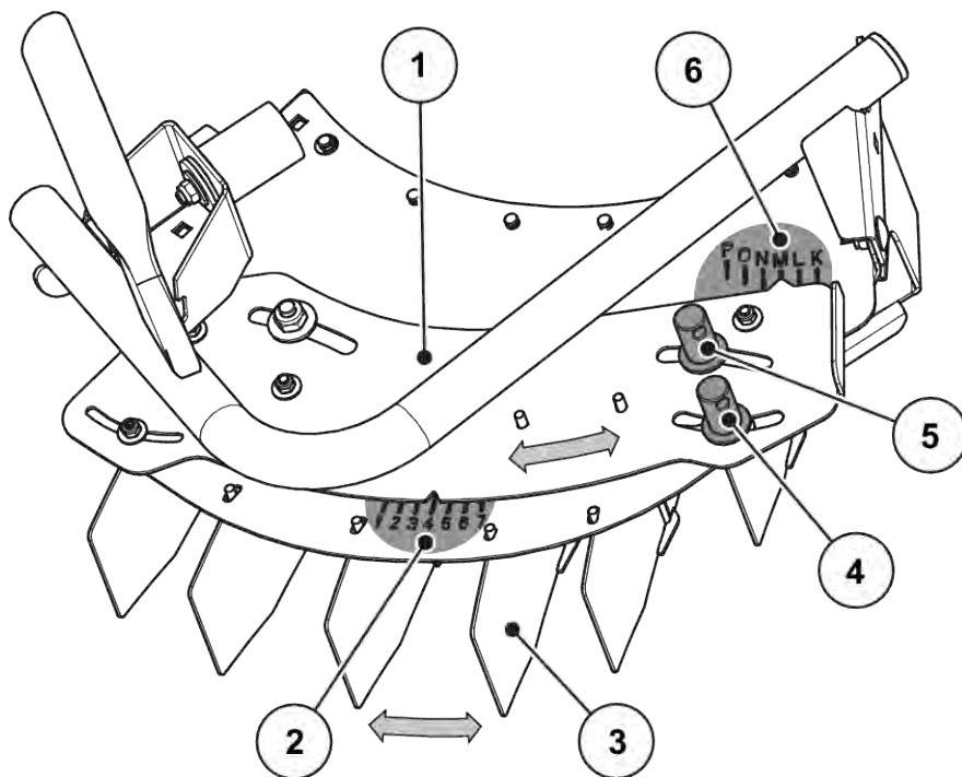
그림 53: TELIMAT 장치 설정
