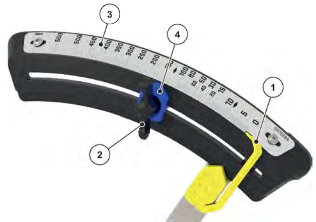
그림 41: 살포량 설정용 눈금(주행 방향 오른쪽, 버전 K/D/C)
