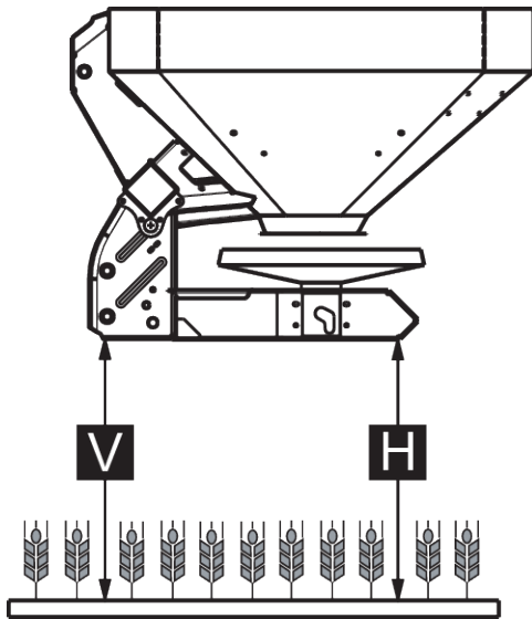
그림 26: 일반 시비와 추비에서 최대 허용 장착 높이
