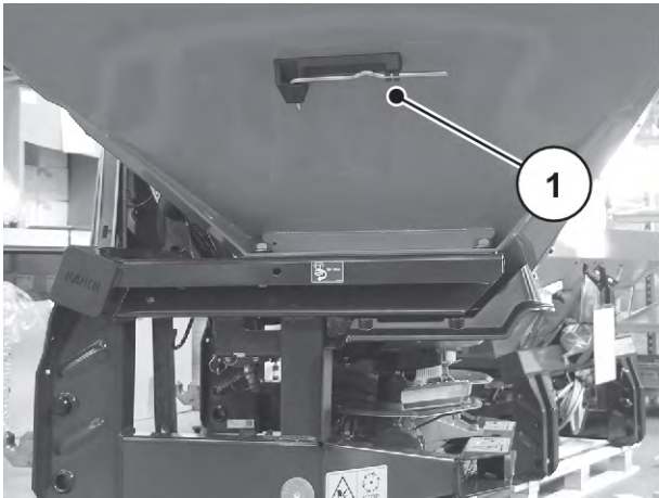
그림 10: 조정 레버의 위치
