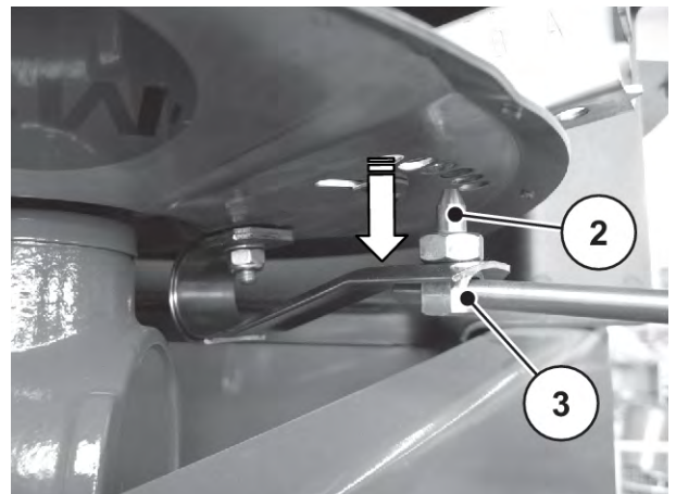
그림 45: 투척 블레이드 설정
