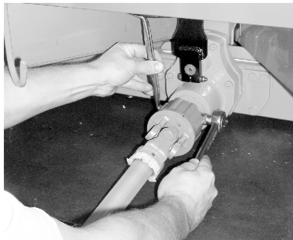
그림 21: 카르단 축 고정
