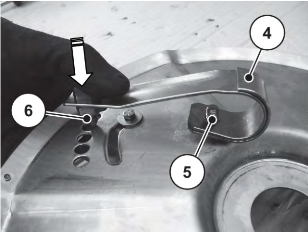
그림 91: 투척 디스크에 있는 판 스프링
