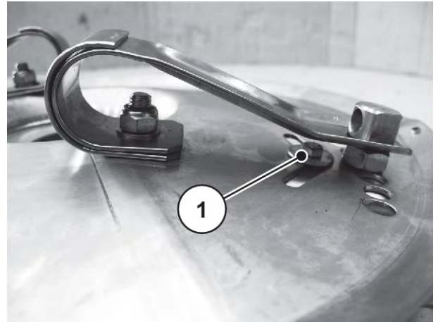
그림 78: 투척 디스크에 있는 판 스프링
