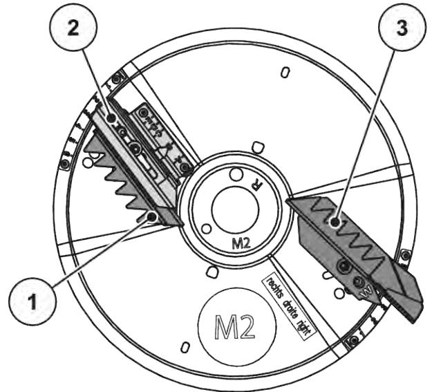
그림 93: 투척 디스크 M2
