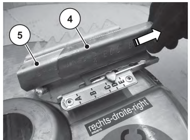
그림 80: 연장 블레이드와 메인 블레이드
