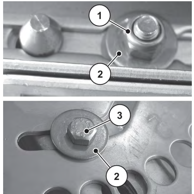
Рис. 90: Точки кріплення лопаті для розкидання
