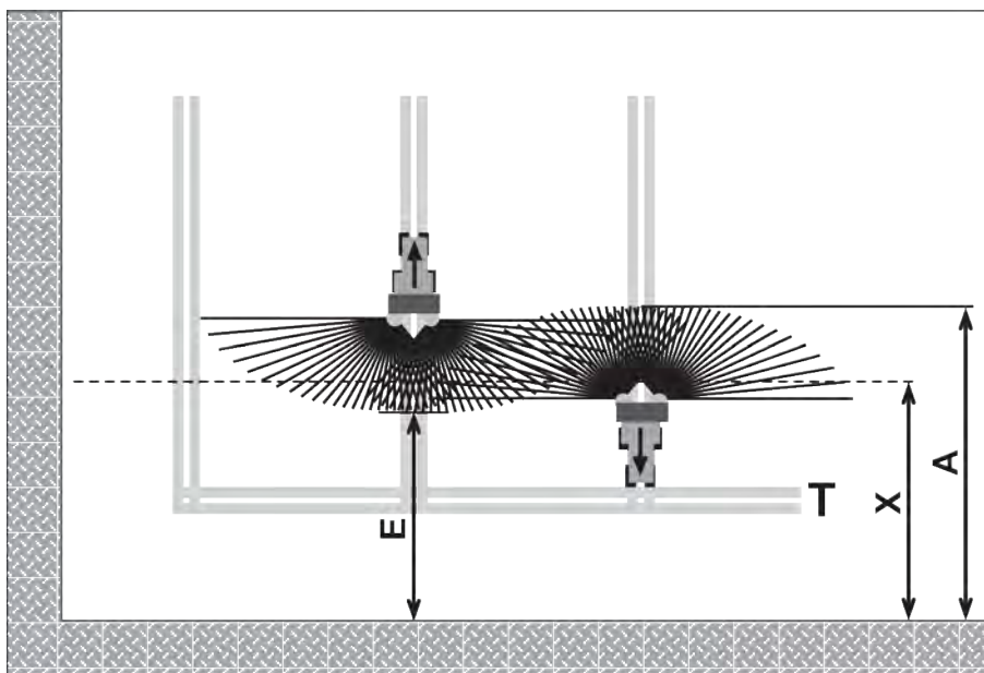
Рис. 56: Звичайне внесення добрива
