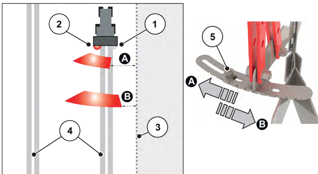
Рис. 52: Налаштування обмежувача ширини розкидання
