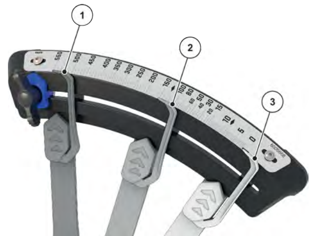
Рис. 31: Положення заслінки дозатора
