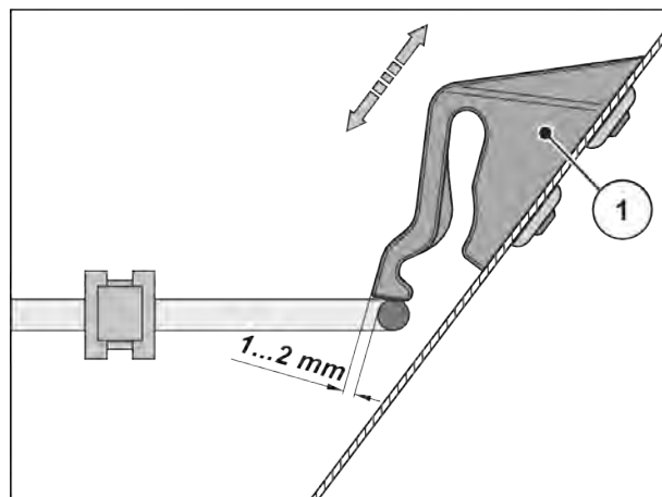
Рис. 65: Контрольний розмір для візуальної перевірки фіксатора захисної решітки
