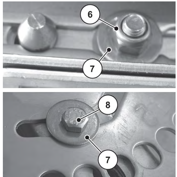
Рис. 82: Точки кріплення лопаті для розкидання
