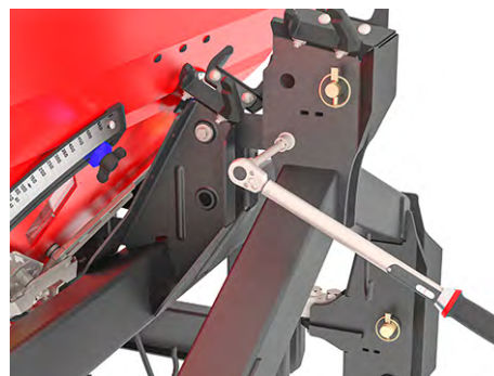
Рис. 62: Кріплення натяжної штанги на рамі ваг
