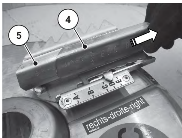
Рис. 80: Продовження лопаті й основна лопать
