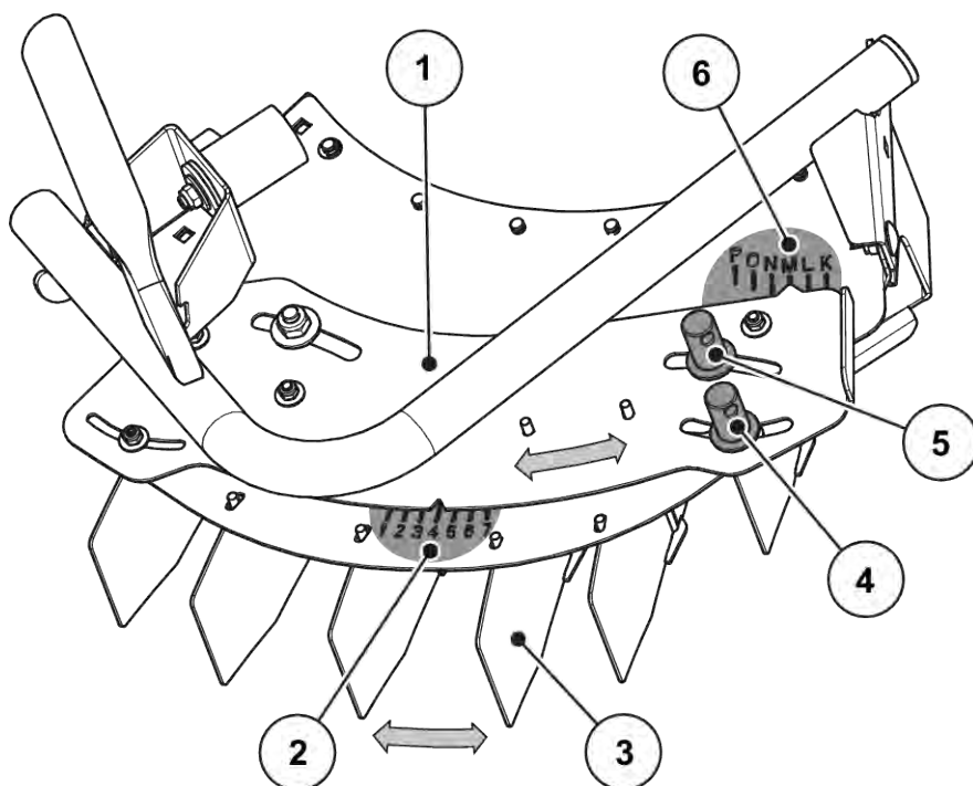
Рис. 53: Налаштування пристрою TELIMAT
