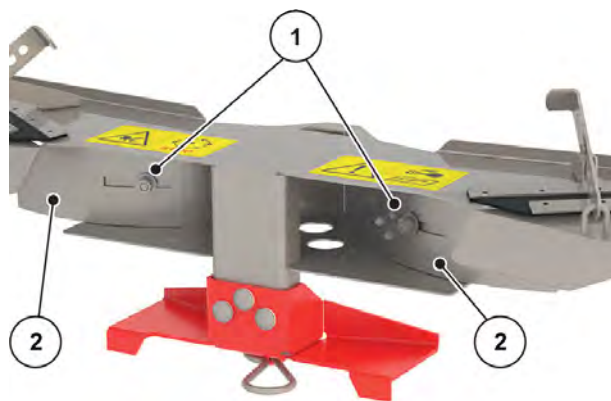
Рис. 58: Пластини рядкового пристрою для розкидання
