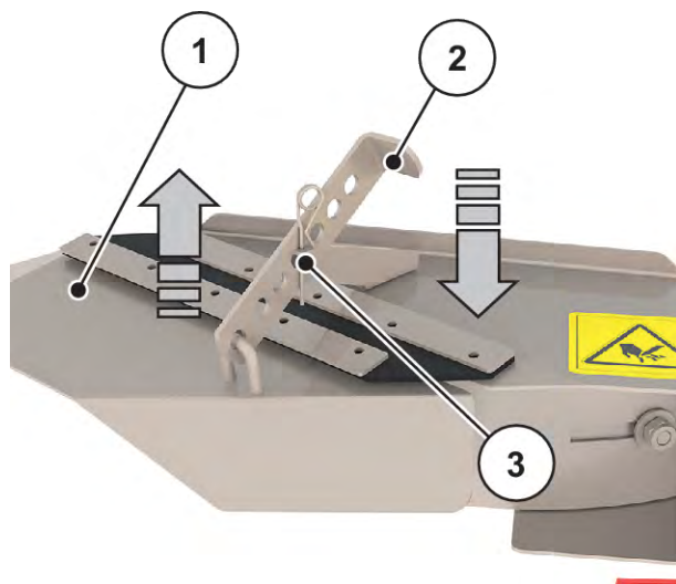
Рис. 59: Переміщення пластини на рядковому пристрої для розкидання
