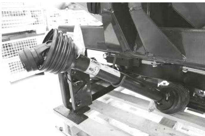
Рис. 60: Місце для зберігання карданного вала, місце для зберігання кабелів і шлангів гідравлічної системи
