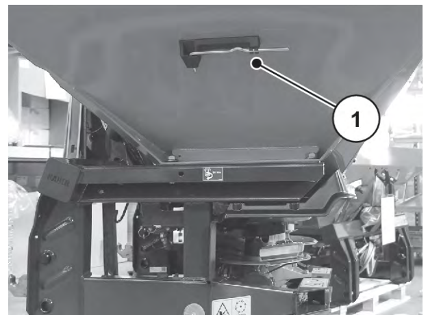
Рис. 10: Розташування регулювального важеля
