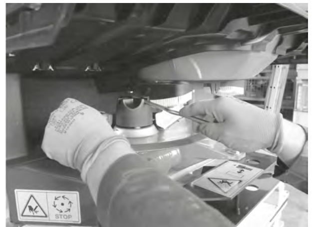
図 37: キャップナットをゆるめる
