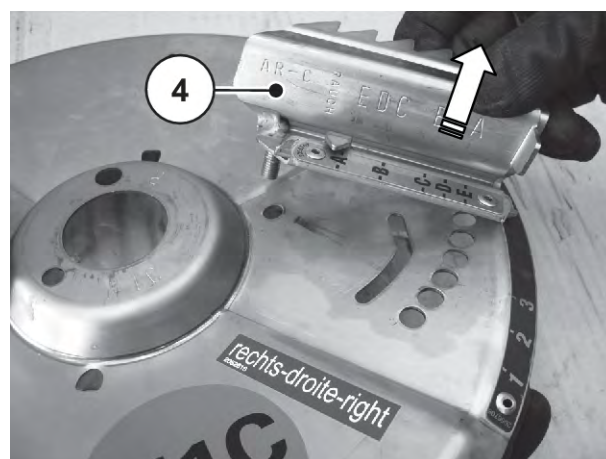
図 87: 散布ブレードを外す
