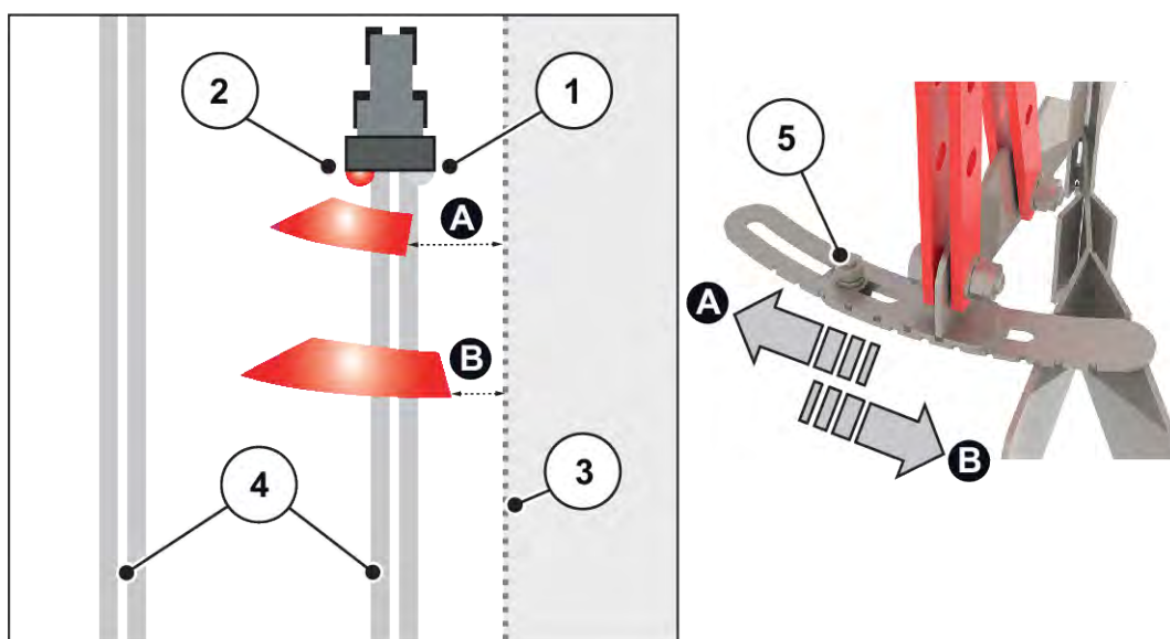
図 52: 境界散布システムの設定
