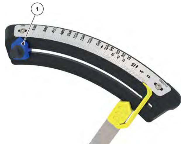
図 42: 散布量設定スケール(進行方向右側、Q タイプ)
