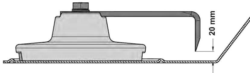
図 73: アジテーターフィンガーの磨耗範囲
