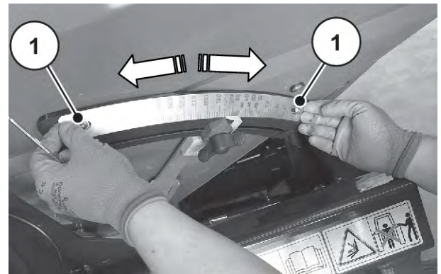
図 72: スケールをスライドさせる
