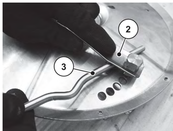
図 79: 板バネをロック解除する
