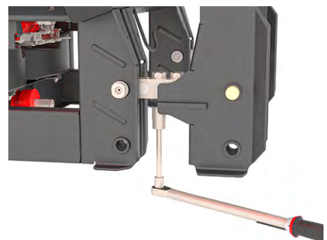
図 61: ロードセルの固定 (進行方向に向かって右側)
