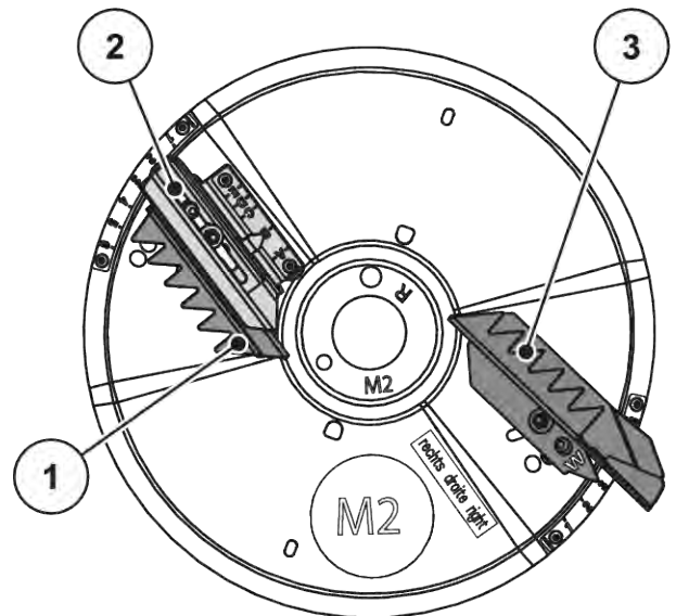
図 93: 散布ディスク M2
