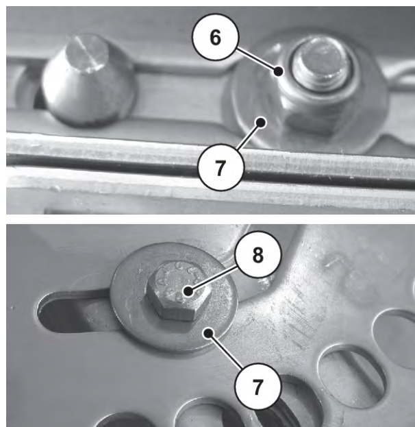
図 82: 散布ブレードの固定ポイント
