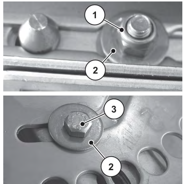
図 90: 散布ブレードの固定ポイント
