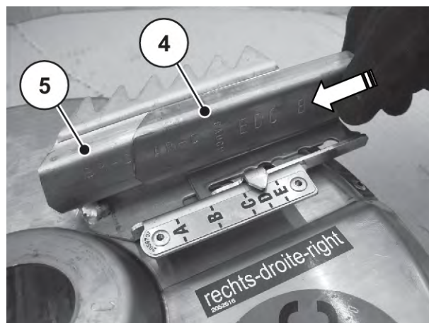
図 81: 新しいエクステンションブレード
