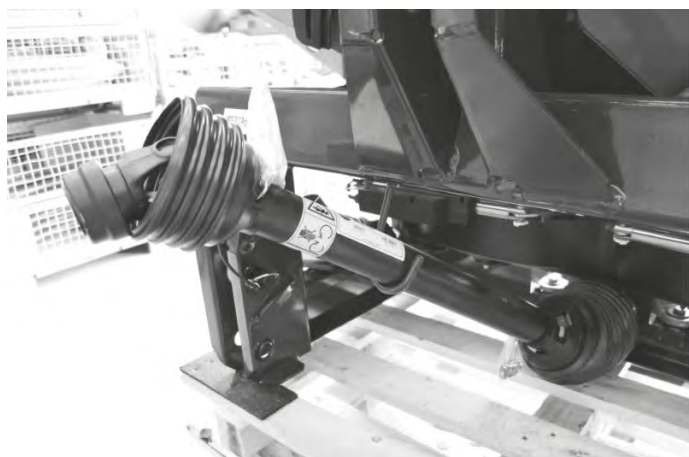
図 60: ジョイントシャフトの保管、ケーブルと油圧ホースの保管
