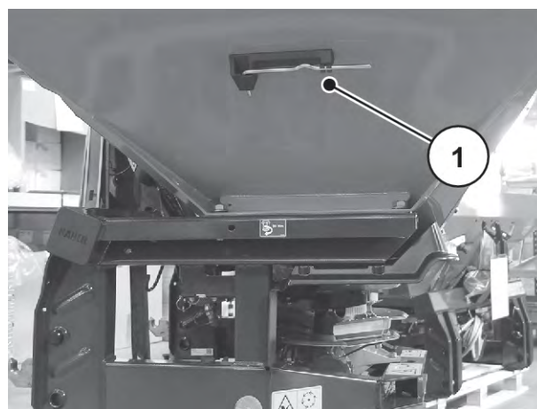
図 10: 調整レバーの位置
