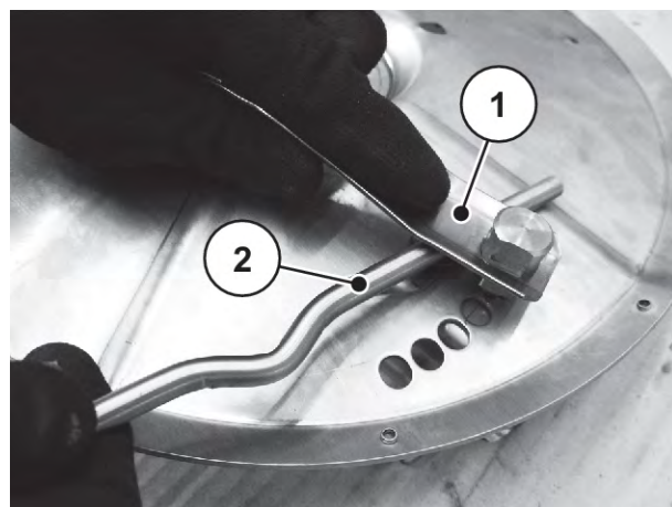
図 85: 板バネを外す
