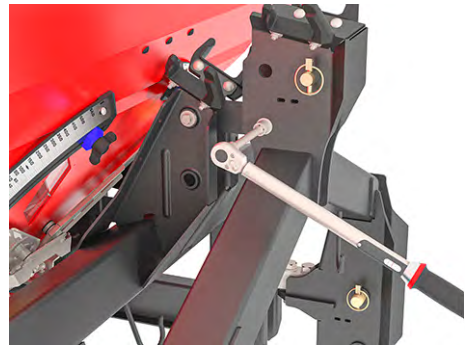
図 62: 重量計フレームのテンションロッドの固定
