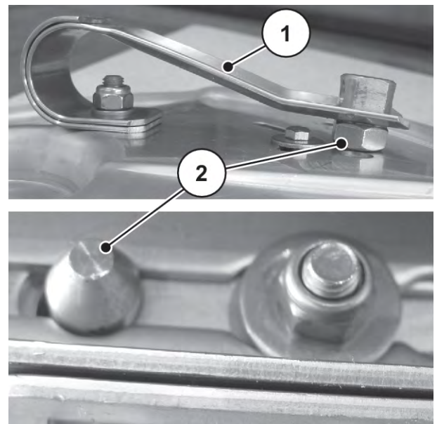
図 75: ロックピンが正しくはめ込まれた状態
