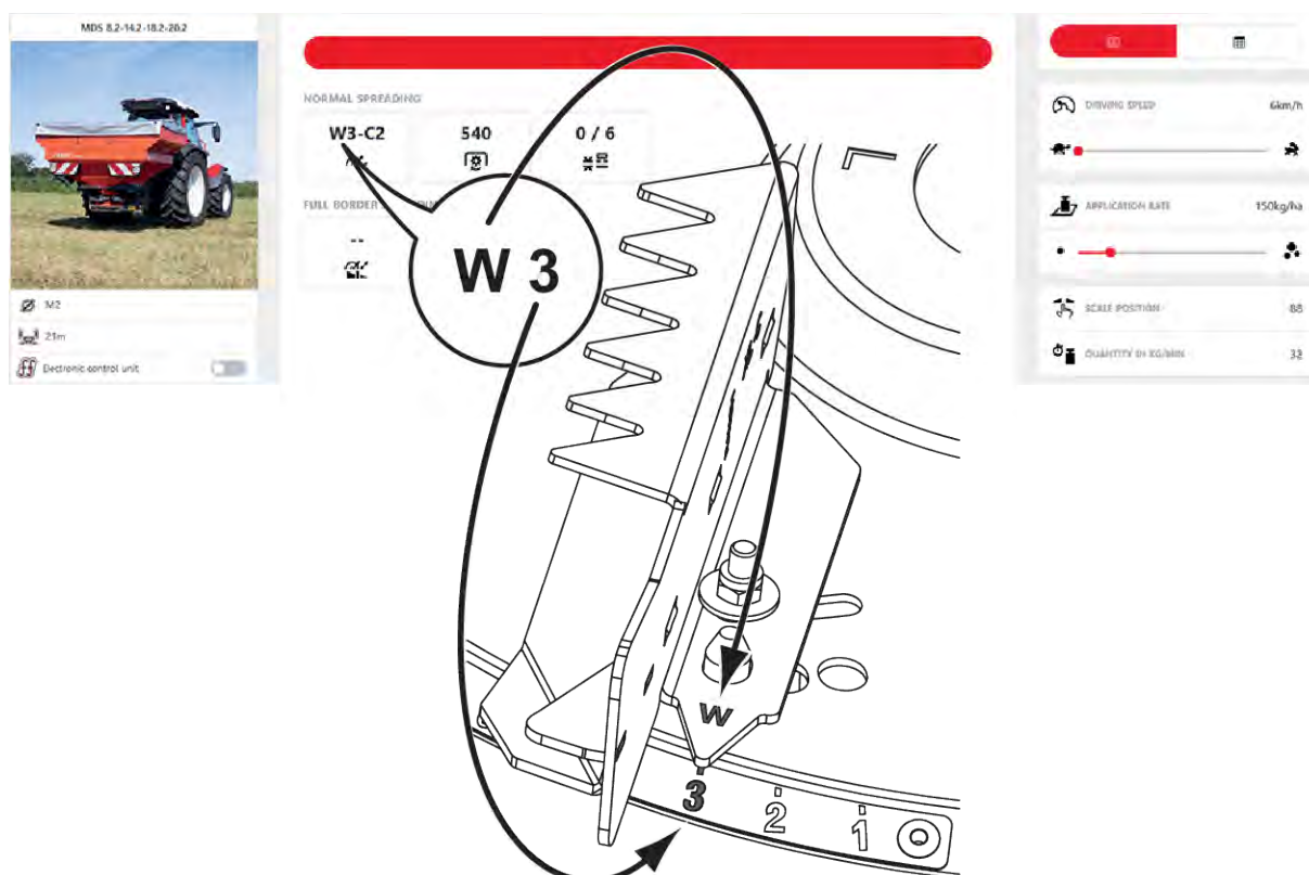
図 44: 散布ブレードの調節 散布ディスク M2、位置 W3、W: 固定長調節 1～6: 角度
