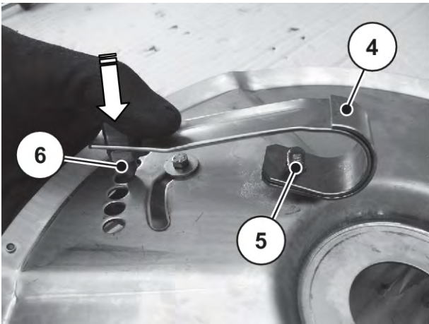
図 91: 散布ディスクの板バネ
