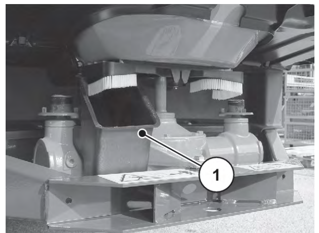
図 38: キャリブレーションテストシュートの取付け
