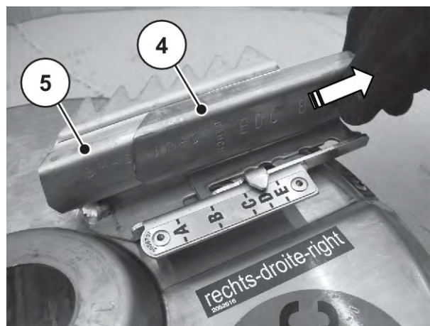
図 80: エクステンションブレードとメインブレード
