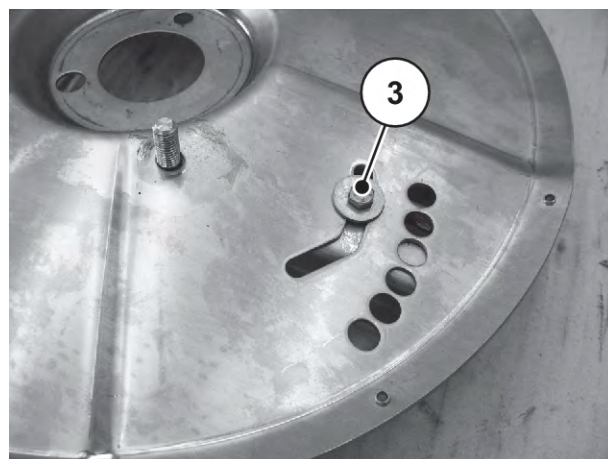
図 86: 散布ディスク下側のネジ
