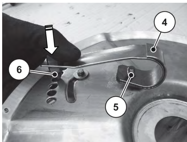
Obr. 91: Plochá pružina na rozmetávacom disku
