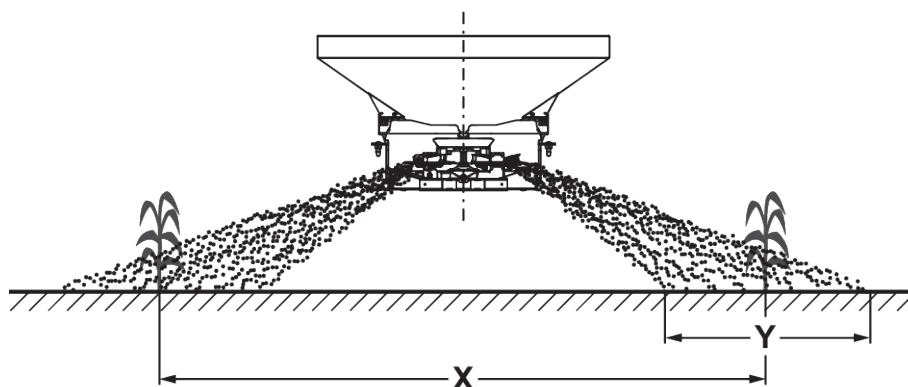
Obr. 57: Rozmetávanie s vybavením na radové rozmetávanie
