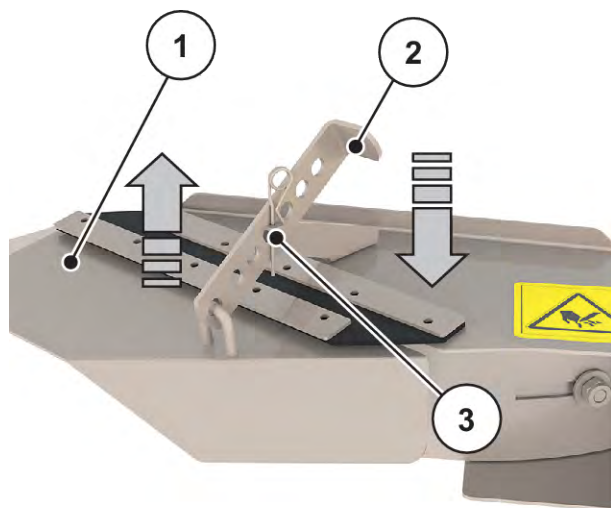
Obr. 59: Prestavenie na vybavenie na radové rozmetávanie
