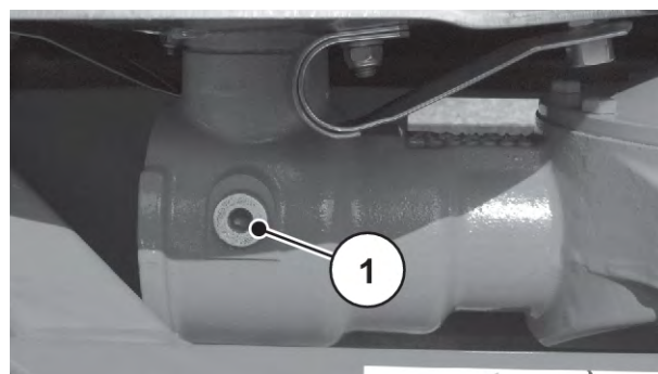
Obr. 93: Miesta pre napĺňanie a vypúšťanie prevodového oleja
