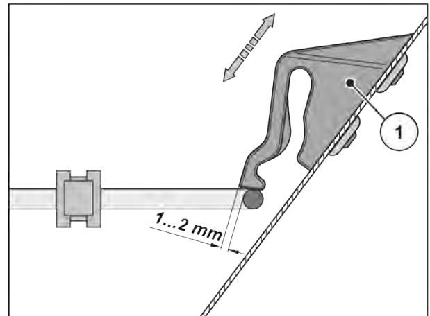
Obr. 65: Mierka na kontrolu funkčnosti zablokovania ochrannej mreže
