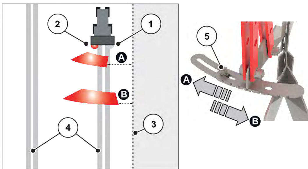
Obr. 52: Nastavenie zariadenia na hraničné rozmetávanie
