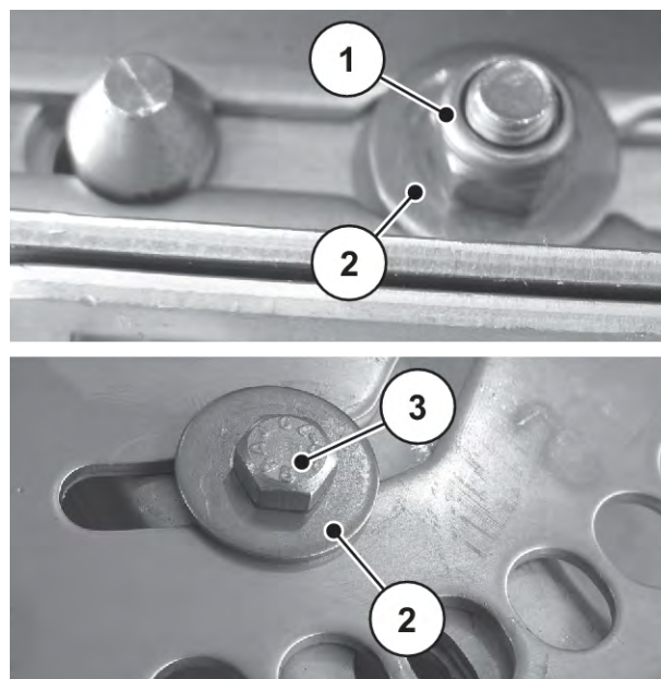
Obr. 90: Upevňovacie body rozmetávacích lopatiek
