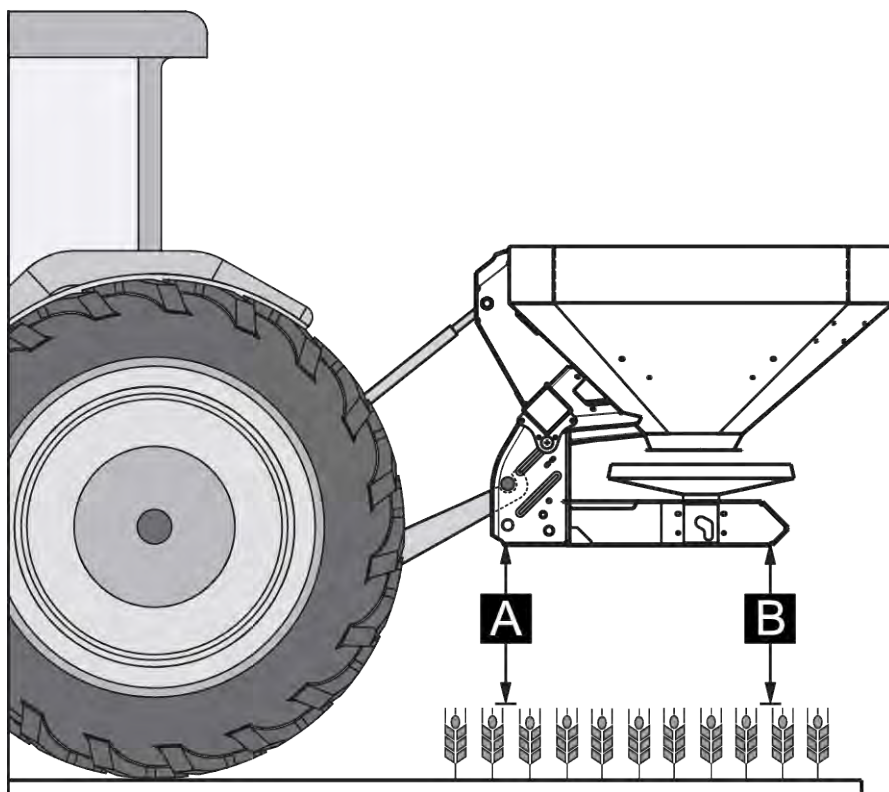
Obr. 24: Montážna poloha
