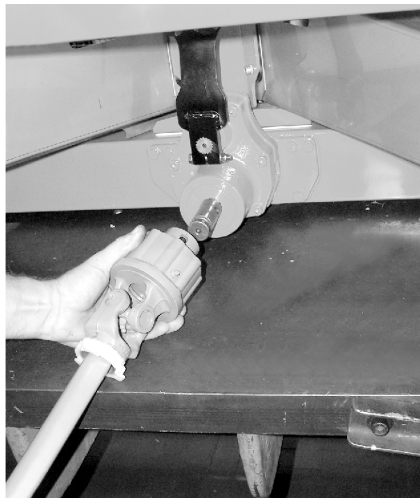
Obr. 20: Nasadenie klbového hriadeľa na výstupný hriadeľ prevodovky
