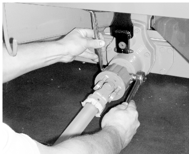
Obr. 21: Upevnenie klbového hriadeľa
