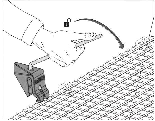
Şek. 64: Koruyucu ızgara kilidini açın
