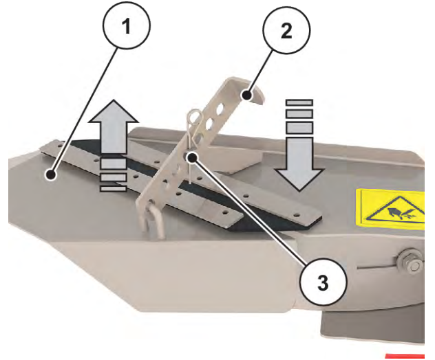
Şek. 59: Sıra serpme tertibatının ayarı
