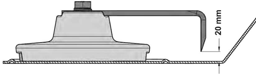
Şek. 73: Karıştırma parmağının aşınma alanı
