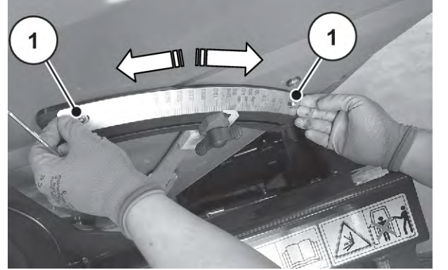
Şek. 72: Skalanın kaydırılması
