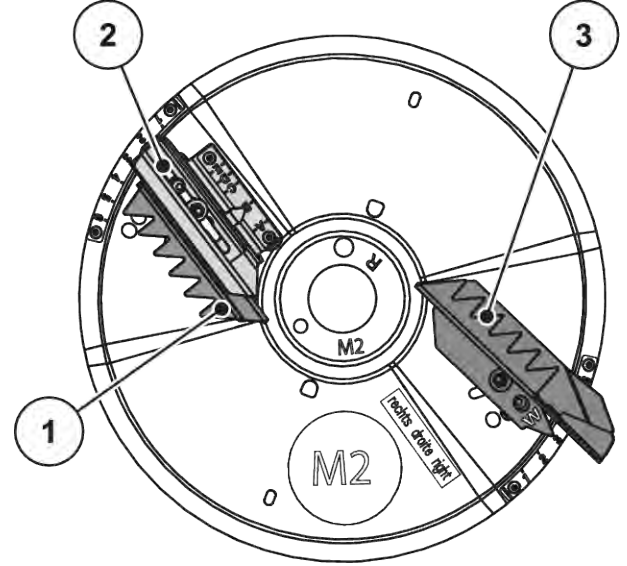
Şek. 93: M2 fırlatma diski
