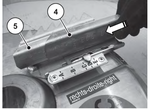
Şek. 81: Yeni uzatma kanadı
