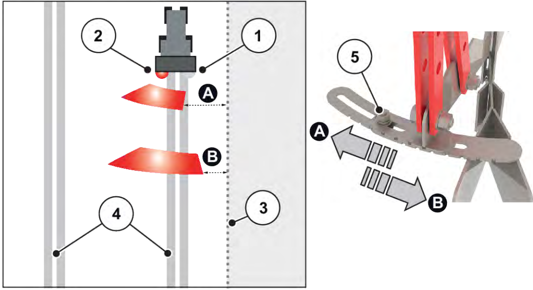
Şek. 52: Sınır serpme tertibatının ayarı
