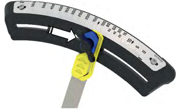
Şek. 71: Sınırlayıcının kaydırılması
