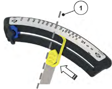
Şek. 70: Konum göstergesinin kaydırılması
