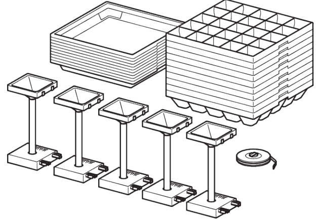
Şek. 12: PPS5 opsiyonel donanım
