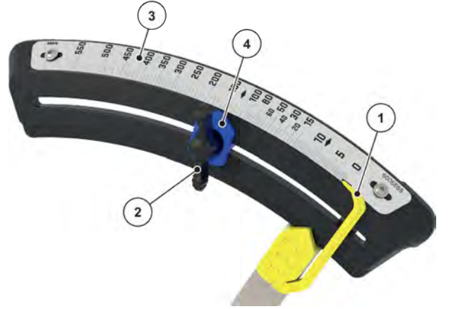
Şek. 41: Uygulama miktarını ayarlamaya yönelik skala (sürüş yönüne göre sağda, K/D/C varyantları)
