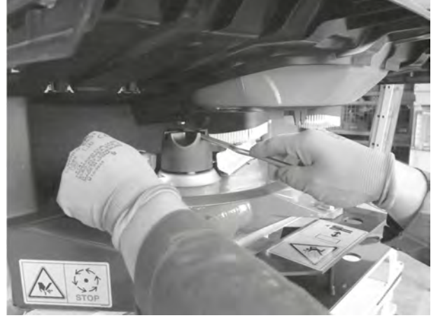
Şek. 74: Başlıklı somunu gevşetin
