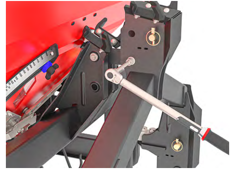
Şek. 62: Gergi çubuğunun tartılı çatkıya sabitlenmesi
