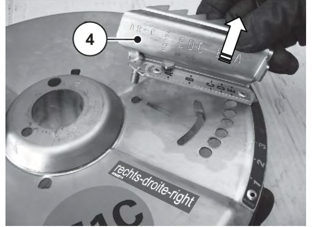
Şek. 87: Fırlatma kanadının çıkarılması
