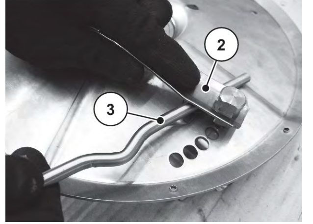
Şek. 79: Yassı yayın yerinden çıkarılması
