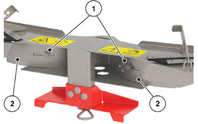
Şek. 58: Sıra serpme tertibatı üzerindeki levhalar
