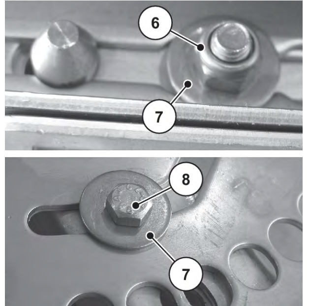
Şek. 82: Fırlatma kanadının sabitleme noktaları
