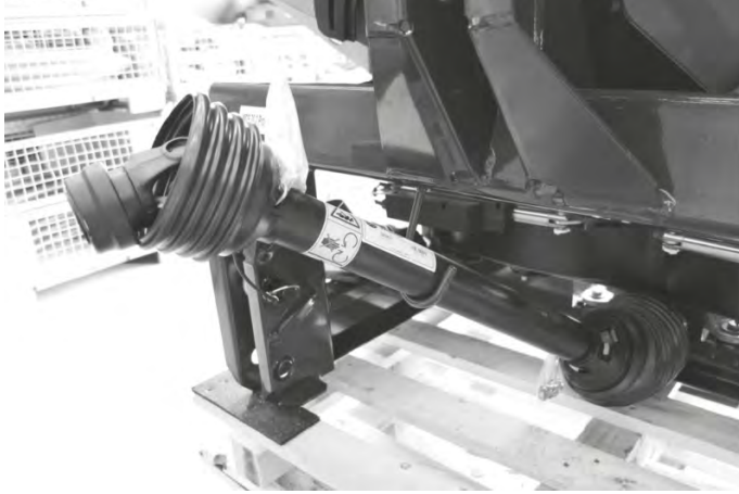
Şek. 60: Tahrik milinin depolanması, kabloların ve hidrolik hortumların depolanması
