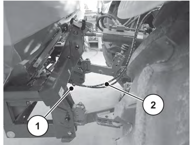
Şek. 25: Hidrolik hortumlarının döşenmesi
