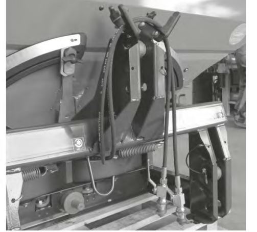
Şek. 60: Tahrik milinin depolanması, kabloların ve hidrolik hortumların depolanması
