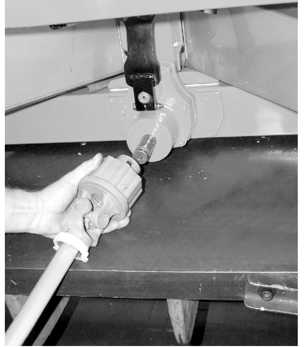
Şek. 20: Tahrik milini şanzıman miline monte edin
