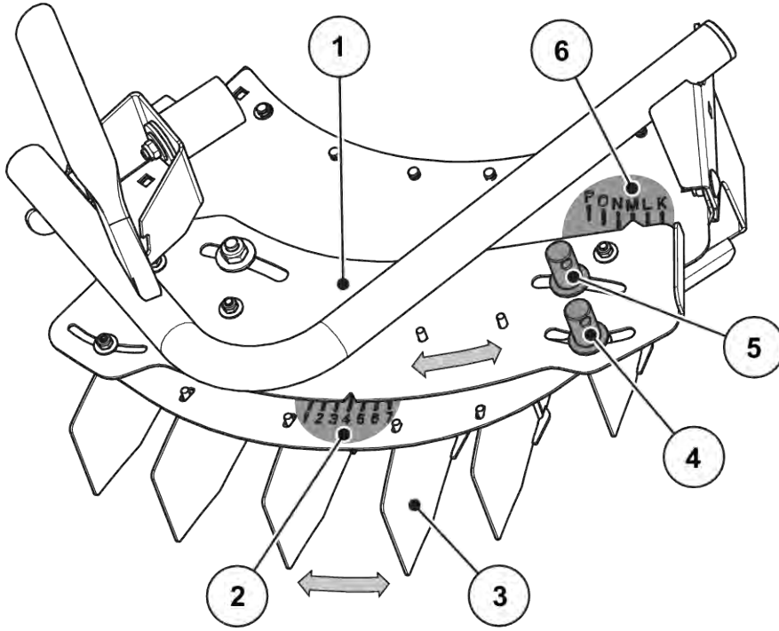
Şek. 53: TELIMAT tertibatının ayarı
