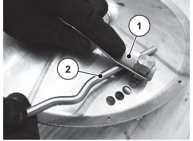
Şek. 85: Yassı yayın çıkarılması
