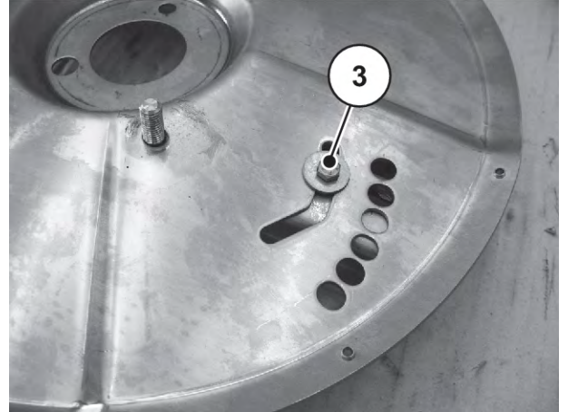
Şek. 86: Fırlatma diski alt tarafındaki cıvata
