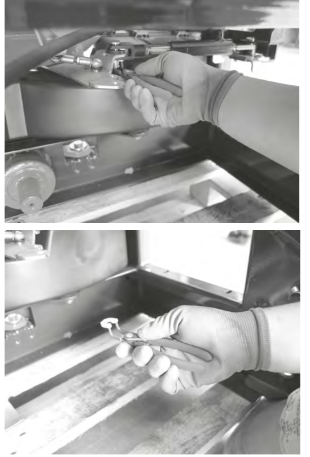
Şek. 68: Silindiri çıkarın.
