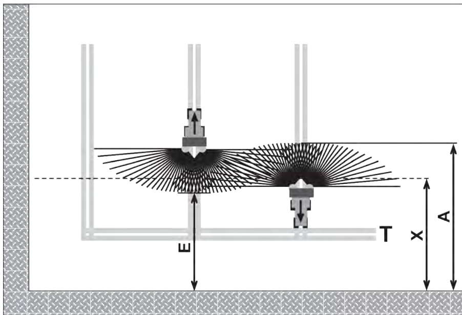
Ábr. 56: Normál szórás
