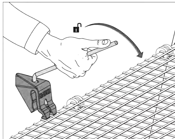
Ábr. 64: Védőrács-reteszelés kinyitása
