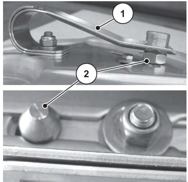
Ábr. 75: A reteszelőcsap megfelelően rögzítve
