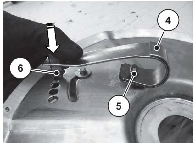
Ábr. 91: Laprugó a szórótárcsán
