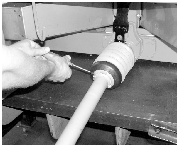
Ábr. 23: A kardántengely-védelem rögzítése
