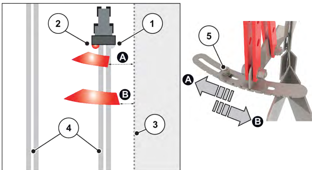
Ábr. 52: A határszóró berendezés beállítása
