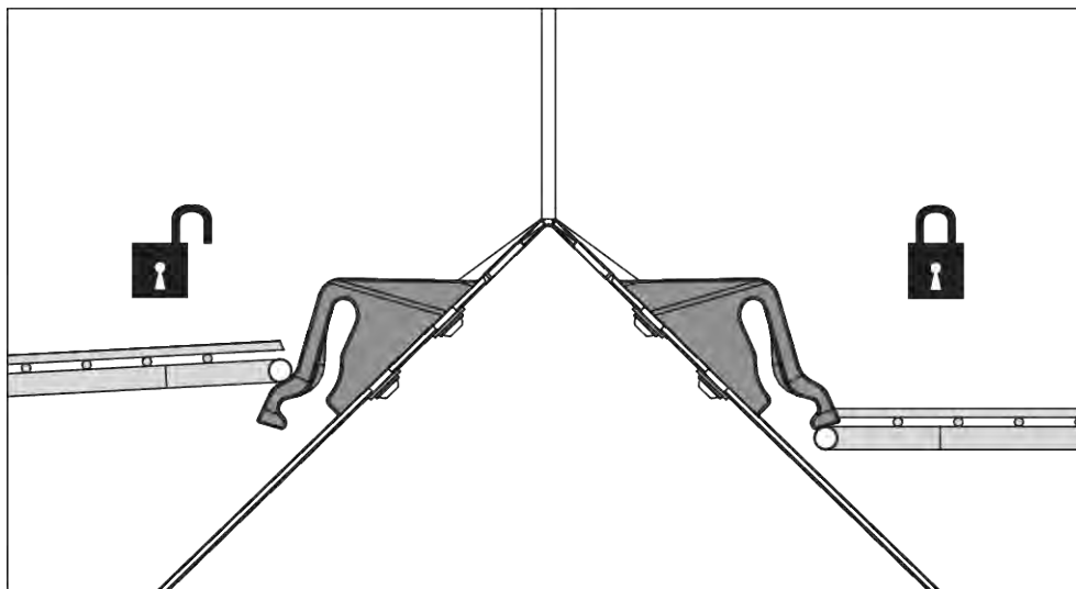
Ábr. 63: Védőrács-reteszelés nyitva/zárva
