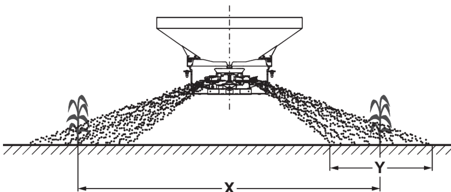
Ábr. 57: Szórás sorszóró berendezéssel
