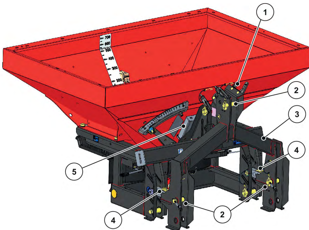
Ábr. 8: Részegységek áttekintése: MDS elülső oldala ISOBUS-szal és mérőkerettel
