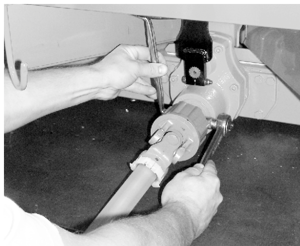
Ábr. 21: Kardántengely rögzítése
