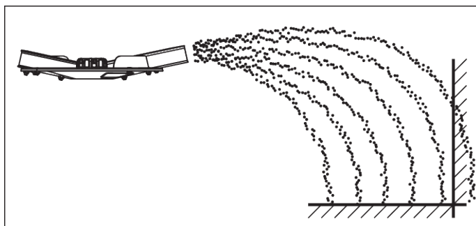
Ábr. 47: Szegélyszórás normál trágyázás esetén
