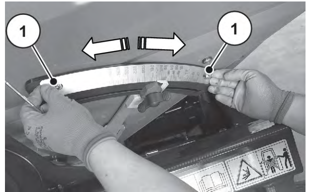
Ábr. 72: Skála eltolása
