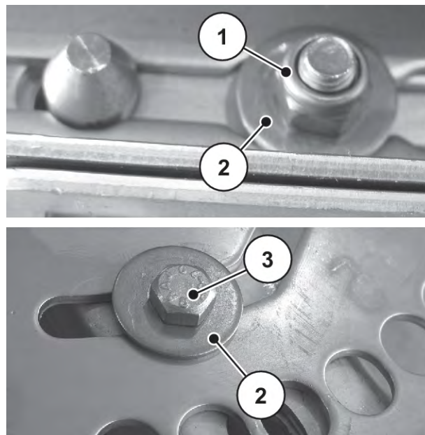
Ábr. 90: Szórólapátok rögzítési pontjai
