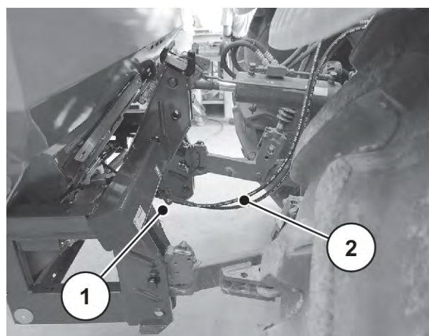
Ábr. 25: Hidraulikatömlők vezetése
