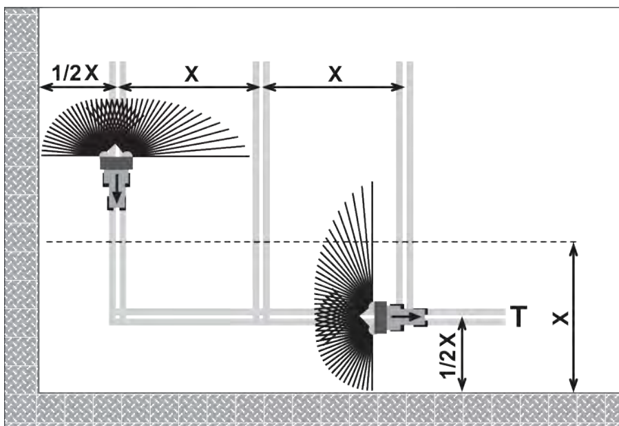
Ábr. 55: Határszórás
