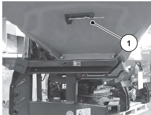
Sl. 10: Položaj poluge za podešavanje
