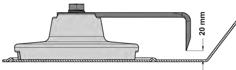
Sl. 73: Područje istrošenosti mešalice
