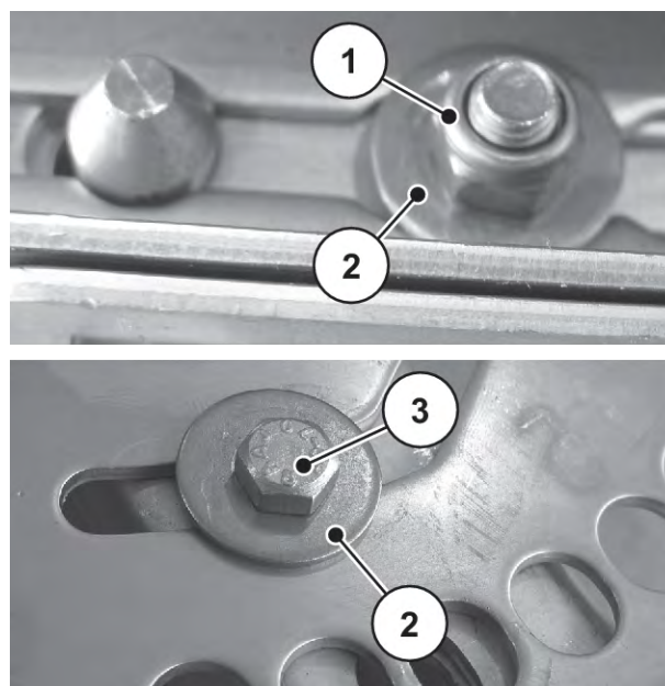
Sl. 90: Pričvrstne tačke lopatica za rasipanje
