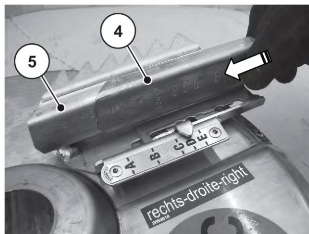
Sl. 81: Nova produžna lopatica
