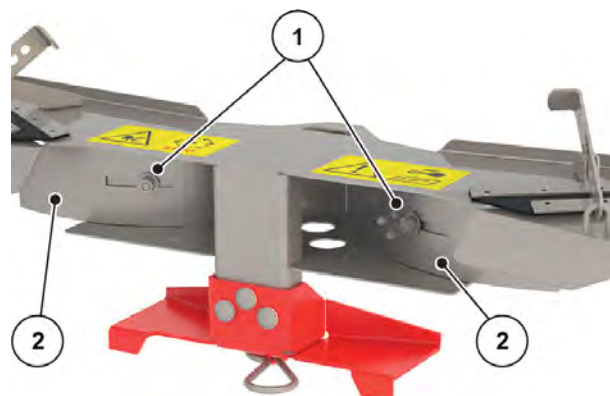
Sl. 58: Limovi na mehanizmu za rasipanje po redovima
