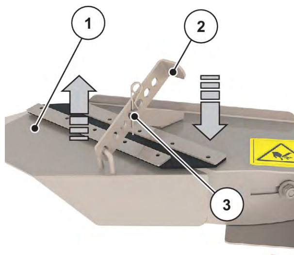
Sl. 59: Podešavanje na mehanizmu za rasipanje po redovima
