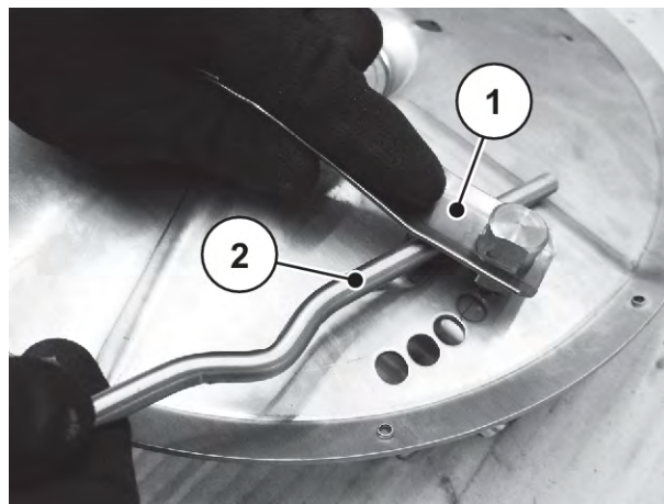
Sl. 85: Uklanjanje ravne opruge
