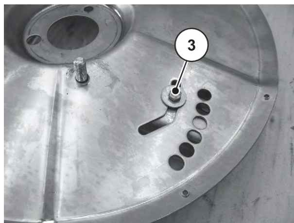
Sl. 86: Zavrtnj na donjoj strani diska za rasipanje
