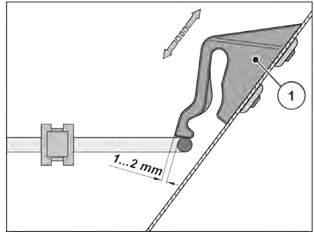
Sl. 65: Kontrolno merilo za proveru funkcionalnosti blokade zaštitne rešetke
