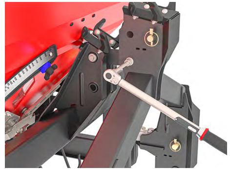
Sl. 62: Pričvrščivanje vučne šipke na okvir za vaganje
