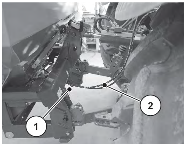
Kuva 25: Hydrauliletkujen reititys
