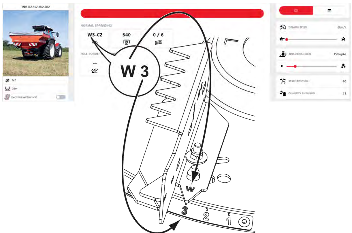
Kuva 44: Levityssiiven asetus levityslautanen M2, asento W3: kiinteä pituusasetus 1–6. Kulma-asetus
