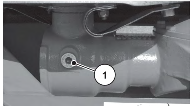
Kuva 94: Vaihteistoöljyn täyttö- ja tyhjennyskohdat
