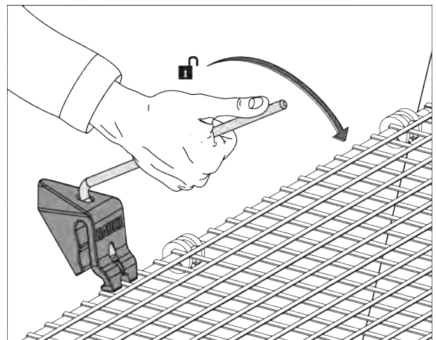
Kuva 64: Suojaristikon lukituksen avaaminen
