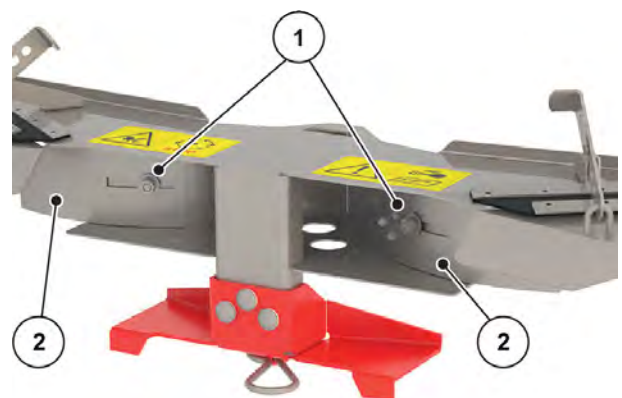
Kuva 58: Levyt rivilevityslaitteessa
