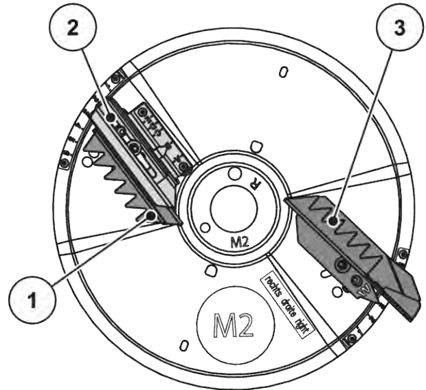
Kuva 93: Levityslautanen M2
