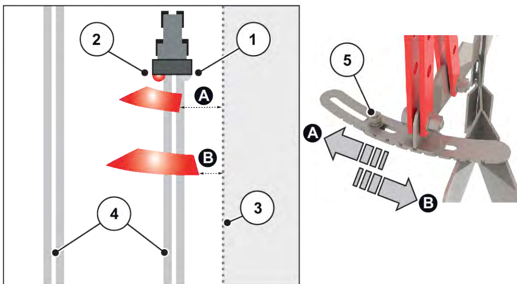
Kuva 52: Rajalevityslaitteen asetus
