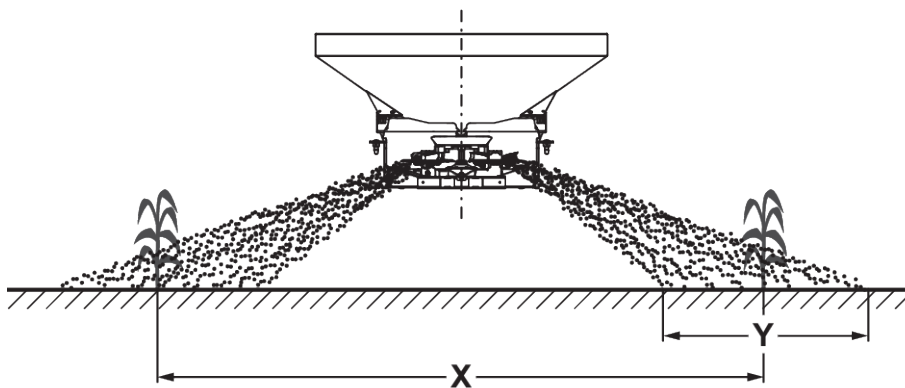
Kuva 57: Levitys rivilevityslaitteella
