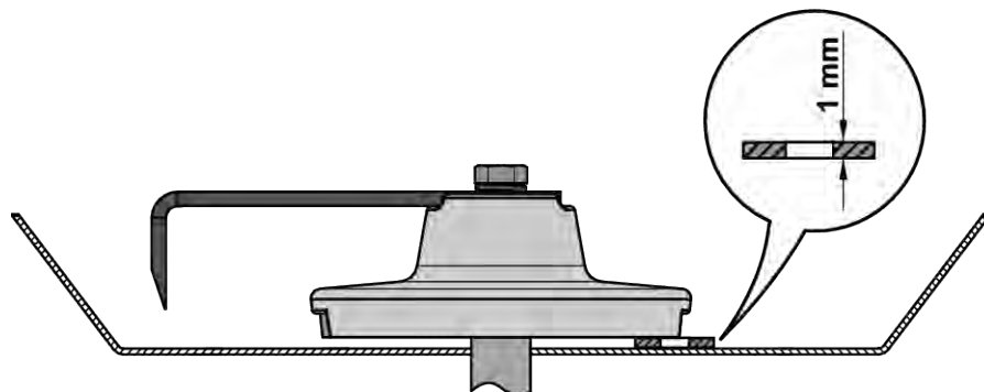
Kuva 76: Sekoittimen asetusten säätö
