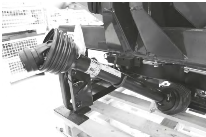
Kuva 60: Nivelakselien, johtojen ja hydrauliletkujen säilytys
