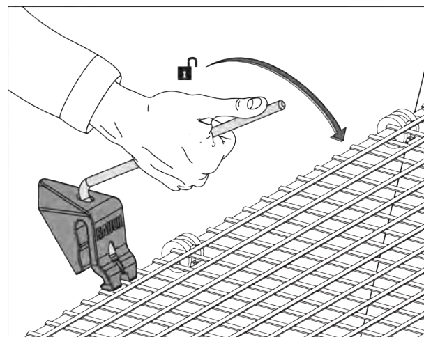
Fig. 64: Öppna skyddsgallerlåsningen
