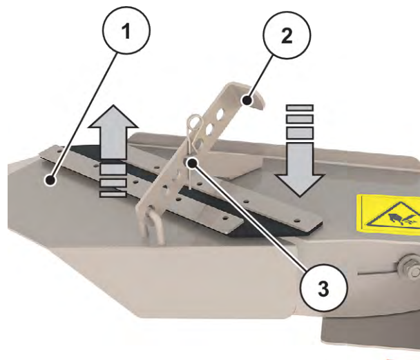
Fig. 59: Justering på radspridningsutrustningen
