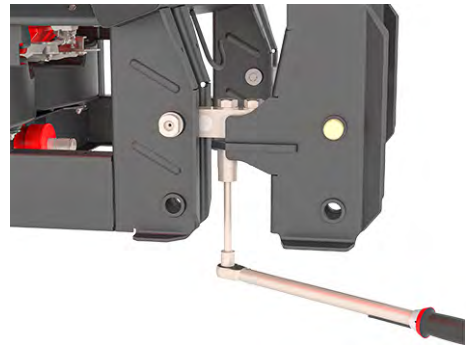
Fig. 61: Lastcellens fastsättning (i körriktning höger)
