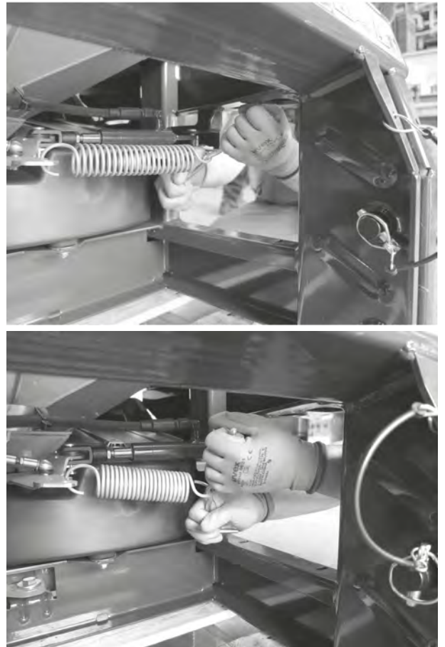
Fig. 67: Haka ur fjädern
