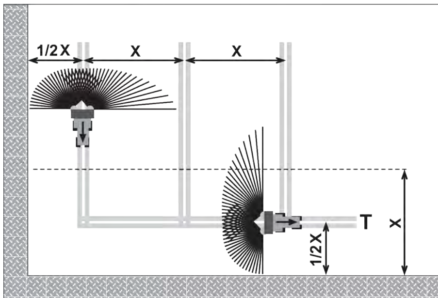
Fig. 55: Gränsspridning
