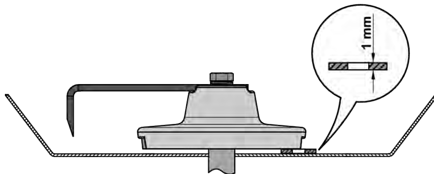
Fig. 76: Innstilling av røreverket
