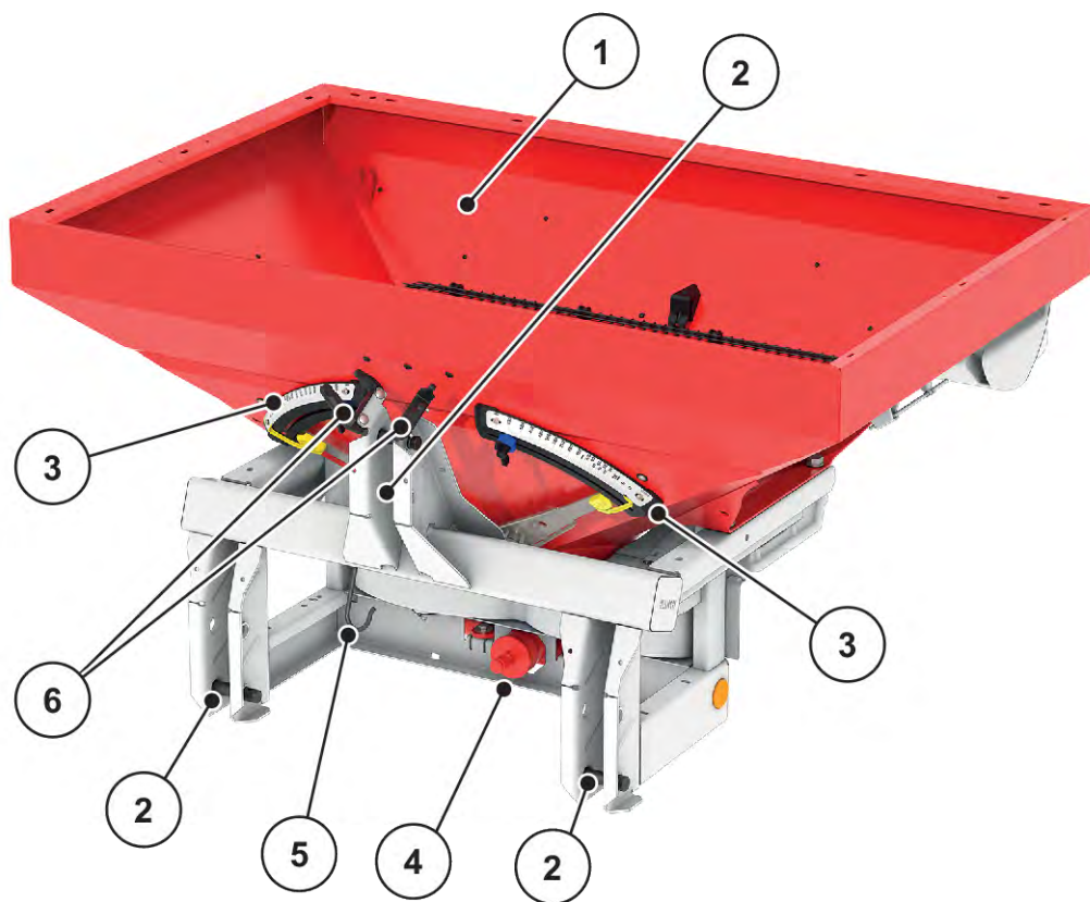
Fig. 5: Komponentoversikt: Forside
