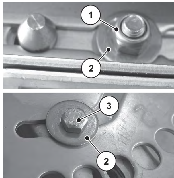
Fig. 90: Festepunktene til spredevingene
