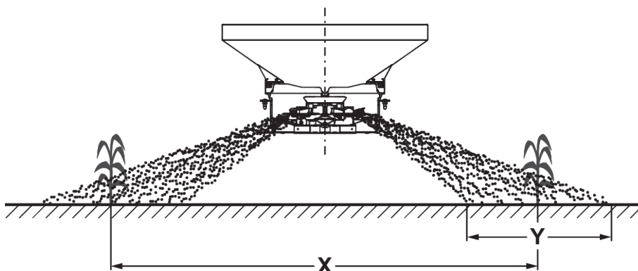
Fig. 57: Spredning med radespredningsenhet
