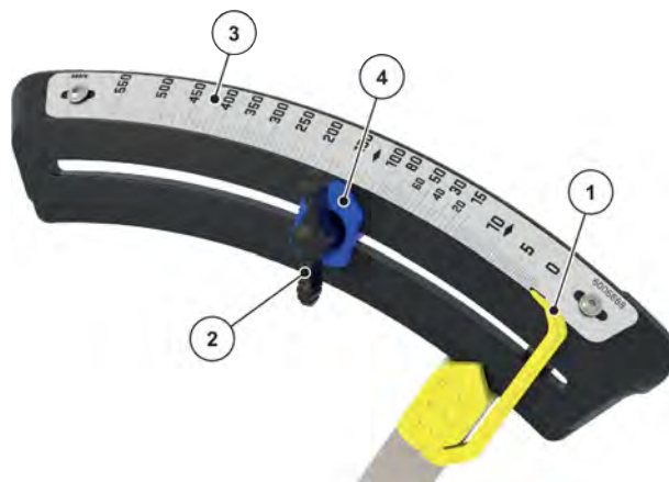
Fig. 41: Skala for å stille inn spredemengden (høyre kjøreretning, variantene K/D/C)
