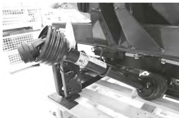
Fig. 18: Kardangakselholder
