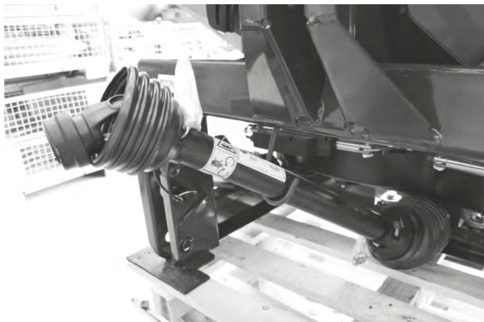
Sl. 60: Nosilec za kardansko gred, nosilec za kabel in hidravlične cevi
