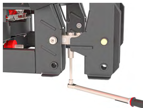
Sl. 61: Pritrditev tehtalnih celic (v smeri vožnje desno)
