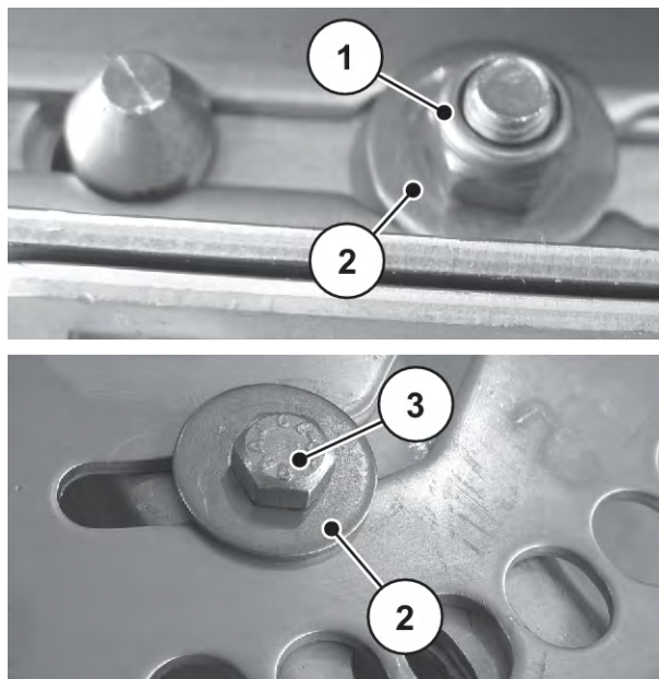
Sl. 90: Pritrdilne točke trosilne lopatice
