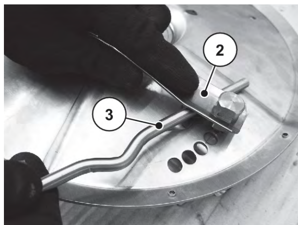
Sl. 79: Izskočite ploščato vzmet.
