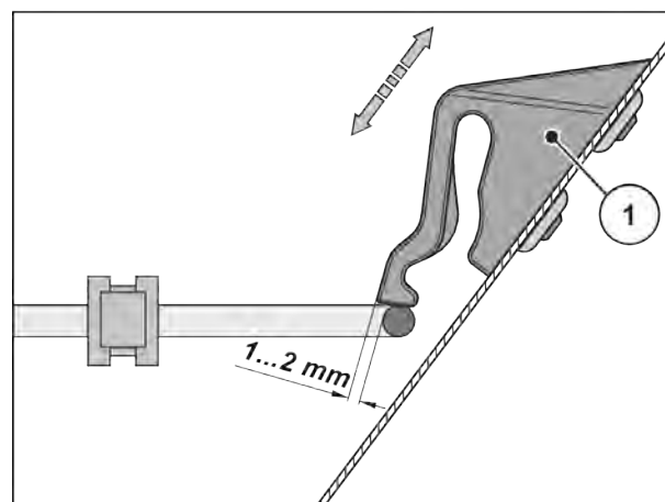
Sl. 65: Mera za preverjanje delovanja zapaha zaščitne mreže
