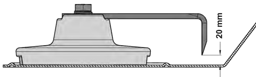
Sl. 73: Obrabljeno območje mešalnega količka
