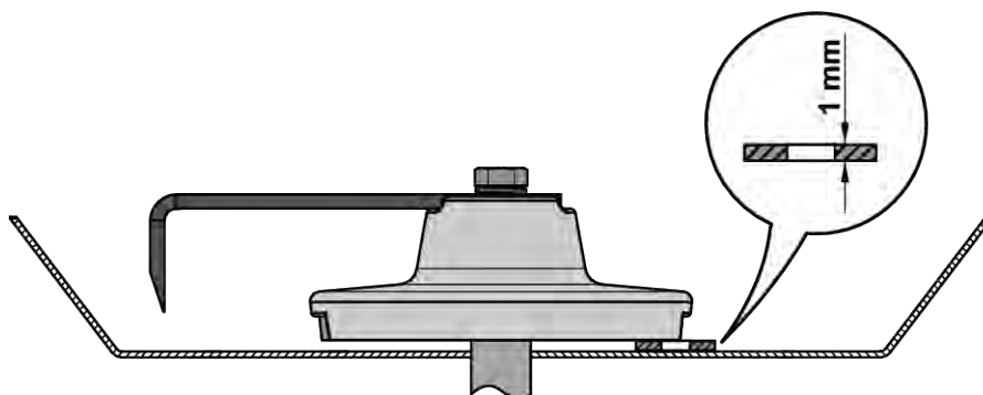
Sl. 76: Namještanje miješalice
