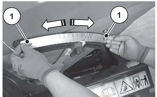
Sl. 72: Pomicanje ljestvice
