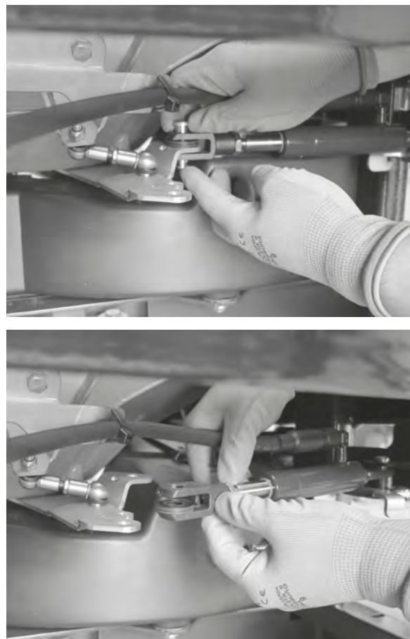
Sl. 69: Izvlačenje hidrauličnog cilindra
