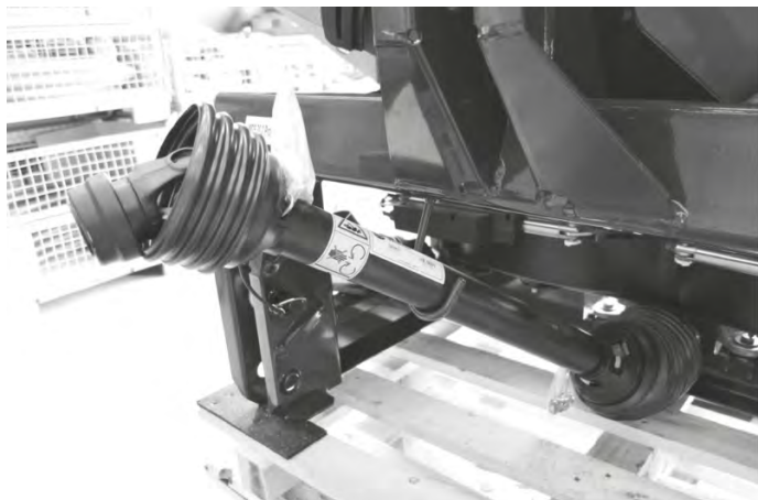
Sl. 60: Mjesto za odlaganje kardanskog vratila, mjesto za odlaganje kabela i hidrauličnih crijeva
