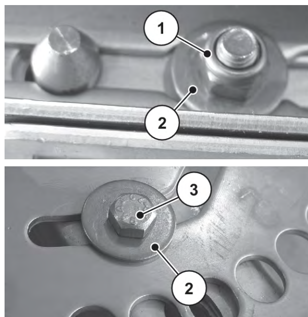
Sl. 90: Pričvrstne točke lopatica za rasipanje
