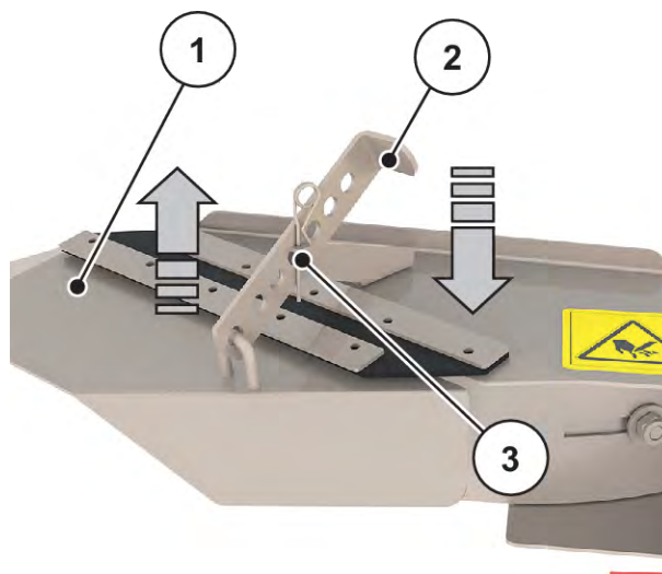
Sl. 59: Namještanje naprave za rasipanje po redovima
