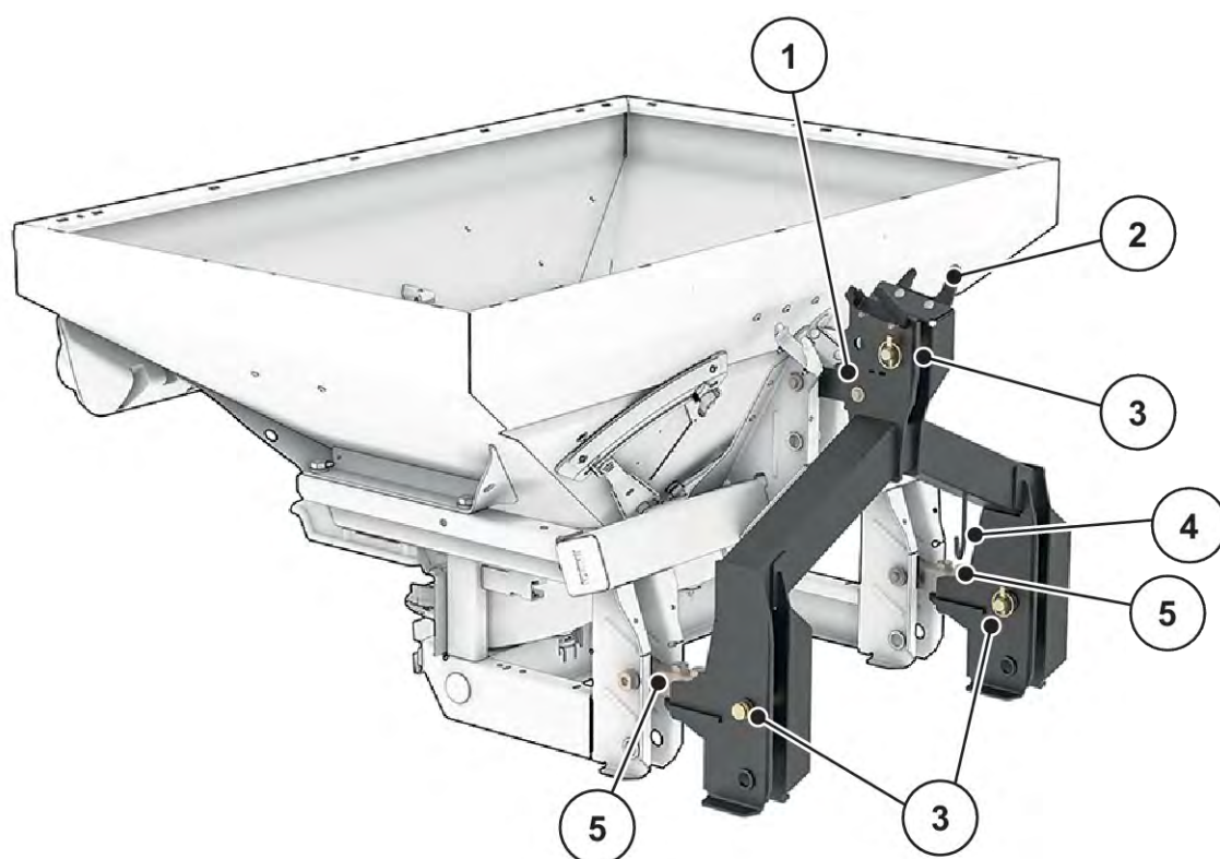
Fig. 6: Prezentare generală a subansamblurilor: Parte anterioară cu cadru de cântărire
