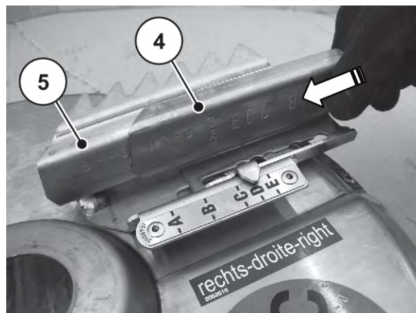
Fig. 81: Aripa de prelungire nouă
