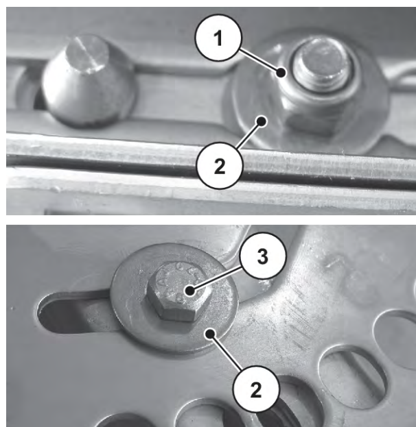
Fig. 90: Punctele de fixare ale aripilor aruncătoare
