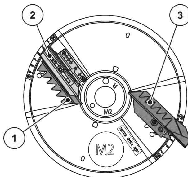
Fig. 93: Disc aruncător M2
