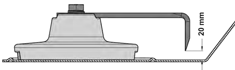
Fig. 73: Zona de uzură a paletelor colțar de amestecare
