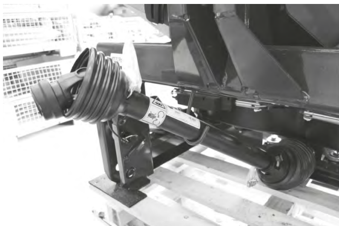
Fig. 60: Așezarea arborelui cardanic, cablurilor și a furtunurilor hidraulice
