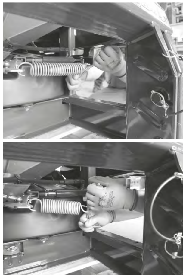
Fig. 67: Suspendarea arcului
