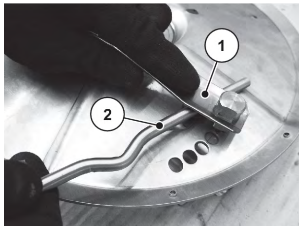
Fig. 85: Scoaterea arcului plat
