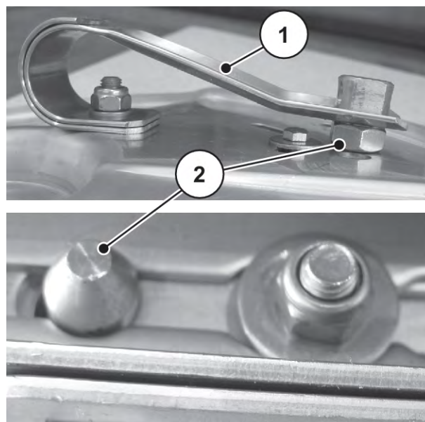
Fig. 75: Bolțul de blocare este fixat corect
