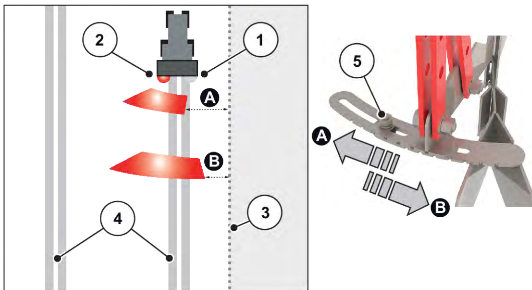
Fig. 52: Reglarea dispozitivului de împrăștiere la limită
