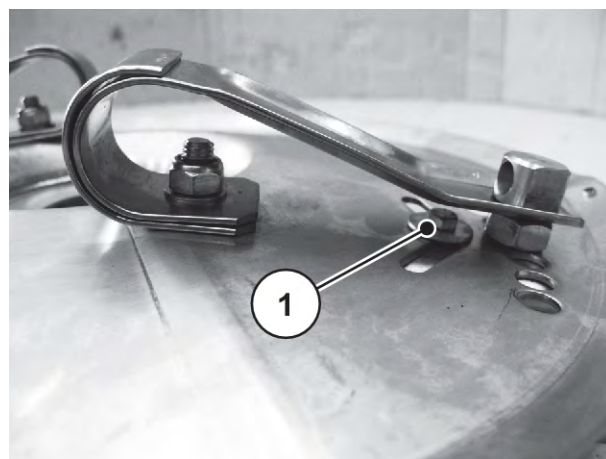
Fig. 78: Arc plat de la discul aruncător
