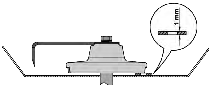
Ilust. 76: Ajuste do agitador
