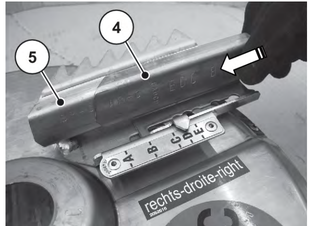
Ilust. 81: Nova hélice de extensão
