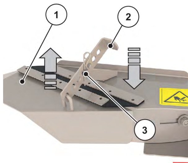
Ilust. 59: Ajuste no dispositivo de dispersão em linhas
