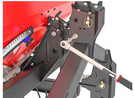
Ilust. 62: Fixação da barra de tração na estrutura de pesagem
