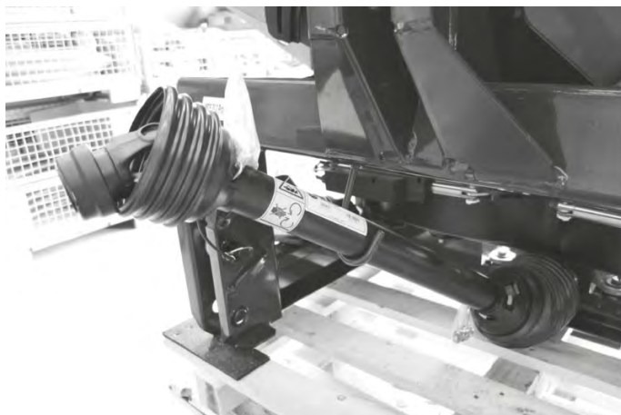
Ilust. 60: Apoio do eixo articulado, apoio dos cabos e mangueiras hidráulicas
