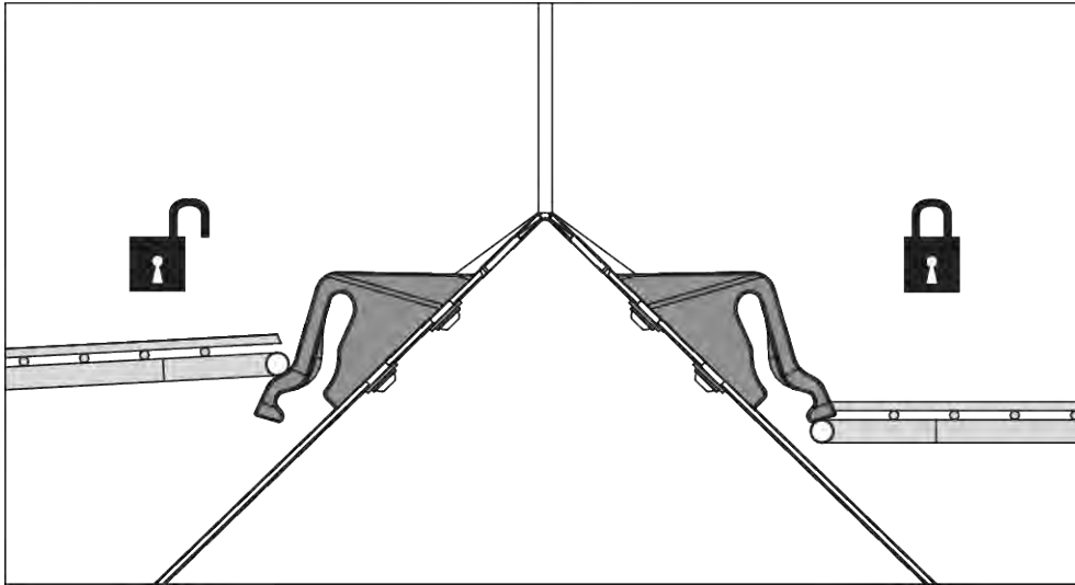
Ilust. 63: Bloqueio das grades de proteção aberto/fechado
