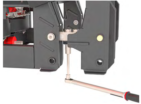
Ilust. 61: Fixação da célula de pesagem (em direção do trajeto à direita)
