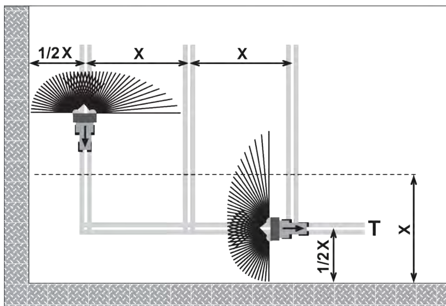
Ilust. 55: Dispersão limite
