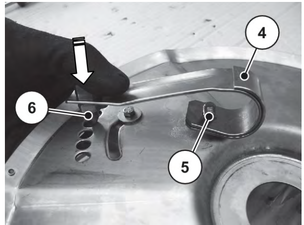
Ilust. 91: Mola plana no disco dispersor
