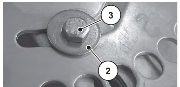
Ilust. 90: Pontos de fixação da hélice de dispersão
