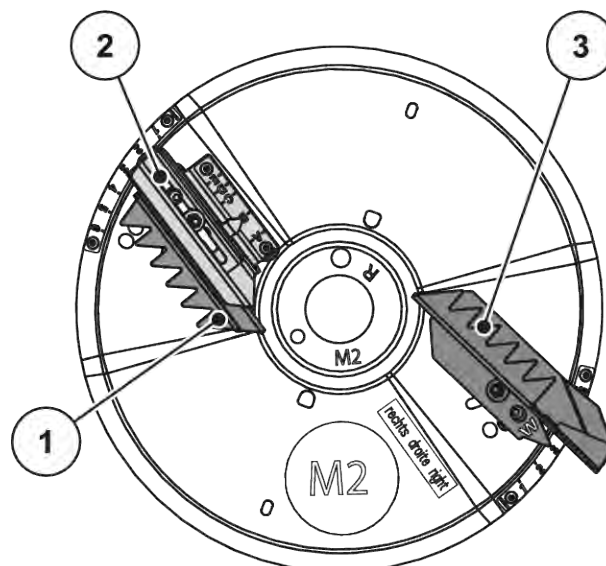
Ilust. 93: Disco dispersor M2
