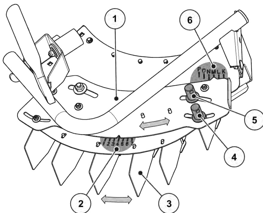
Rys. 53: TELIMAT Ustawianie urządzenia
