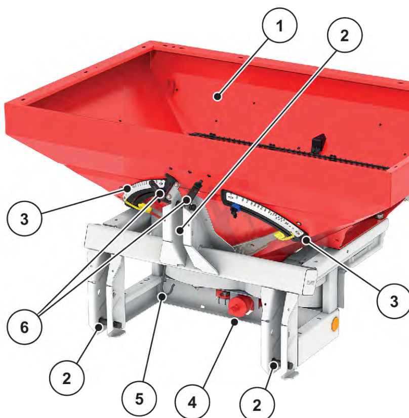
Rys. 5: Widok ogólny zespołów: Widok od przodu
