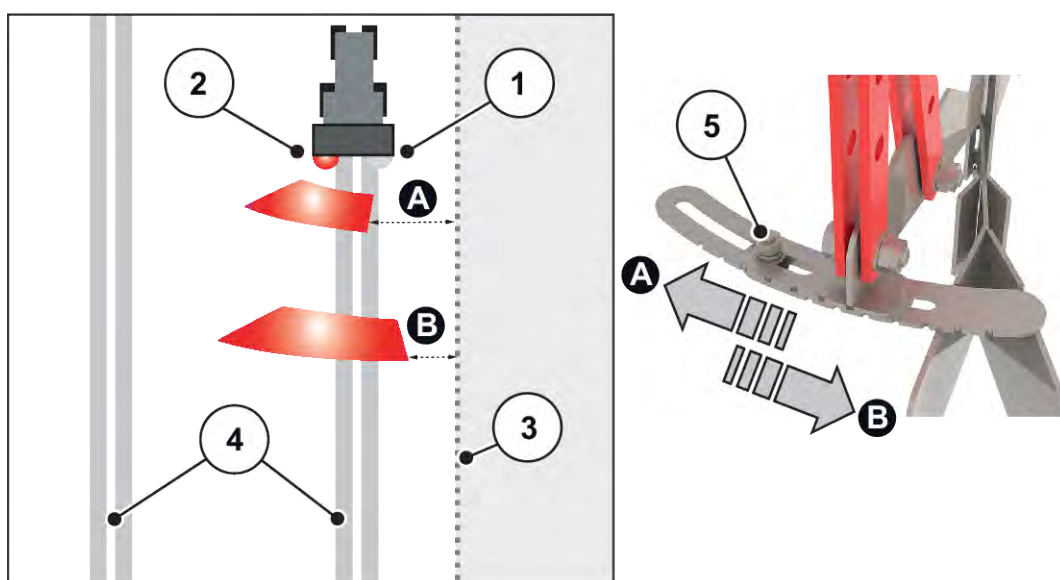
Rys. 52: Ustawienie urządzenia do wysiewu granicznego
