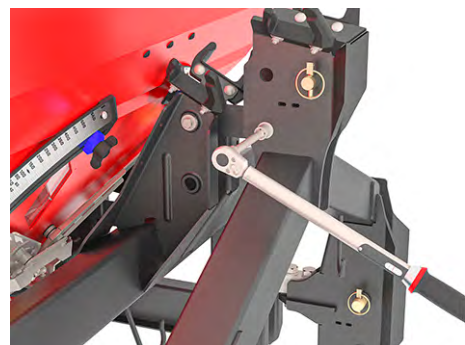
Rys. 62: Mocowanie cięgła do ramy wagi
