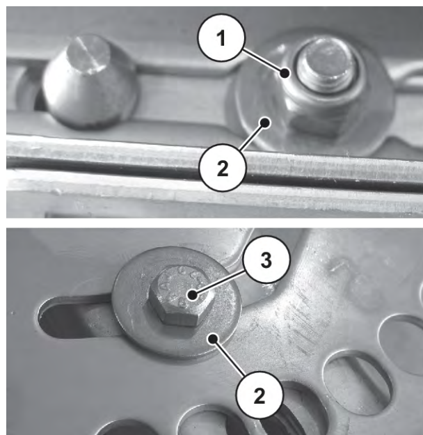
Rys. 90: Punkty mocowania łopatek rozrzucających
