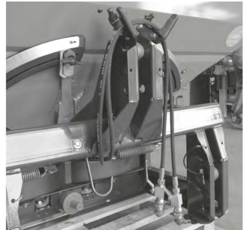
Rys. 60: Schowek na wał przegubowy, schowek na kable i giętkie przewody hydrauliczne
