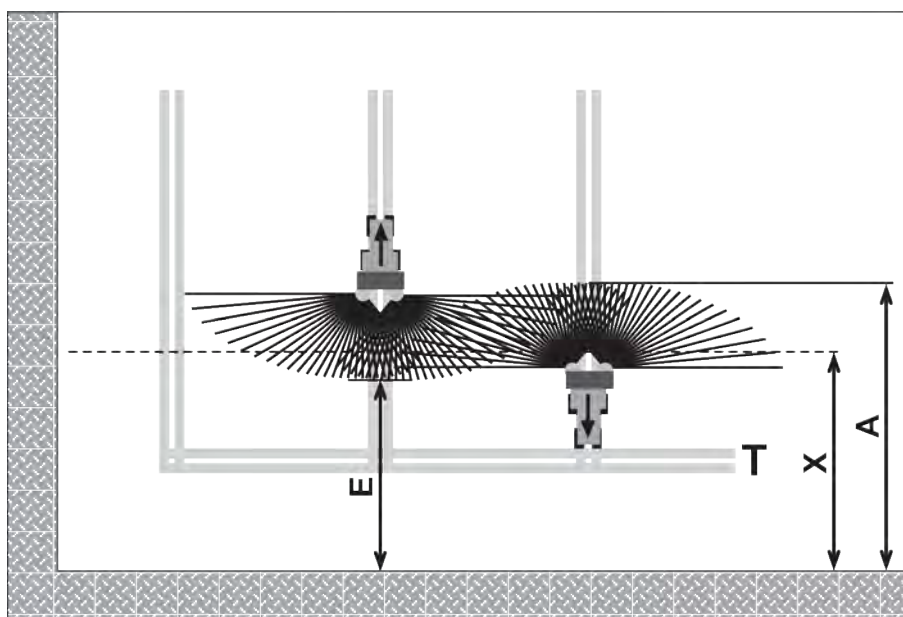
Rys. 56: Wysiew normalny
