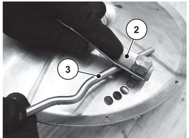
Pav. 79: Plokščiosios spyruoklės atlaisvinimas
