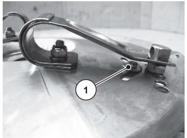
Pav. 78: Barstymo disko plokščioji spyruoklė
