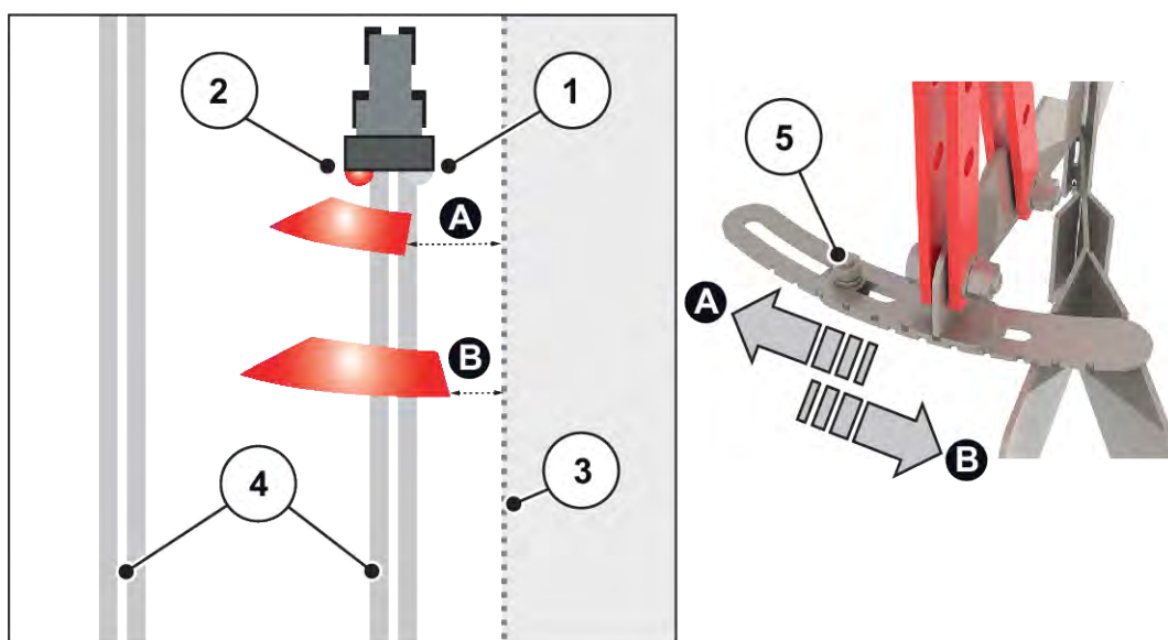
Pav. 52: Paribių barstymo įrenginio nustatymas
