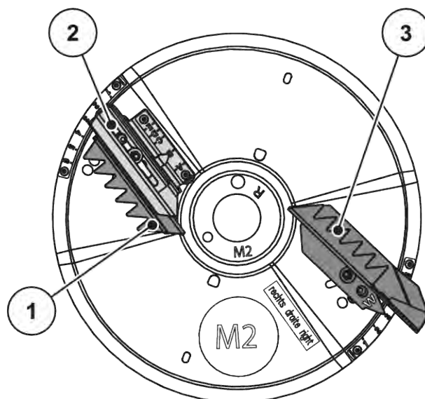
Pav. 93: Barstymo diskas M2
