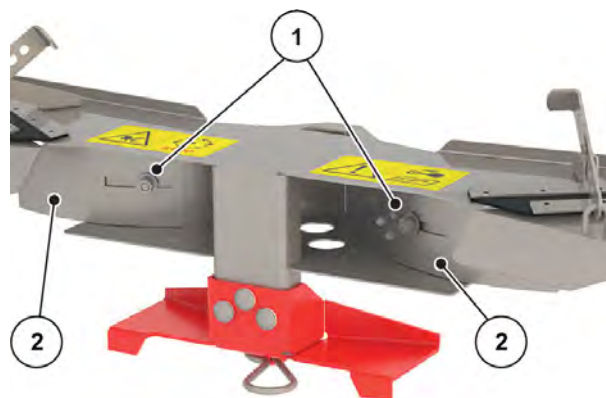
Pav. 58: Barstymo eilėmis įrenginio plokštelė
