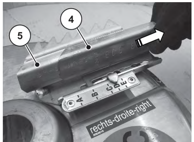
Pav. 80: Ilginamoji ir pagrindinė mentė
