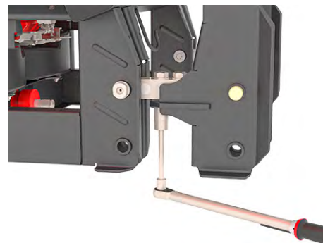
Pav. 61: Svorio jutiklio pritvirtinimas (važiavimo kryptimi dešinėje pusėje)
