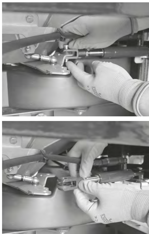
Pav. 69: Hidraulinio cilindro ištraukimas
