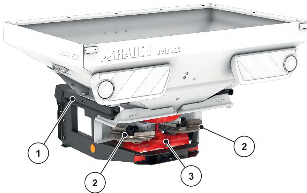
Pav. 9: Konstrukcinių grupių apžvalga: Užpakalinės pusės
