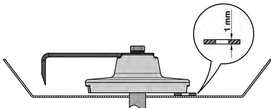
Pav. 76: Maišytuvo nustatymas
