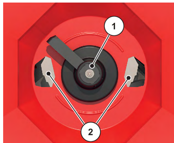
Фиг. 11: Бъркалка
