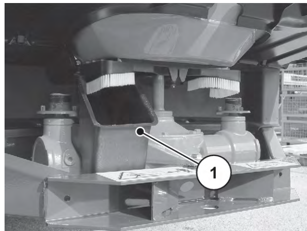
Фиг. 38: Закачване на улея за калибриране
