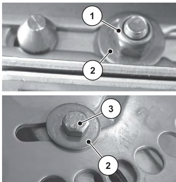
Фиг. 90: Точки на закрепване на разпръскващите лопатки
