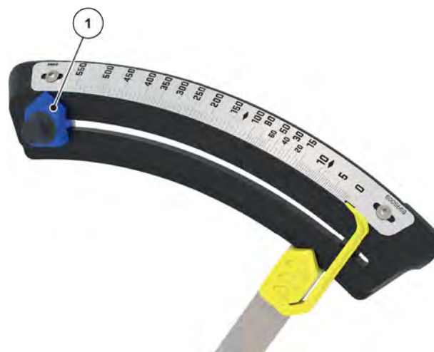
Фиг. 42: Скала за настройка на количеството използван тор (по посока на движението отдясно, вариант Q)
