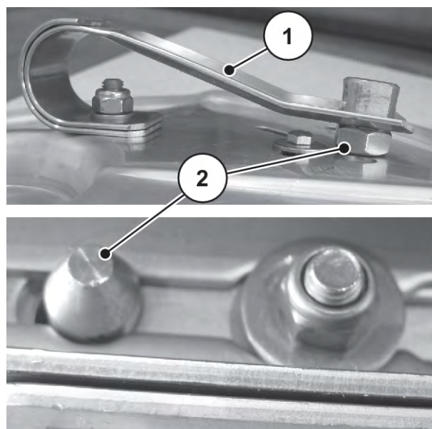
Фиг. 75: Фиксиращият болт е фиксиран правилно.
