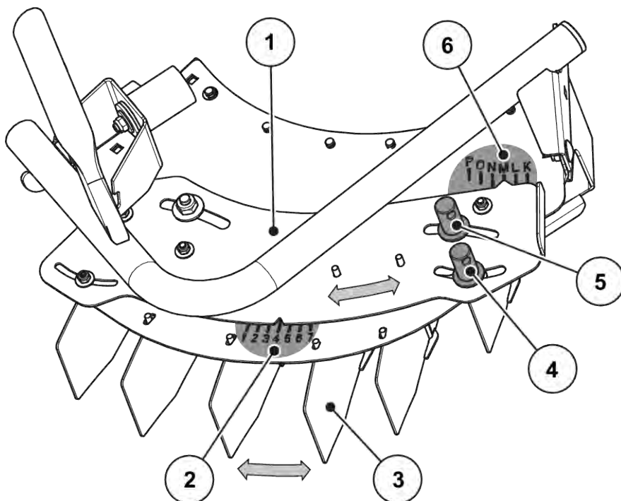
Фиг. 53: Настройка на устройството TELIMAT
