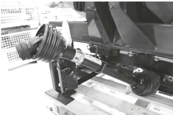
Фиг. 60: Място за съхранение на карданныя вал, на кабелите и на хидравличните маркучи
