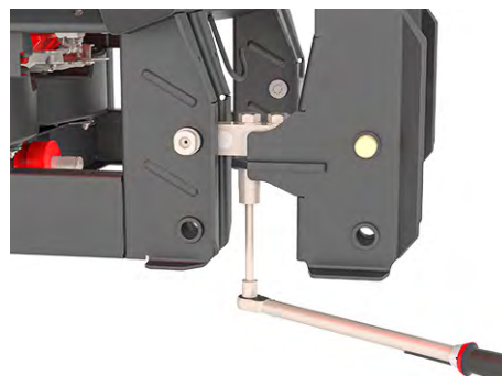
Фиг. 61: Закрепване на датчика за маса (по посока на движението отъясно)
