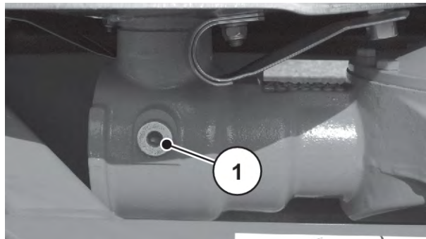
Фиг. 94: Места за пълнене и източване на трансмисионното масло
