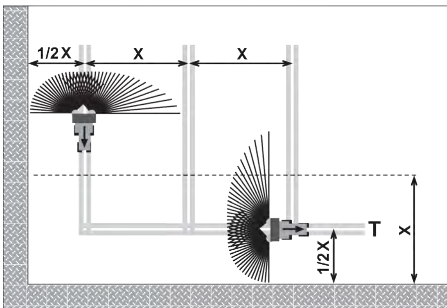
Фиг. 55: Гранично разпръскване
