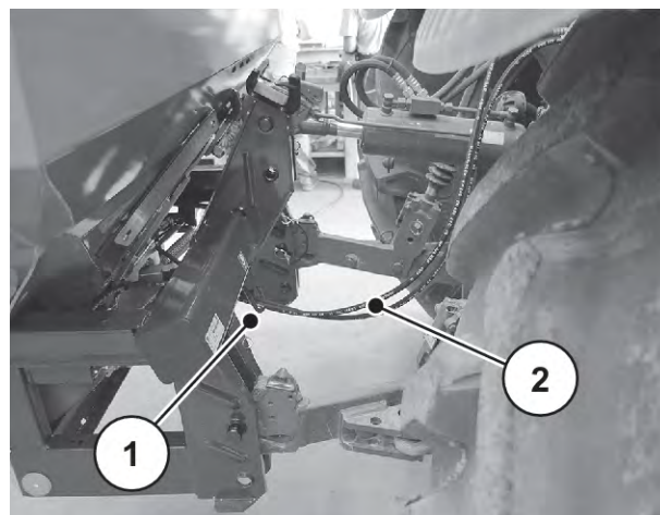
Фиг. 25: Направление на хидравлични маркучи
