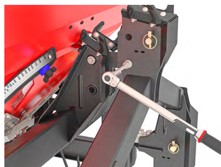
Фиг. 62: Закрепване на разтегателния прът на претеглящата рама
