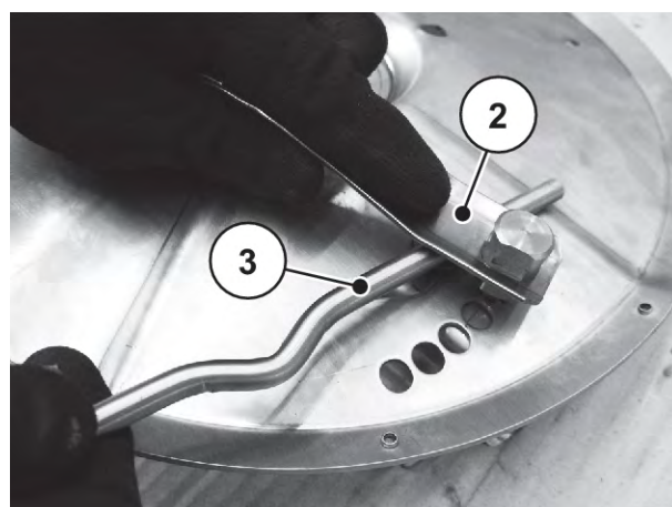
Фиг. 79: Освобождаване на плоската пружина
