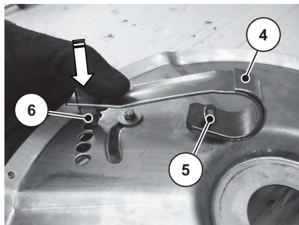
Фиг. 91: Плоска пружина на разпръскващия диск
