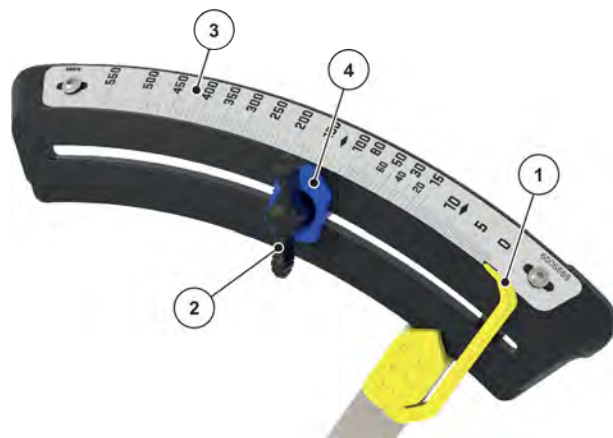
Фиг. 41: Скала за настройка на количеството използван тор (по посока на движението отдясно, варианти K/D/C)
