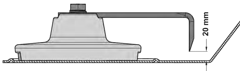
Фиг. 73: Зона на износване на разбъркващия елемент
