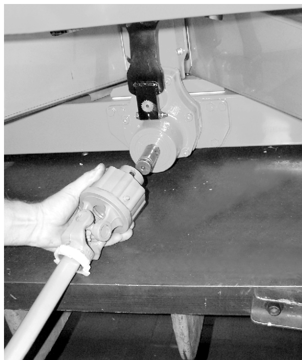
Фиг. 20: Поставяне на карданния вал върху края на вала на редуктора
