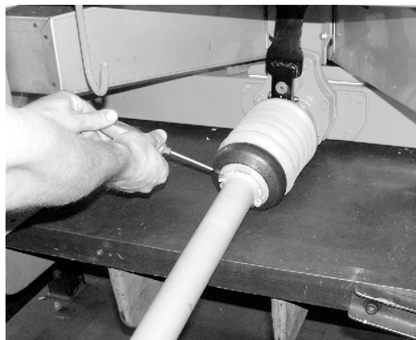
Фиг. 23: Фиксиране на защитата на карданныя вал
