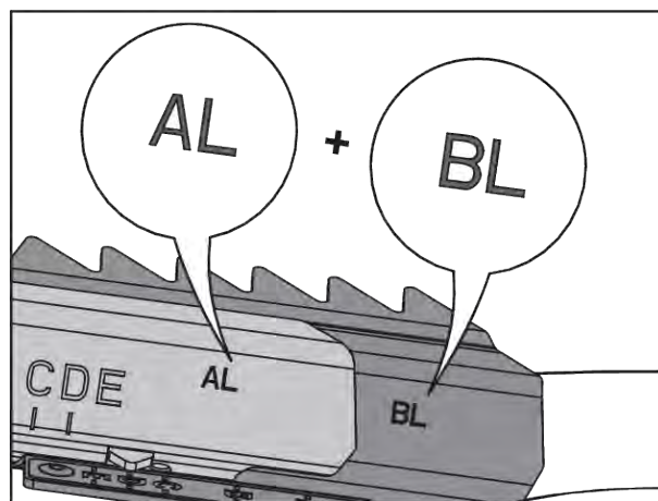
Фиг. 77: Комбинация от разпръскващи лопатки
