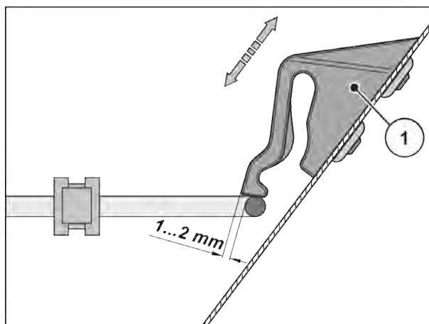
Фиг. 65: Контролен размер за проверка на функционирането на блокировката на предпазната решетка
