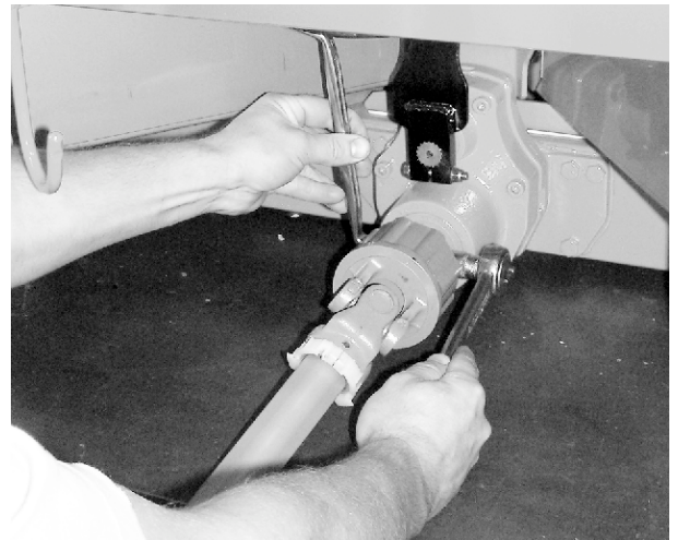
Фиг. 21: Закрепване на карданный вал
