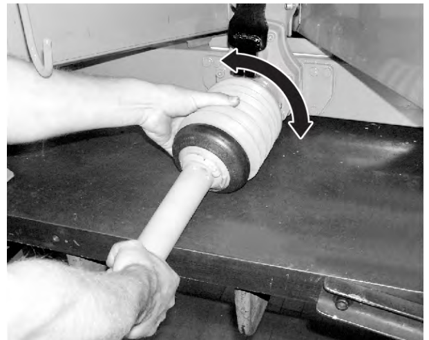
Фиг. 22: Поставяне на защитата на карданный вал
