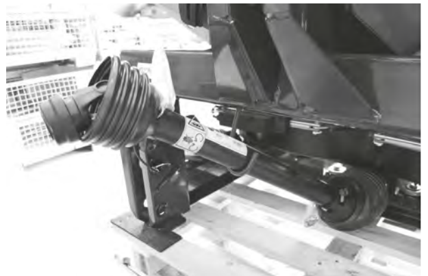
Фиг. 18: Държач на карданния вал
