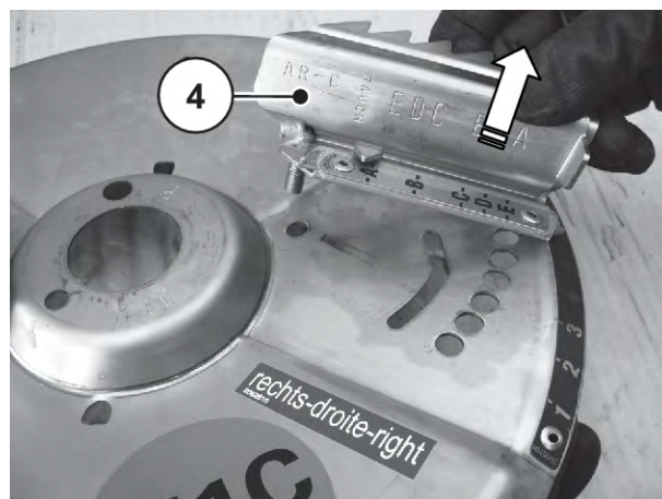
Фиг. 91: Сваляне на разпръскващата лопатка
