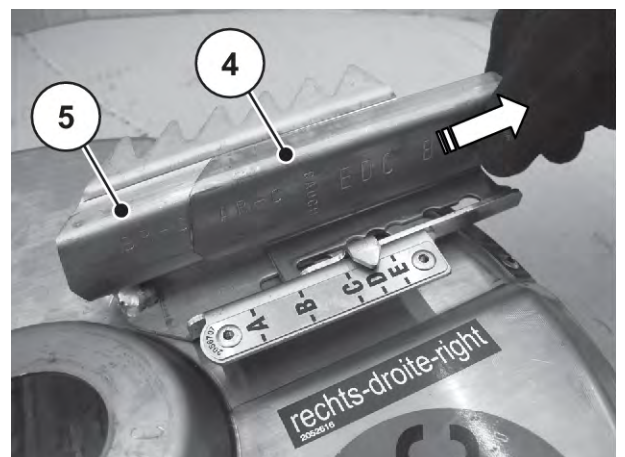
Фиг. 84: Удължителна и главна лопатка
