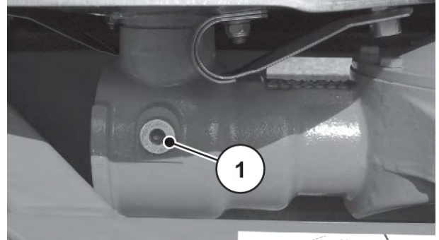
Фиг. 98: Места за пълнене и източване на трансмисионното масло
