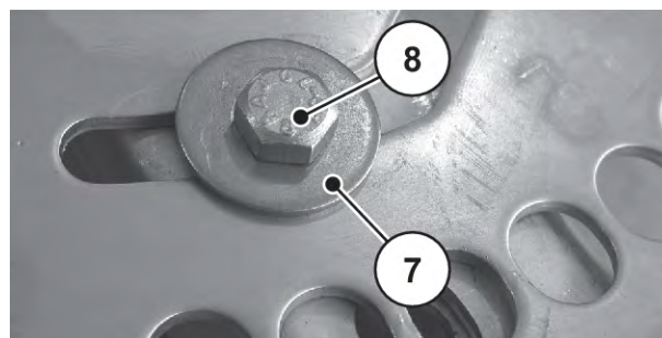
Фиг. 86: Точки на закрепване на разпръскващите лопатки
