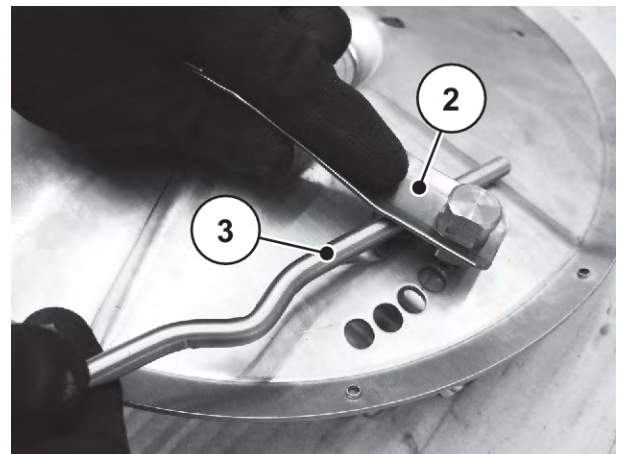
Фиг. 83: Освобождение на плоската пружина
