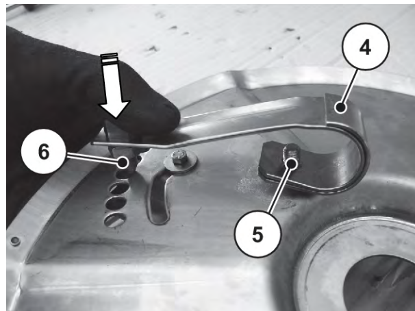
Фиг. 95: Плоска пружина на разпръскващия диск
