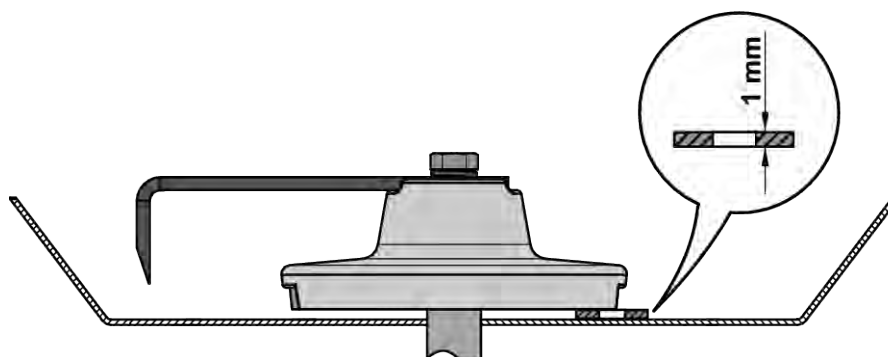
Фиг. 80: Настройка на бъркалката
