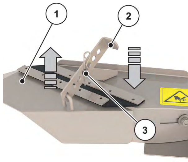
Фиг. 63: Регулиране на устройството за редово разпръскване
