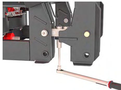
Фиг. 65: Закрепване на датчика за маса (по посока на движението отдясно)
