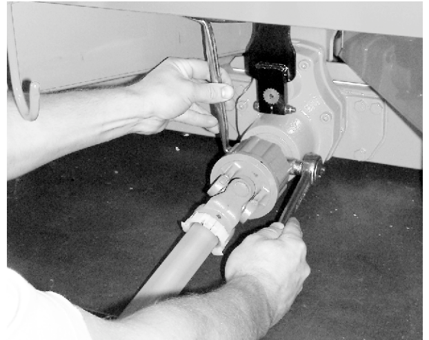
Фиг. 21: Закрепване на карданния вал
