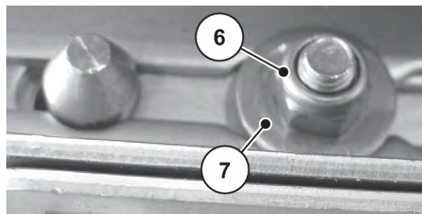
Фиг. 85: Нова удължителна лопатка
