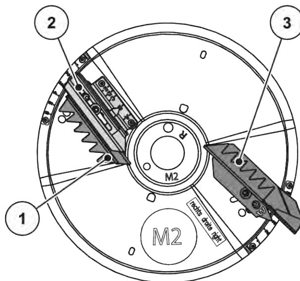
Фиг. 97: Разпръскващ диск M2
