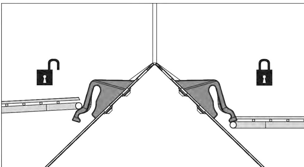
Рис. 63: Блокировочное устройство защитной сетки открыто/закрыто
