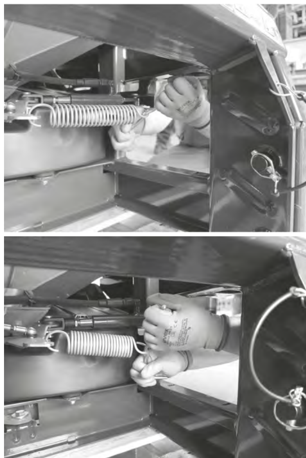
Рис. 67: Отцепление пружины
