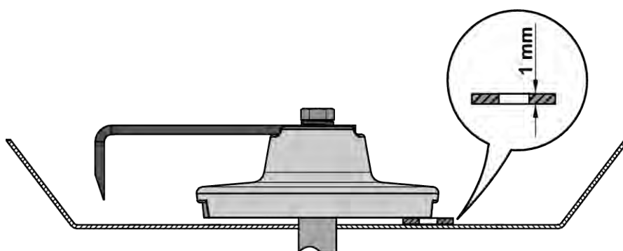
Рис. 76: Настройка мешалки
