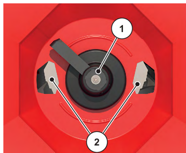
Рис. 11: Мешалка
