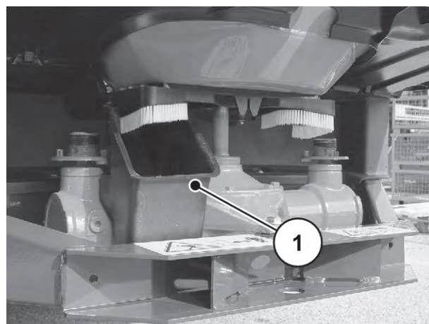
Рис. 38: Навешивание лотка для установки нормы внесения
