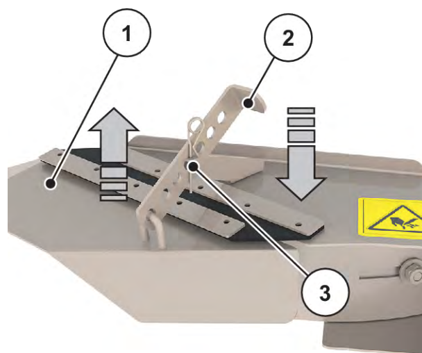
Рис. 59: Регулировка на приспособлении для внесения по рядам
