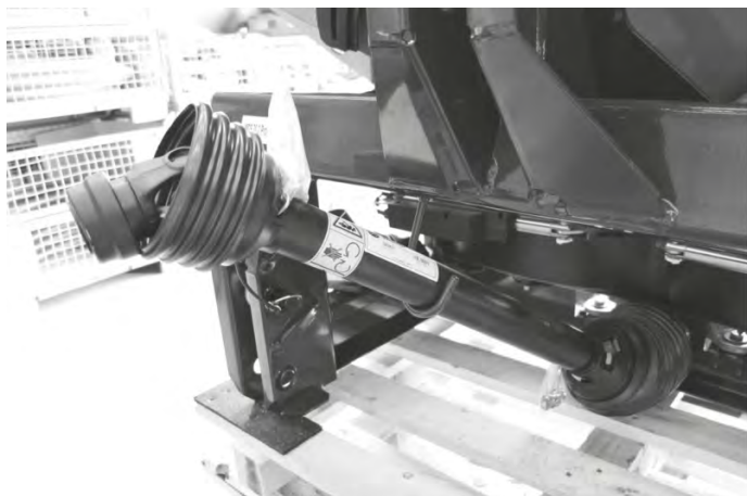
Рис. 60: Место размещения карданного вала, кабелей и гидравлических шлангов
