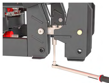
Рис. 61: Крепление датчика массы (справа относительно направления движения)
