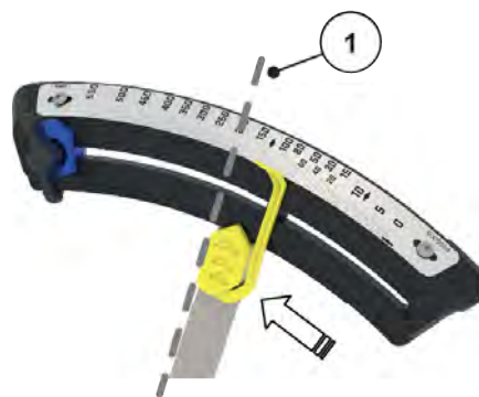
Рис. 70: Смещение индикатора положения
