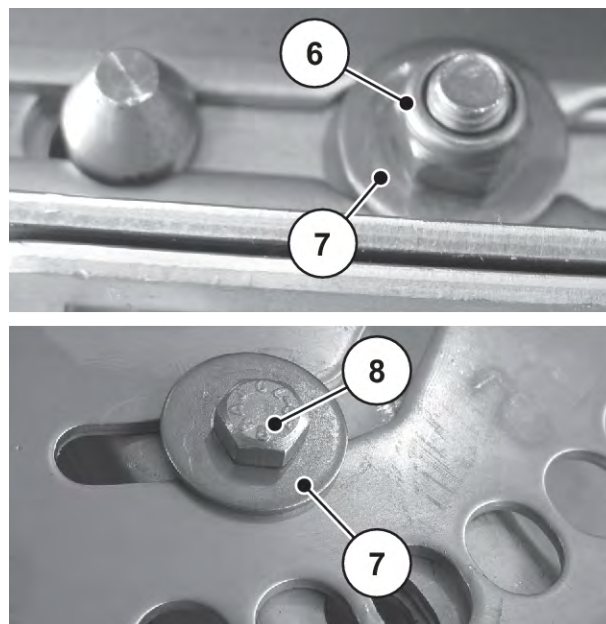
Рис. 82: Точки крепления лопаток для разбрасывания
