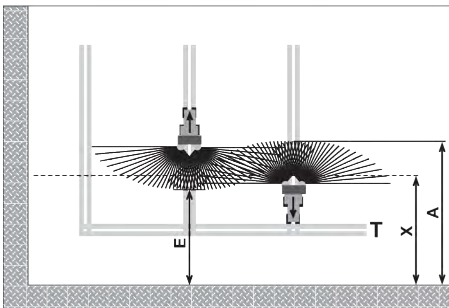
Рис. 56: Нормальное внесение
