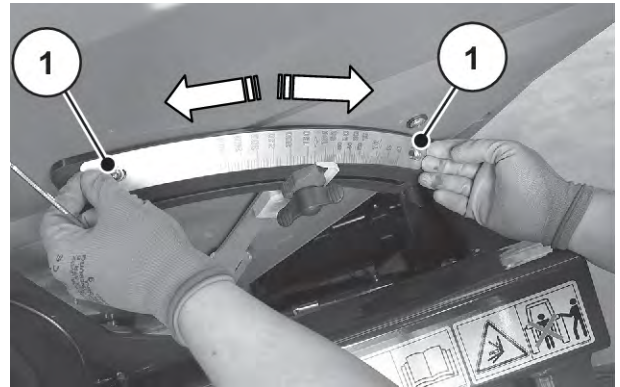
Рис. 72: Перемещение шкалы
