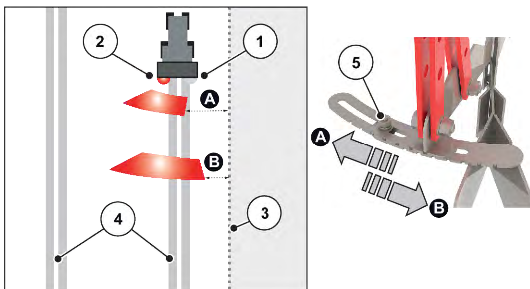
Рис. 52: Регулировка устройства внесения на границе поля
