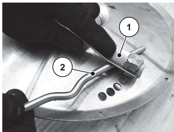
Рис. 85: Снятие плоской пружины
