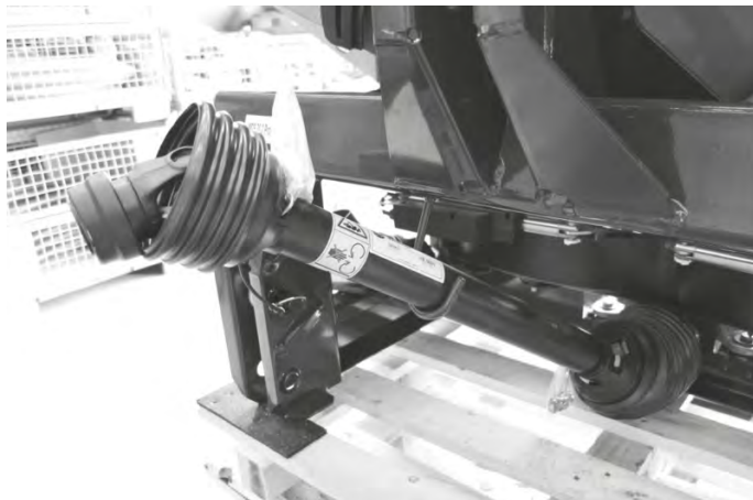
Obr. 60: Uložení kloubového hřídele, uložení kabelů a hydraulických hadic
