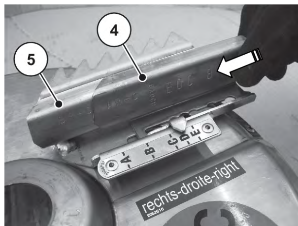
Obr. 81: Nová prodlužovací lopatka
