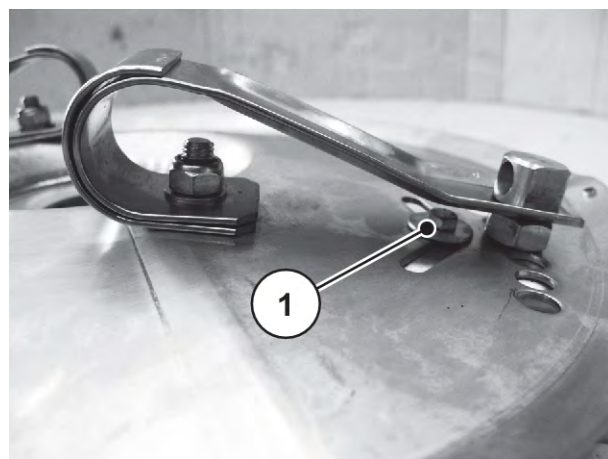
Obr. 78: Plochá pružina rozmetacího disku
