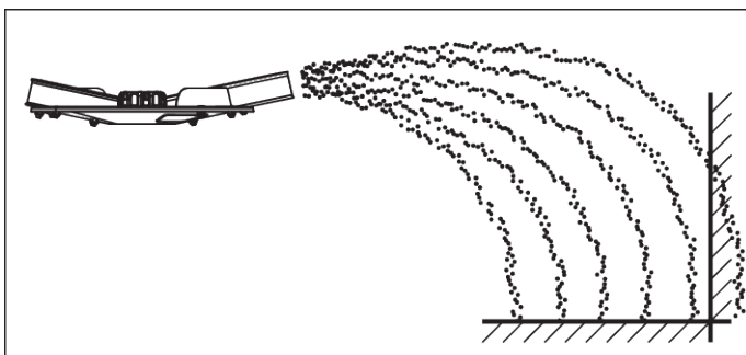
Obr. 47: Okrajové rozmetání při normálním hnojení
