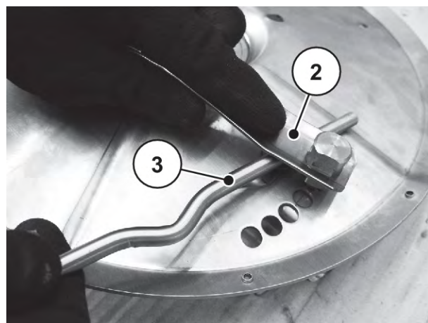
Obr. 79: Uvolnění ploché pružiny
