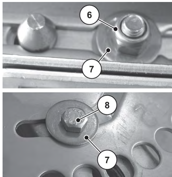
Obr. 82: Upevňovací body rozmetacích lopatek
