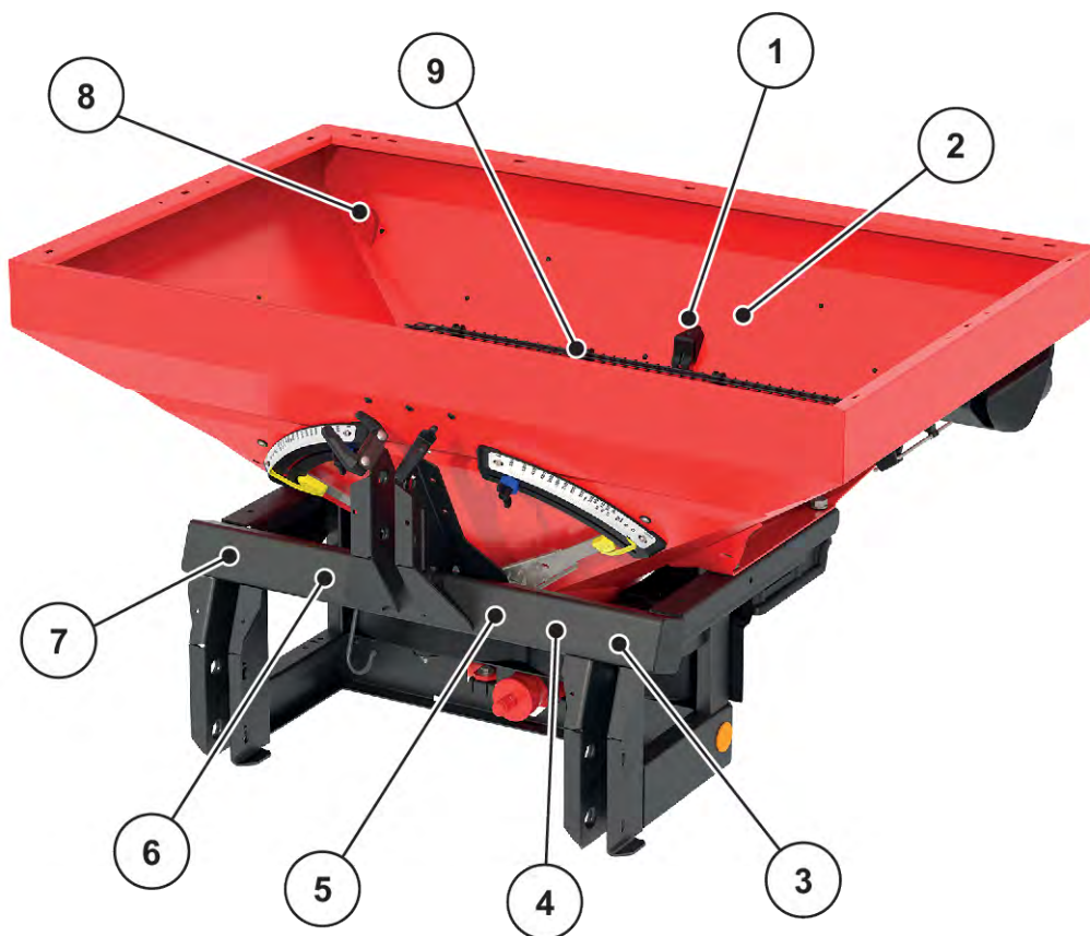
Obr. 2: Umístění ochranných zařízení, výstražných a instruktážních pokynů, odrazových světél (vpředu)
