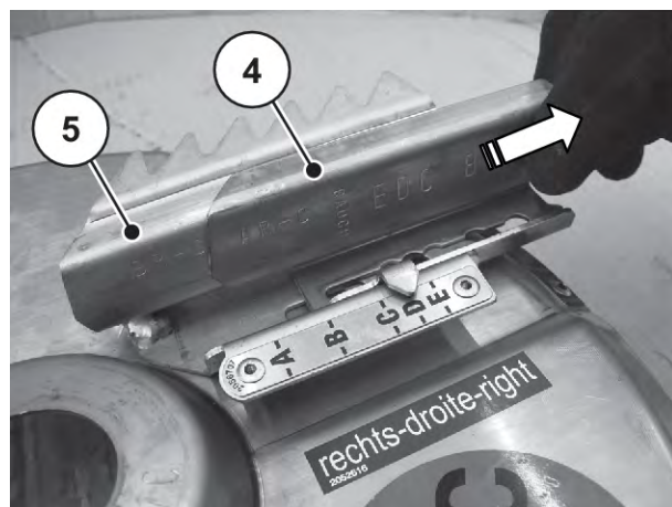
Obr. 80: Prodlužovací a hlavní lopatka
