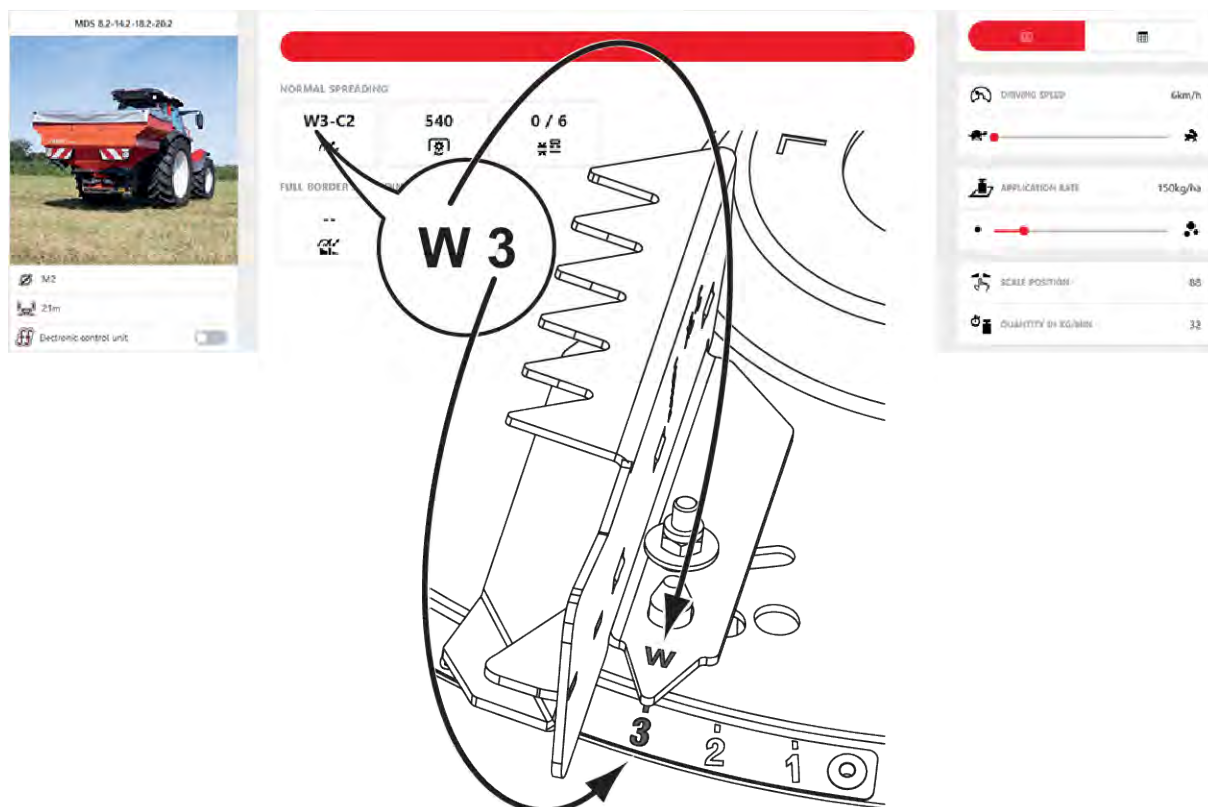
Obr. 44: Nastavení rozmetací lopatky, rozmetací disk M2, poloha W3; W: pevné nastavení délky 1 až 6: nastavení úhlu
