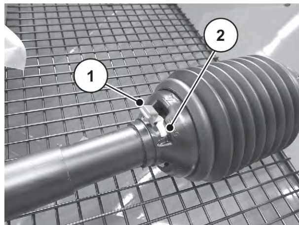
Obr. 13: Otevření krytu kloubového hřídele
