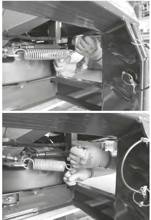
Afb. 67: Veer eruit nemen
