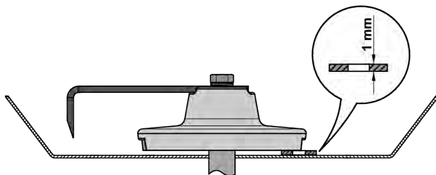
Afb. 76: Instelling van het roerwerk
