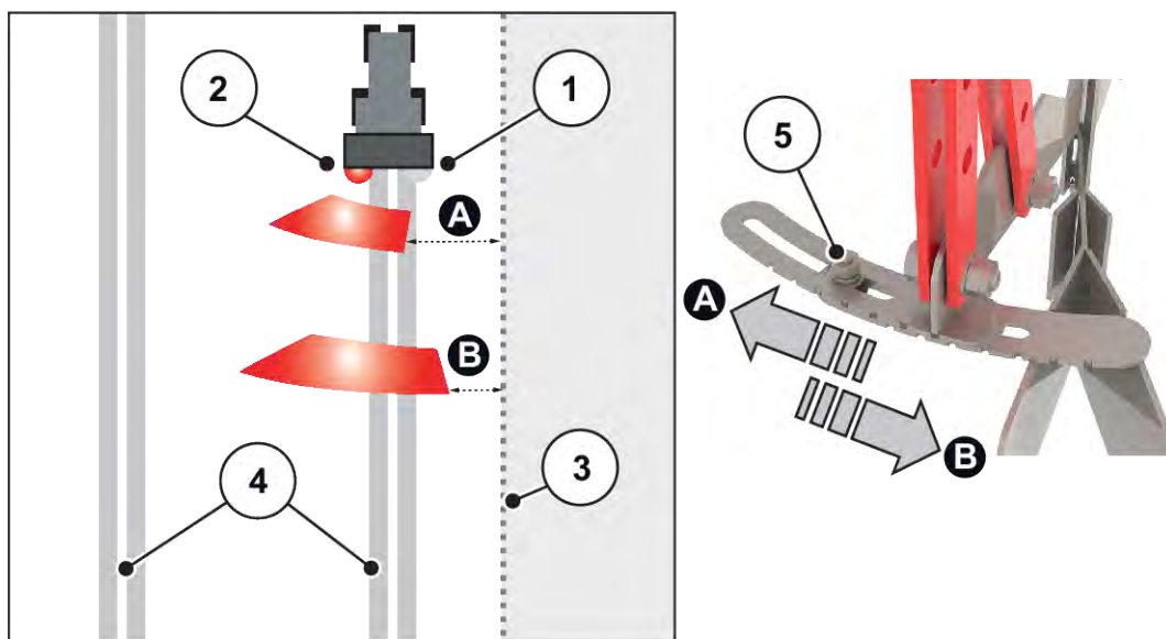
Afb. 52: Instelling van de grensstrooi-inrichting
