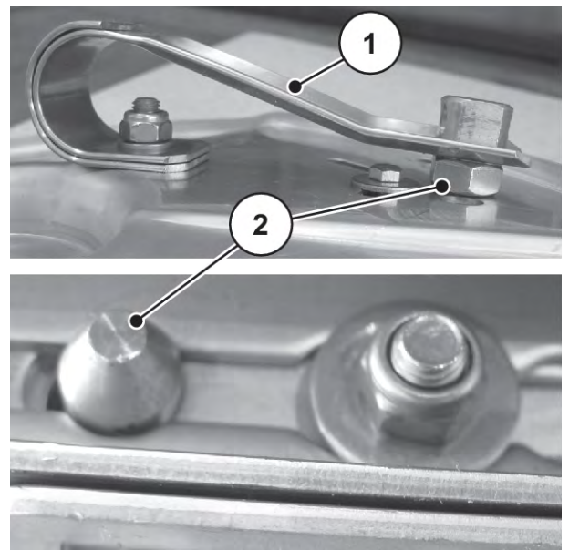
Afb. 75: Vergrendelingsbout naar behoren vergrendeld
