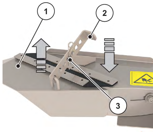
Afb. 59: Verstelling aan de rijenstrooier
