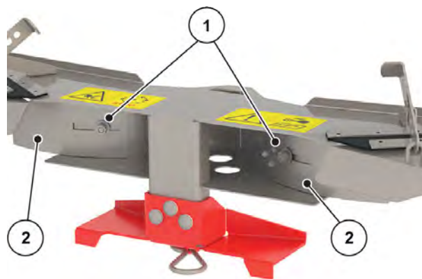
Afb. 58: Platen aan de rijenstrooier
