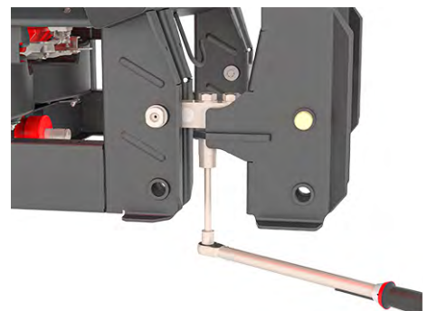
Afb. 61: Bevestiging van de weegcel (in rijrichting rechts)
