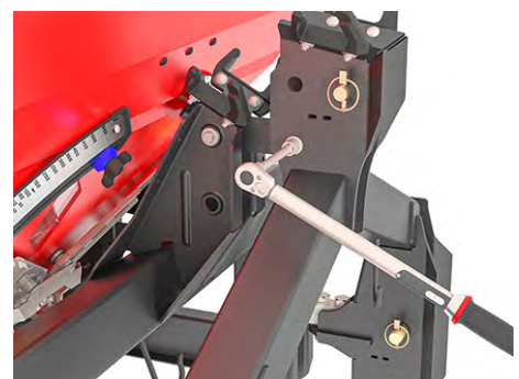
Afb. 62: Bevestiging van de trekstaaf aan het weegframe
