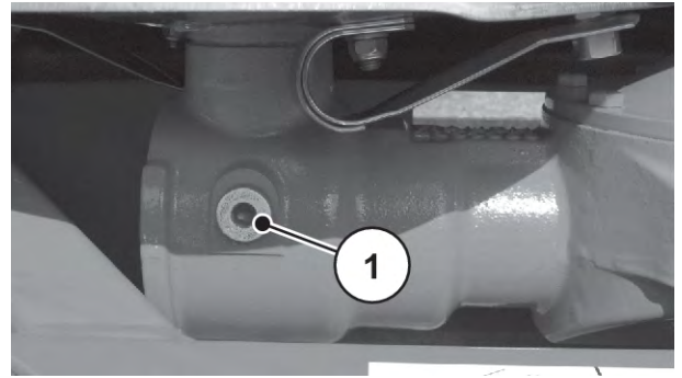
Afb. 93: Vul- en aftappunten voor drijfwerkolie
