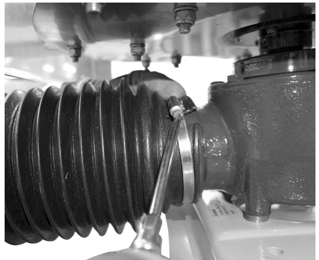
Afb. 14: Aftakasbescherming aanbrengen.
