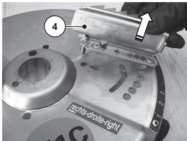
Afb. 89: Strooschoep verwijderen
