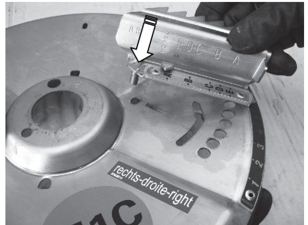
Afb. 90: Hoofdschoepmontage
