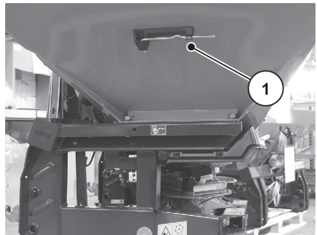
Afb. 8: Positie van de instelhendel
