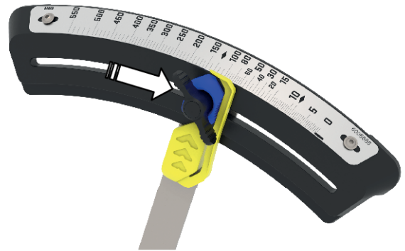
Afb. 73: Aanslag verschuiven
