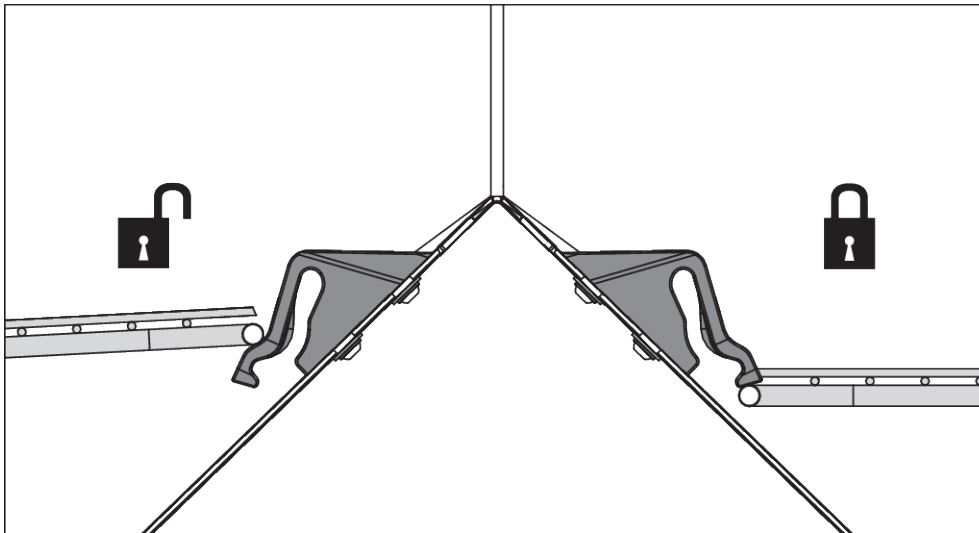
Afb. 65: Beschermroostervergrendeling open/gesloten
