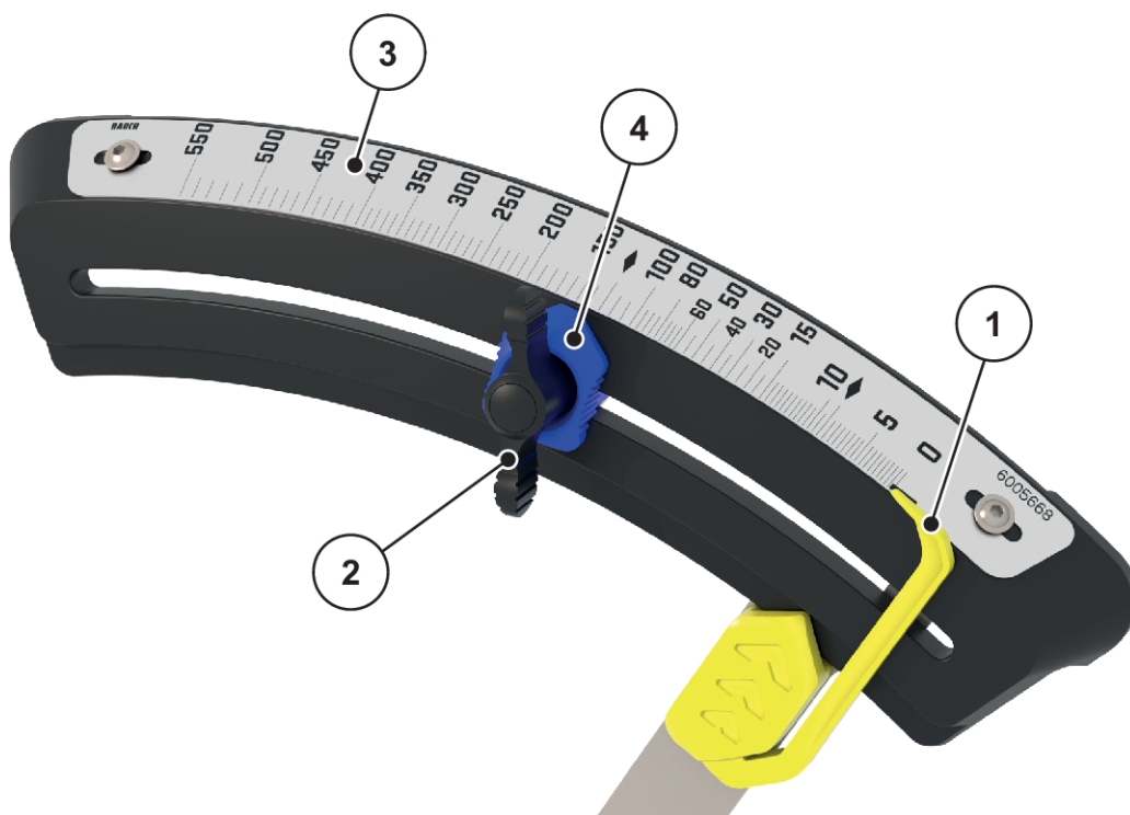
Afb. 39: Schaal voor instelling van de strooihoeveelheid (rijrichting rechts, varianten K/D/C)
