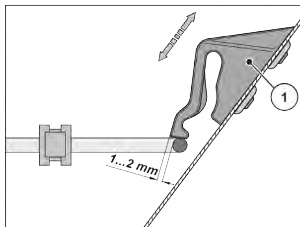
Fig. 65: Kontrolmål til funktionskontrol af beskyttelsesgitterlåsen
