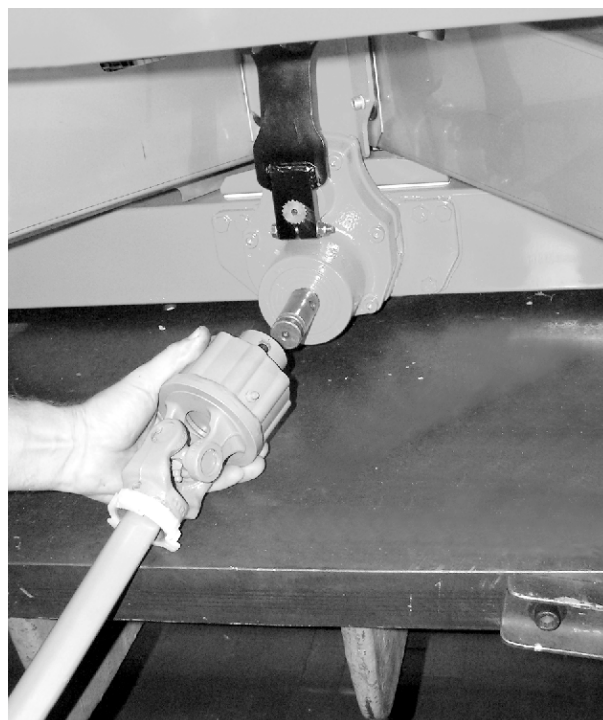
Fig. 20: Montering af kardanakslen på akseltappen
