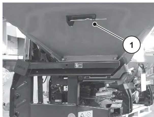
Fig. 10: Indstillingshåndtagets placering
