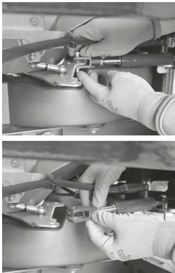
Fig. 69: Træk hydraulikcylinderen ud
