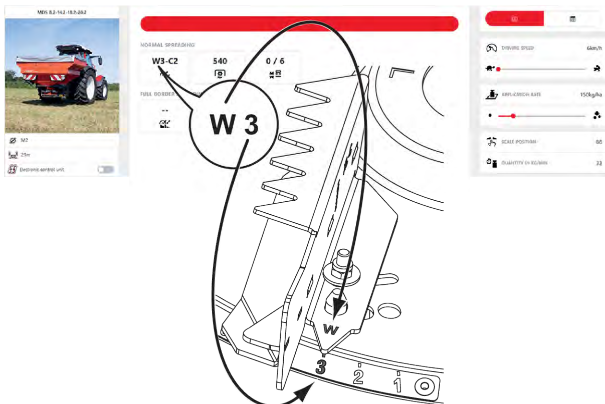
Fig. 44: Spredevingeindstilling spredeskive M2, stilling W3; W: fast længde indstilling 1 til 6: Vinkelindstilling
