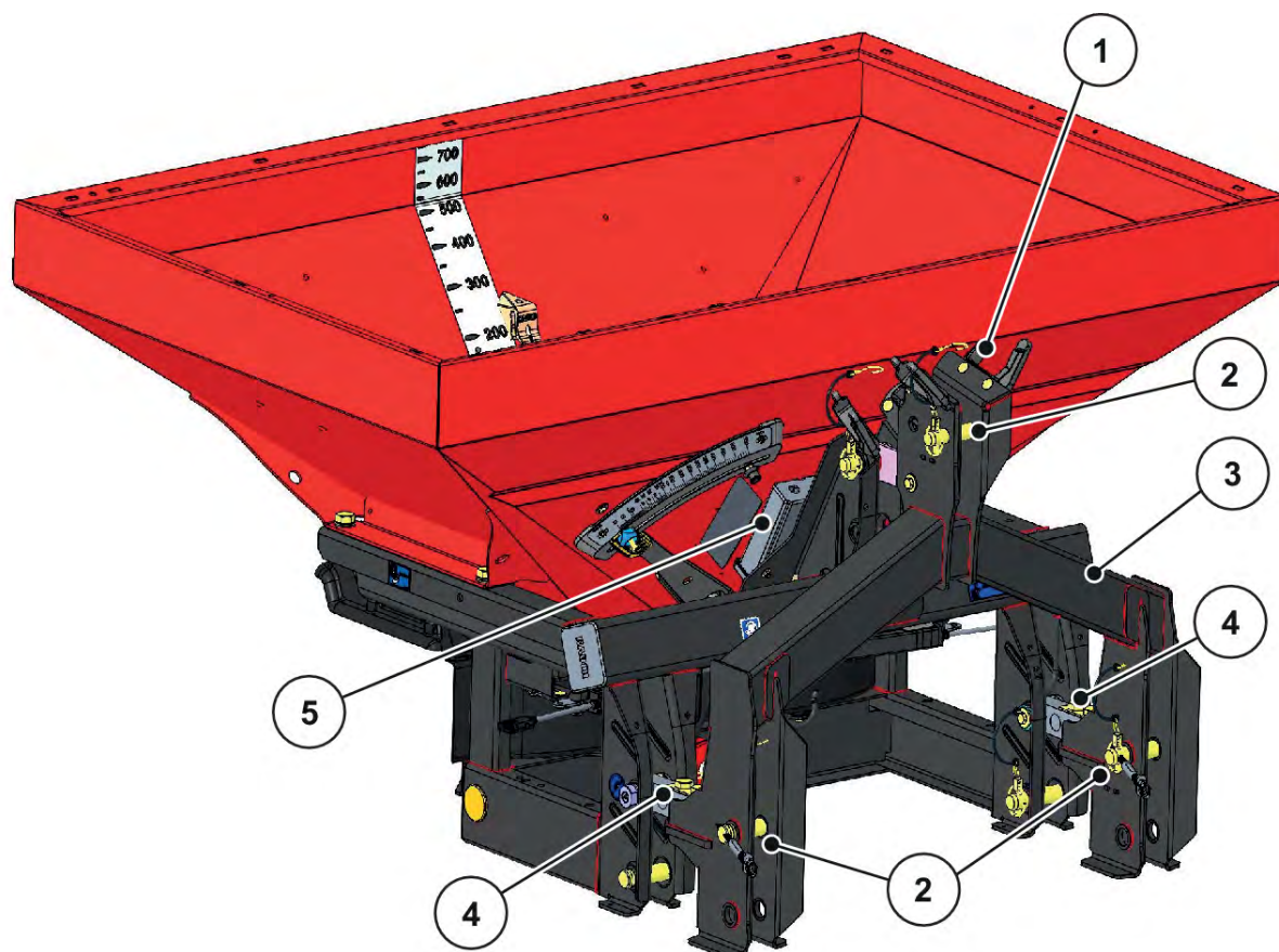
III. 8: Panoramica gruppi costruttivi: Lato anteriore MDS con ISOBUS con telaio di pesatura
