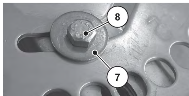
III. 82: Punti di fissaggio della paletta di lancio
