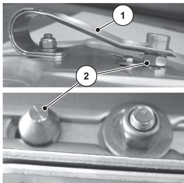
III. 75: Perno di arresto innestato correttamente
