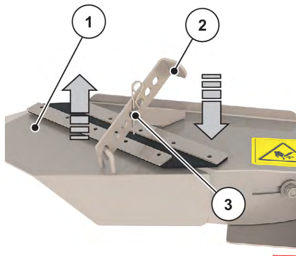
III. 59: Regolazione nel dispositivo di distribuzione a file
