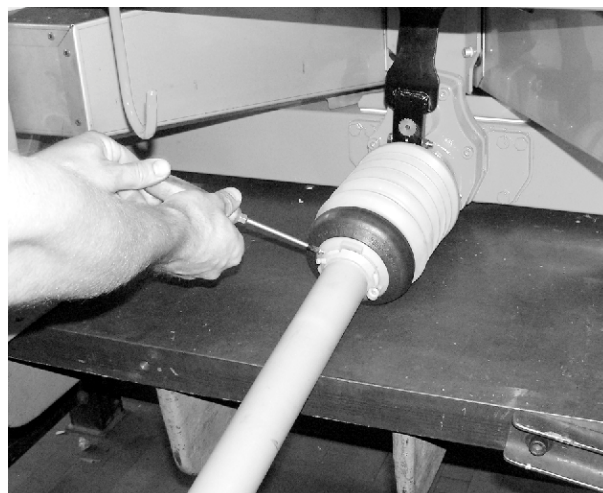
III. 23: Fissare la protezione dell'albero cardanico
