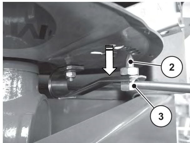
III. 45: Impostazione palette di lancio
