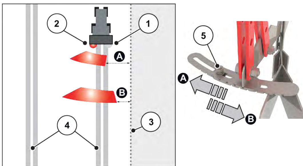
III. 52: Regolazione del sistema di distribuzione ai margini
