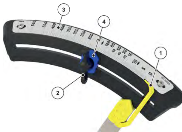
III. 41: Procedura per la regolazione della dose (a destra rispetto alla direzione di marcia, varianti K/D/C)
