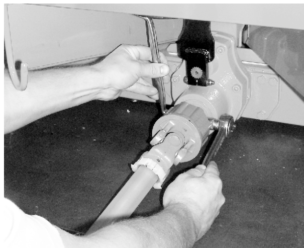
III. 21: Fissaggio dell'albero cardanico
