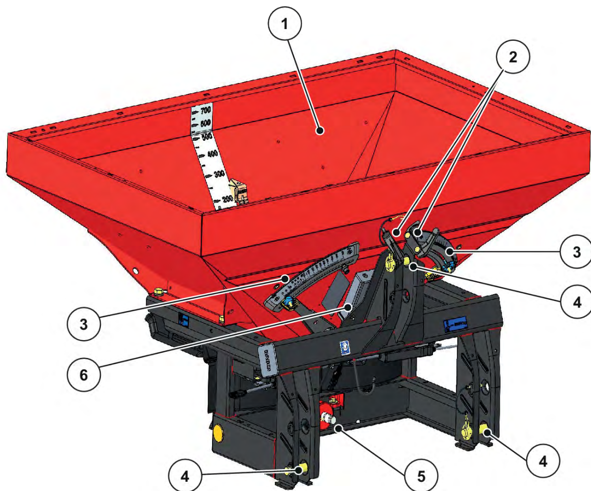
III. 7: Panoramica gruppi costruttivi: Lato anteriore MDS con ISOBUS
