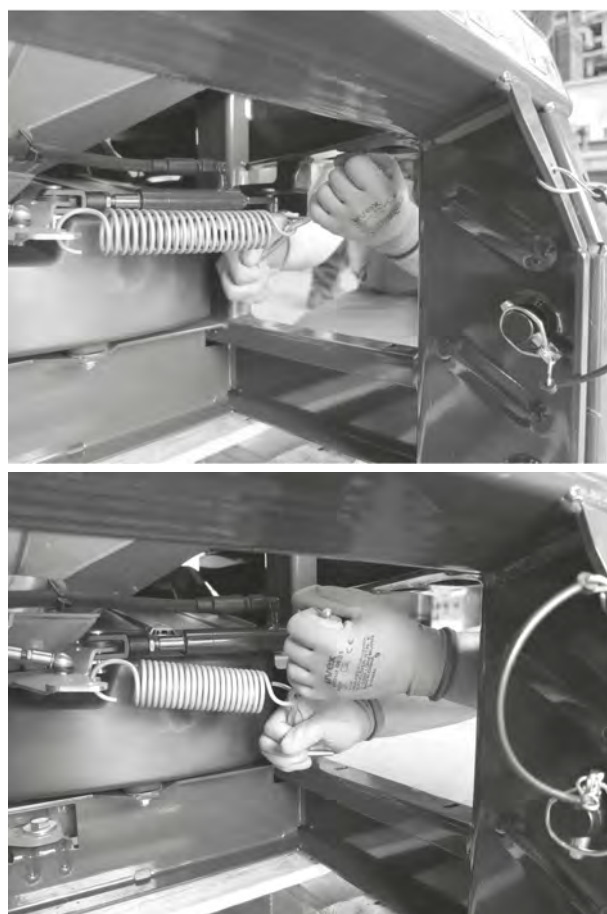
III. 67: Sganciare la molla
