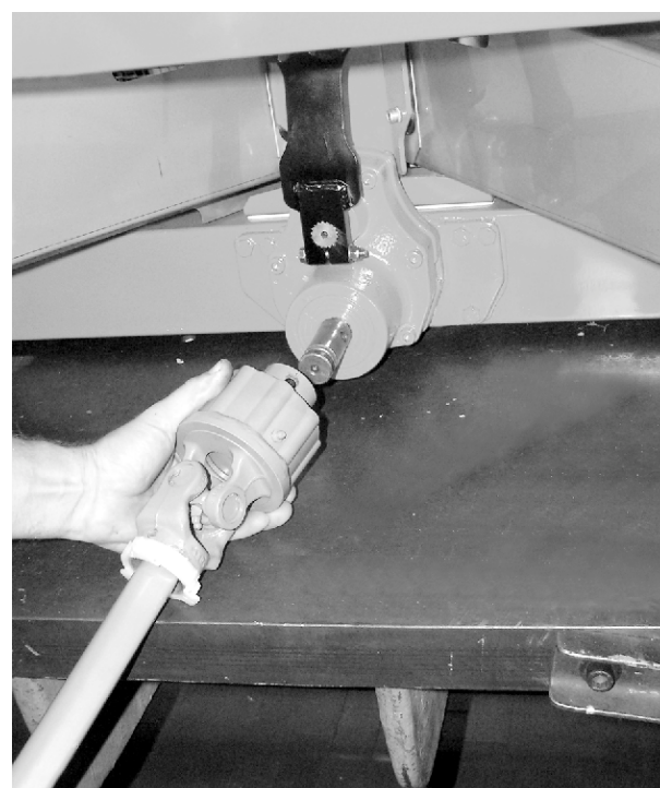
III. 20: Inserimento dell'albero cardanico sul perno del riduttore
