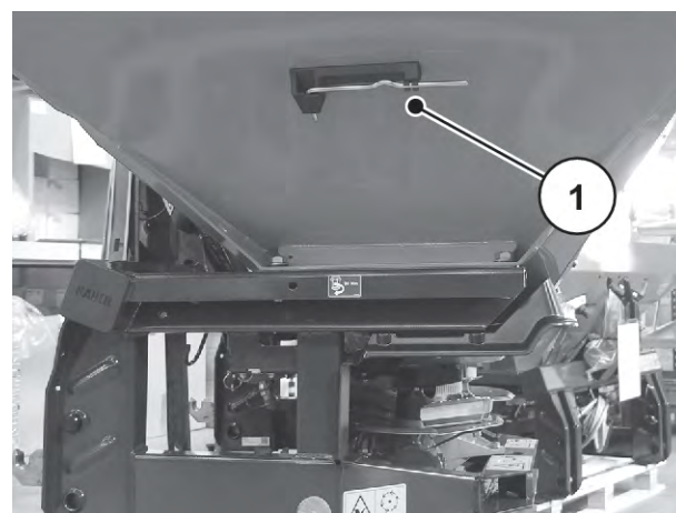
III. 10: Posizione della leva di regolazione
