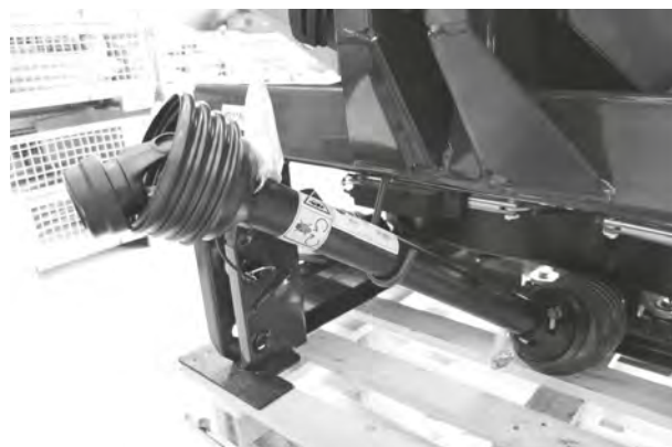
III. 18: Supporto dell'albero cardanico
