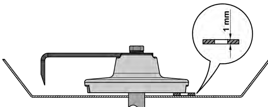
III. 76: Regolazione dell'agitatore
