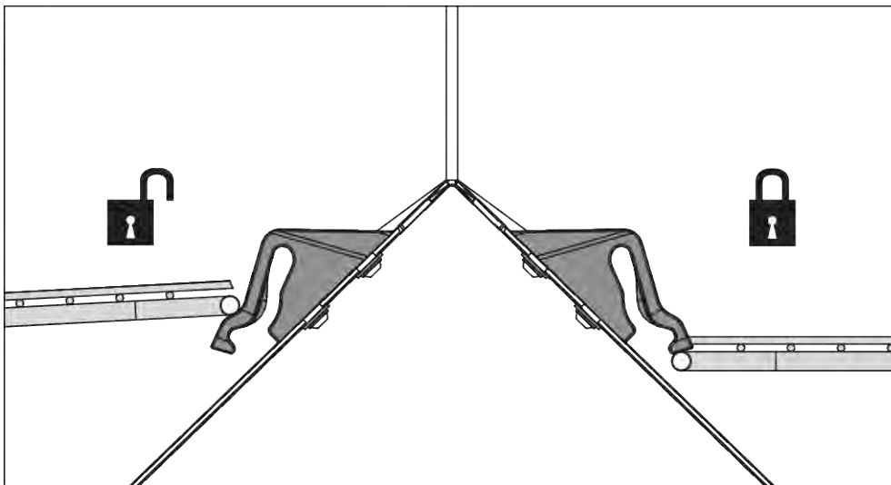
III. 63: Bloccaggio della griglia protettiva aperto/chiuso
