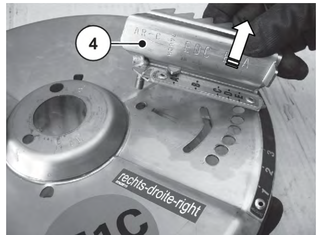
Abb. 87: Wurfflügel entnehmen
