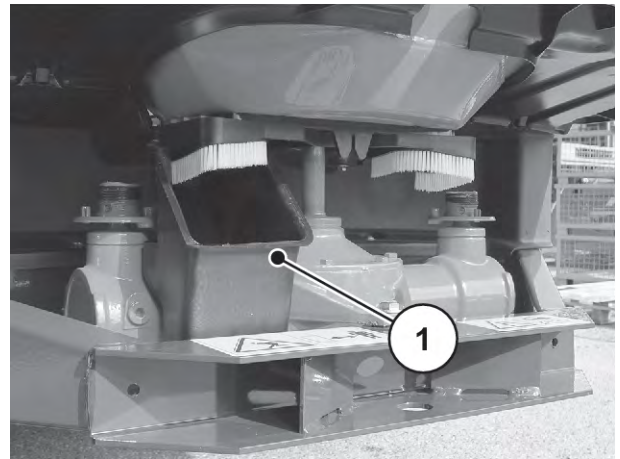
Abb. 38: Abdrehprobenrutsche einhängen
