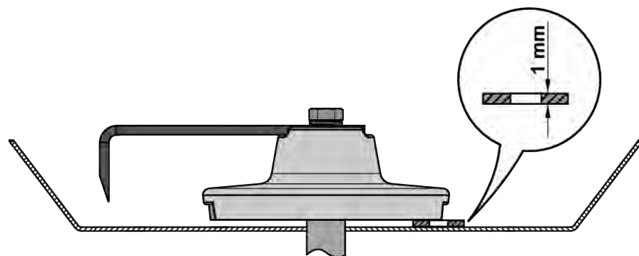
Abb. 76: Einstellung des Rührwerks
