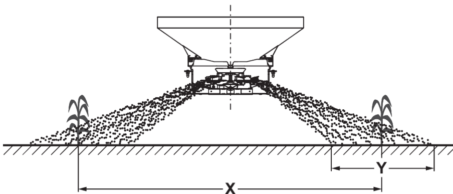
Abb. 57: Streuen mit Reihenstreuvorrichtung
