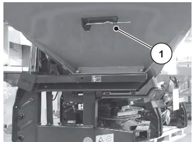
Abb. 36: Lage Einstellhebel
