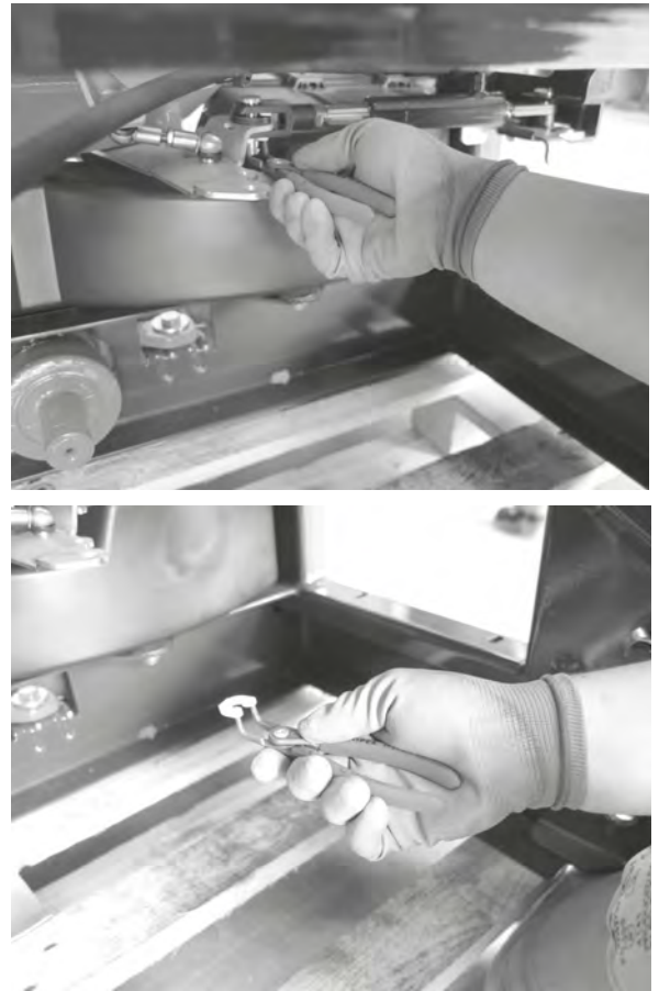
Abb. 68: Zylinder aushängen
