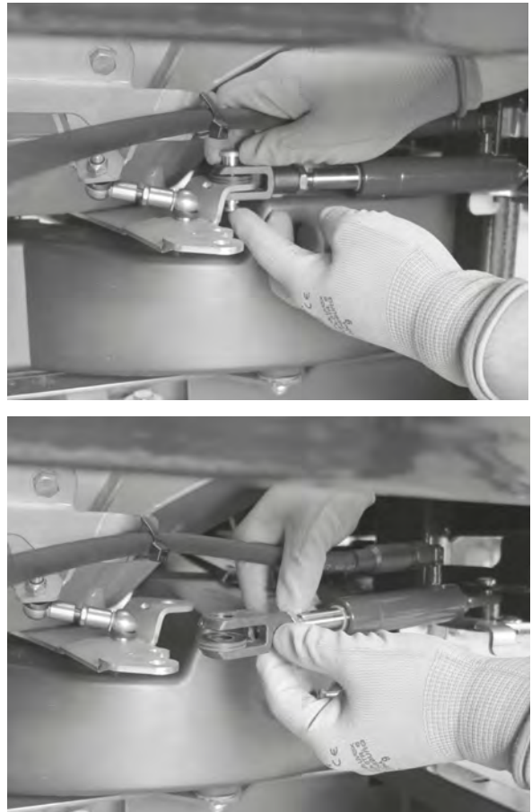
Abb. 69: Hydraulikzylinder herausziehen
