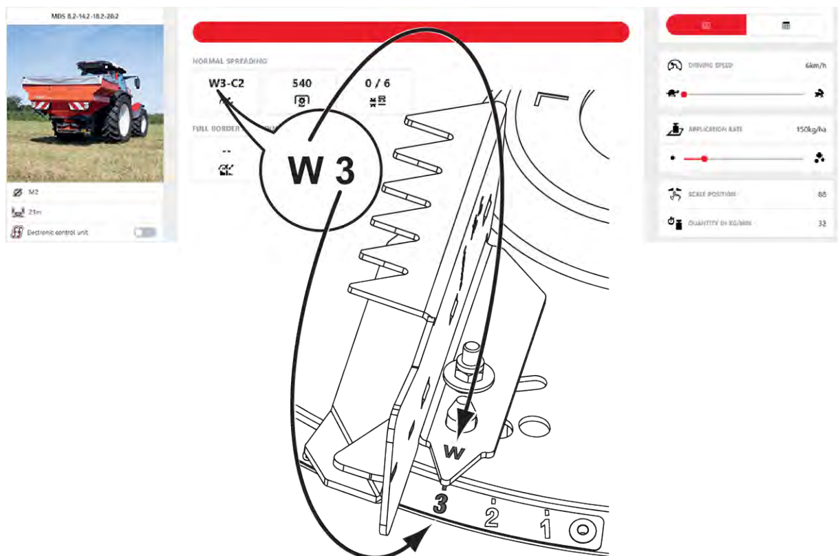
Abb. 44: Wurfblügeleinstellung Wurfscheibe M2, Stellung W3; W: feste Längeneinstellung 1 bis 6: Winkeleinstellung
