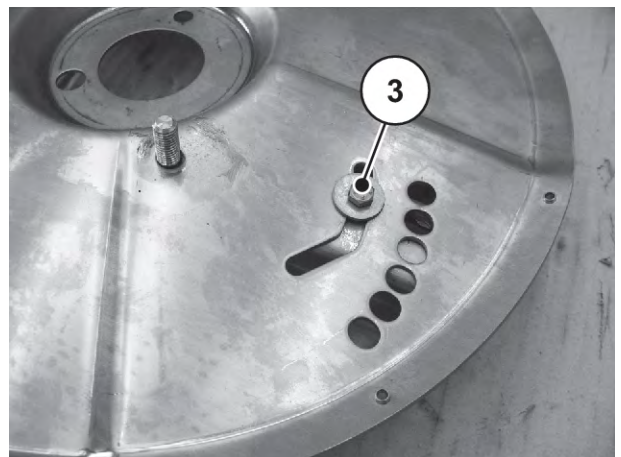
Abb. 86: Schraube an der Wurfscheiben- Unterseite
