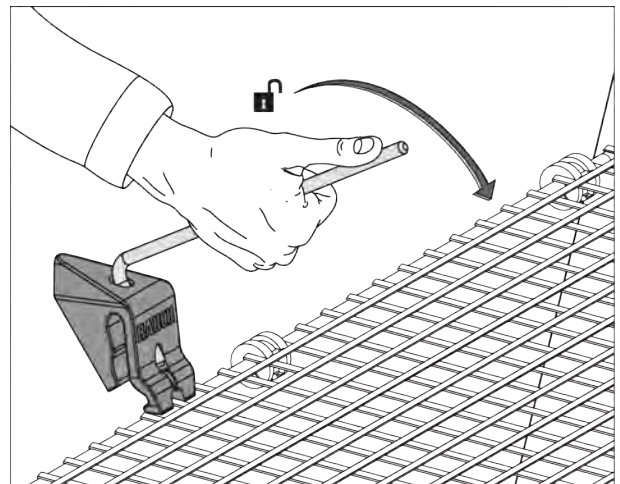
Abb. 64: Schutzgitterverriegelung öffnen
