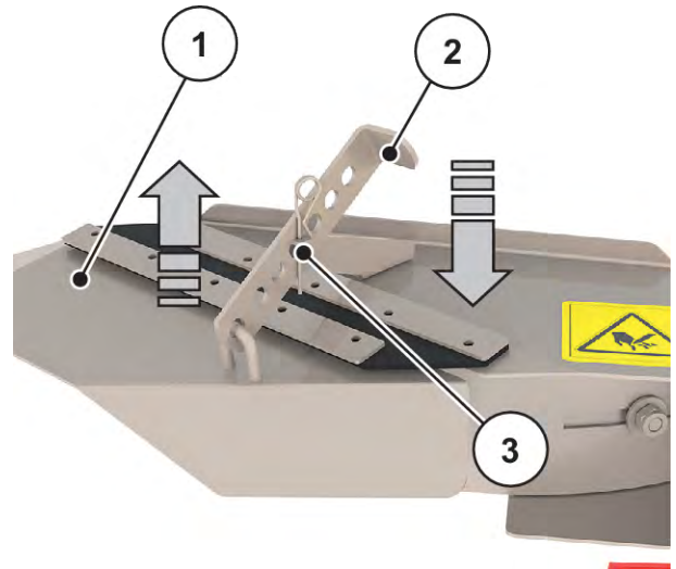
Abb. 59: Verstellung an der Reihenstreuvorrichtung
