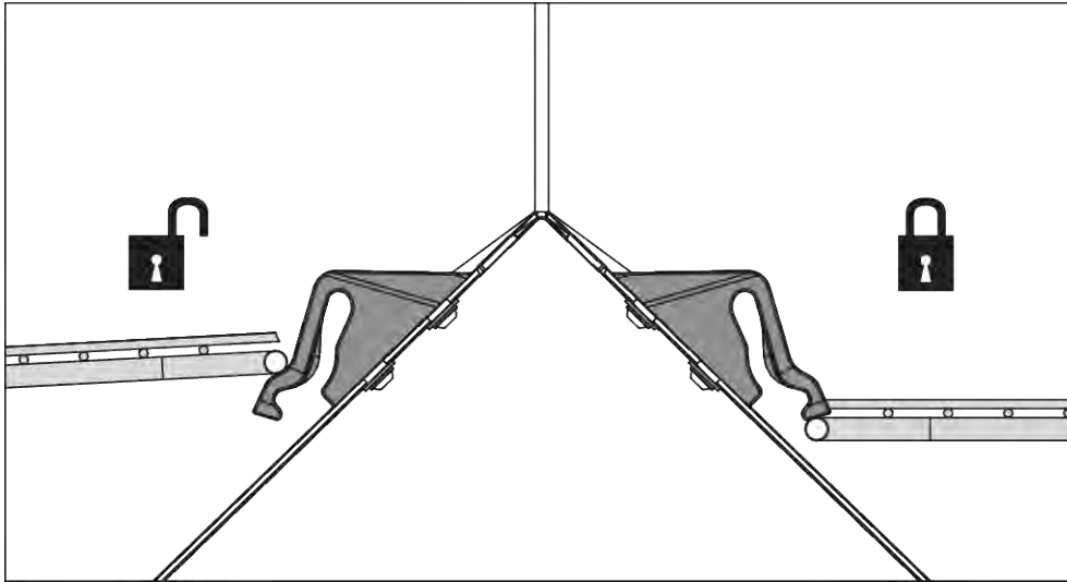
Abb. 63: Schutzgitterverriegelung offen/geschlossen
