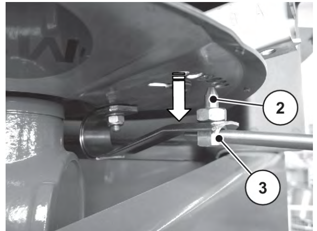
Abb. 45: Wurf Flügeleinstellung
