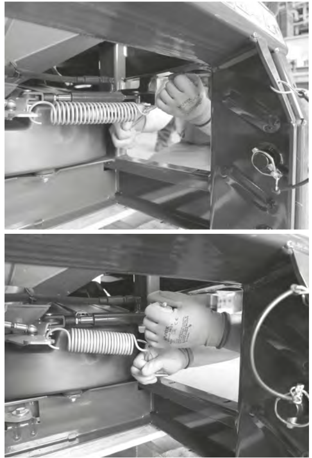
Abb. 67: Feder aushängen
