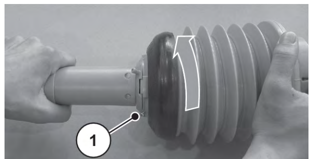
Abb. 19: Gelenkwellenschutz lösen
