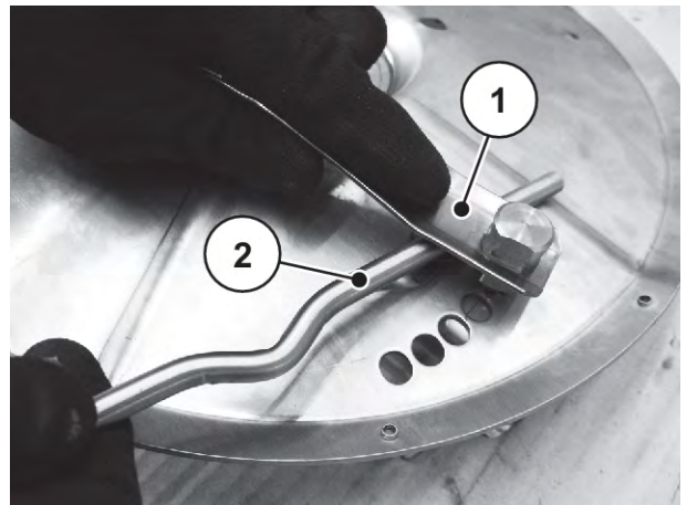
Abb. 85: Entfernen der Flachfeder
