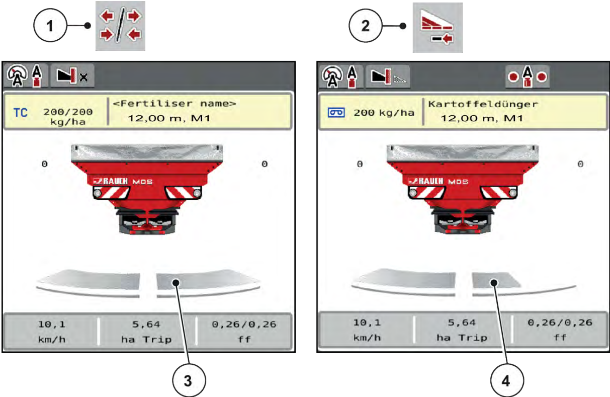
Рис. 5: Індикація стану секцій штанги
