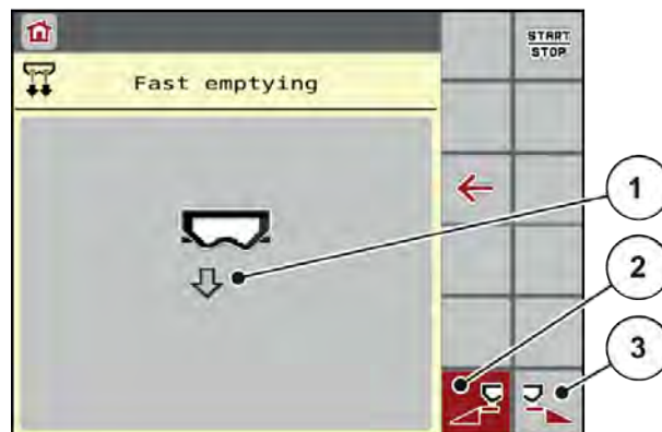
Рис. 17: Меню Fast emptying - Швидке розвантаження
