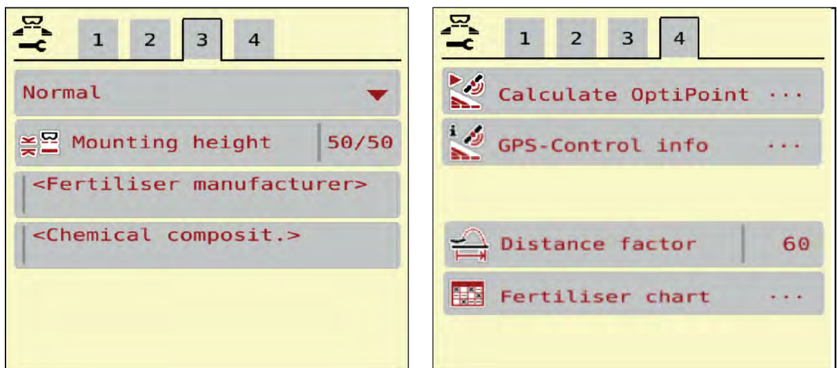
Рис. 9: Меню Параметри добрива, вкладки 3 та 4
