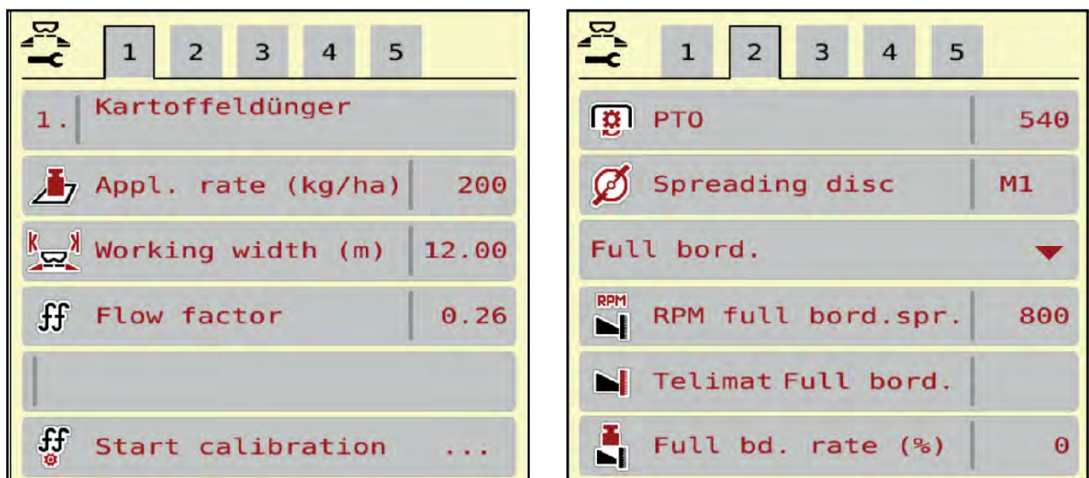
Рис. 8: Меню Параметри добрива, вкладки 1 та 2
