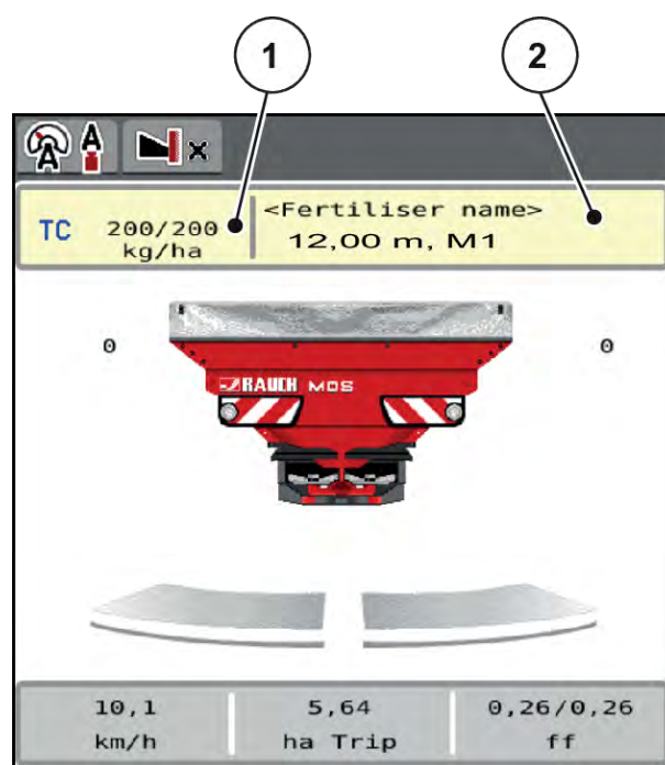
Рис. 14: Керування таблицею дозування добрив через сенсорний екран
