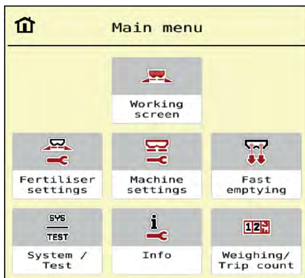
Рис. 7: Головне меню з підменю
