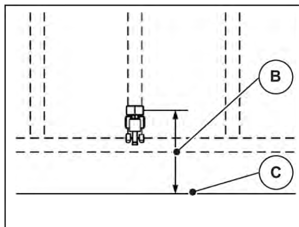
Рис. 34: «Відступ вимк.» (відносно межі поля)
