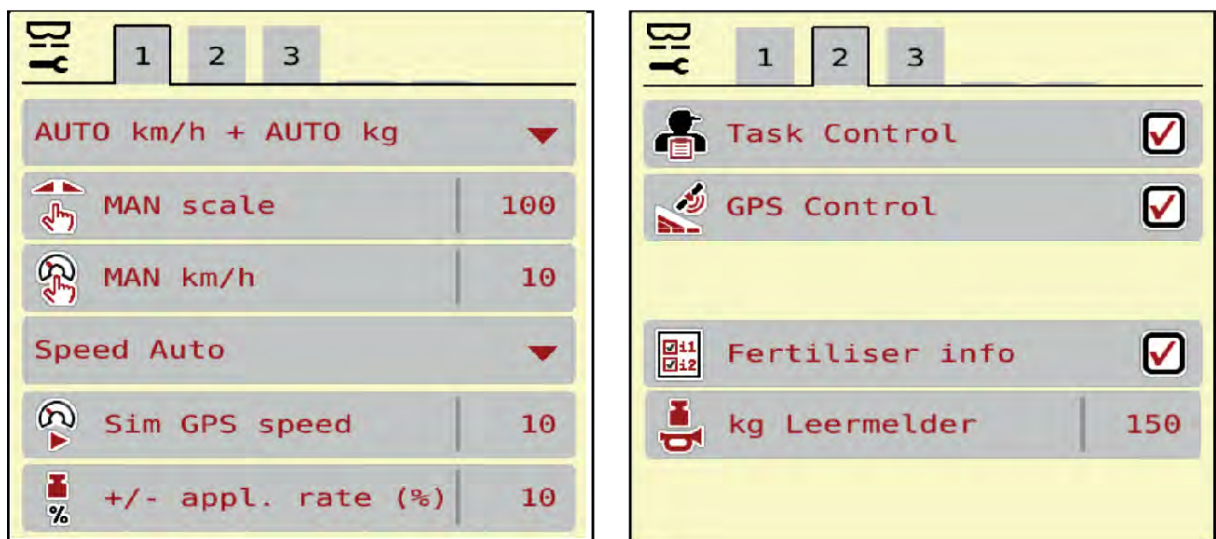
Рис. 15: Меню Параметри маш., вкладки 1 та 2
