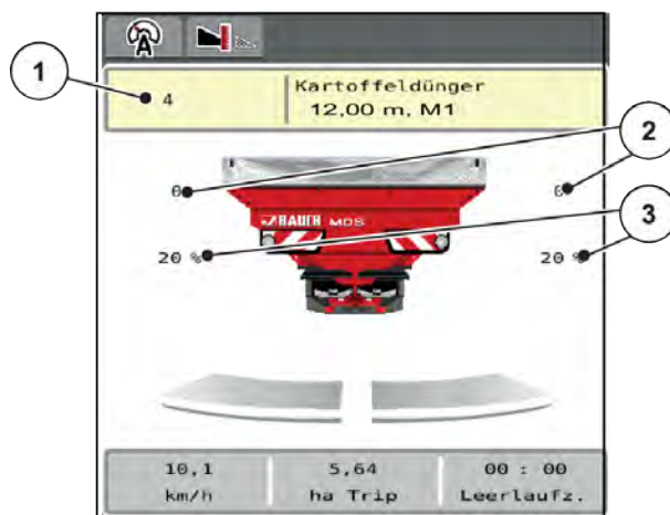
Рис. 31: Робочий екран «ВРУЧНУ шкала»
