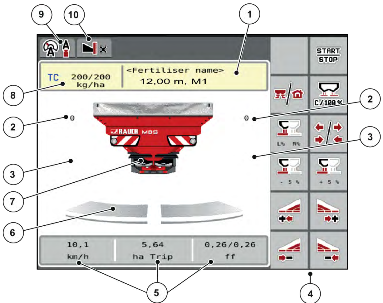
Рис. 2: Дисплей системи керування машиною MDS
