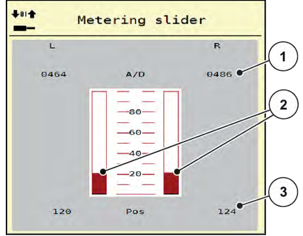
Şek. 20: Test/Teşhis; Örnek: Metering slider - Dozaj sürgüsü
