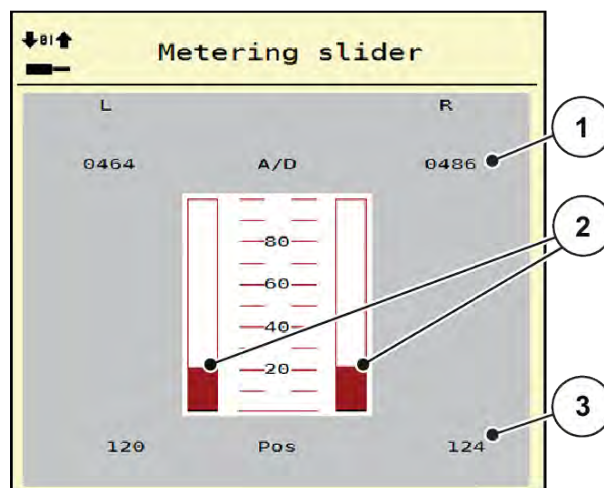
Sl. 20: Test/Dijagnoza; primer: Metering slider - Zasun dozera
