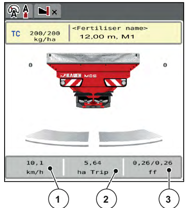
Fig. 3: Indikeringsfält
