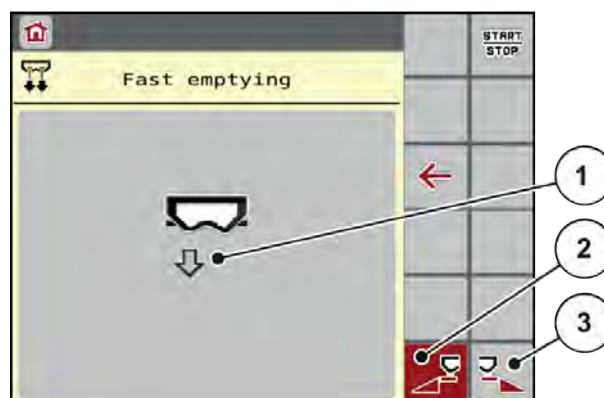
Fig. 17: Meny Fast emptying - Snabbtömning
