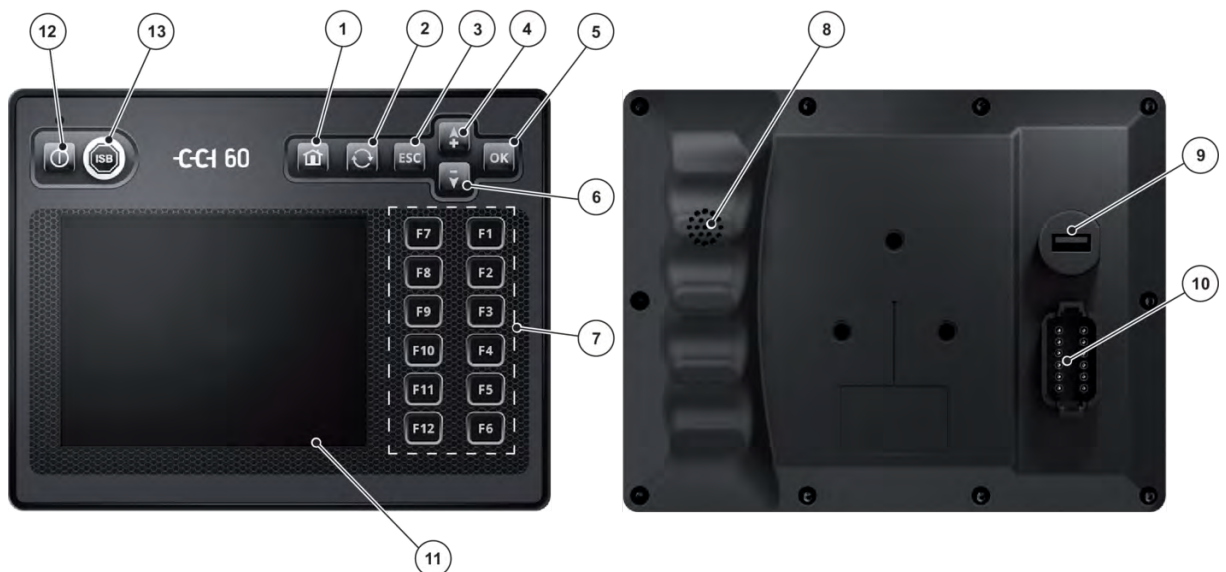
Fig. 1: Betjeningselementer
