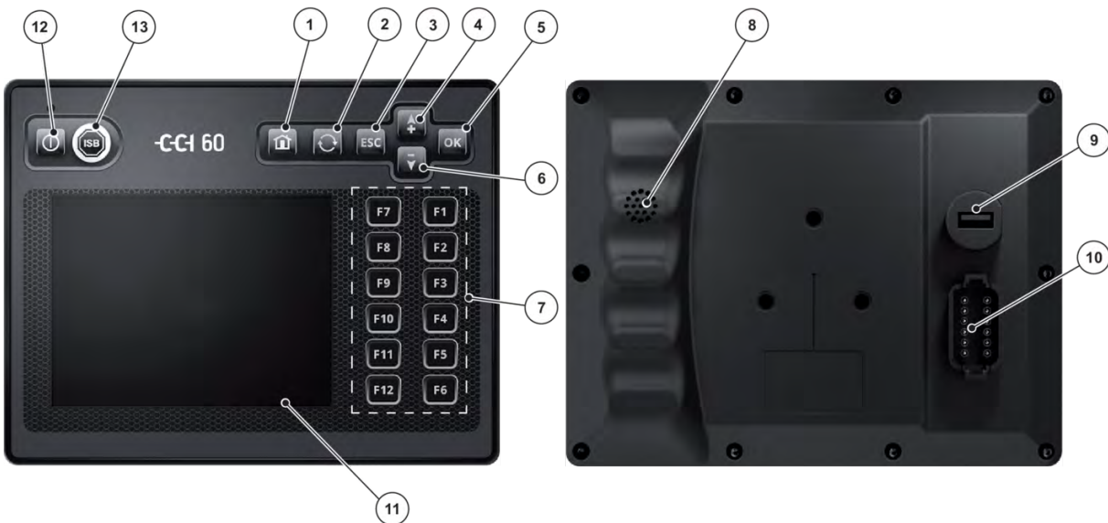
Рис. 1: Элементы управления
