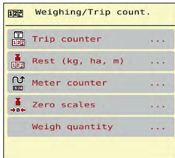
Obr. 21: Menu Vážení-odpracováno
