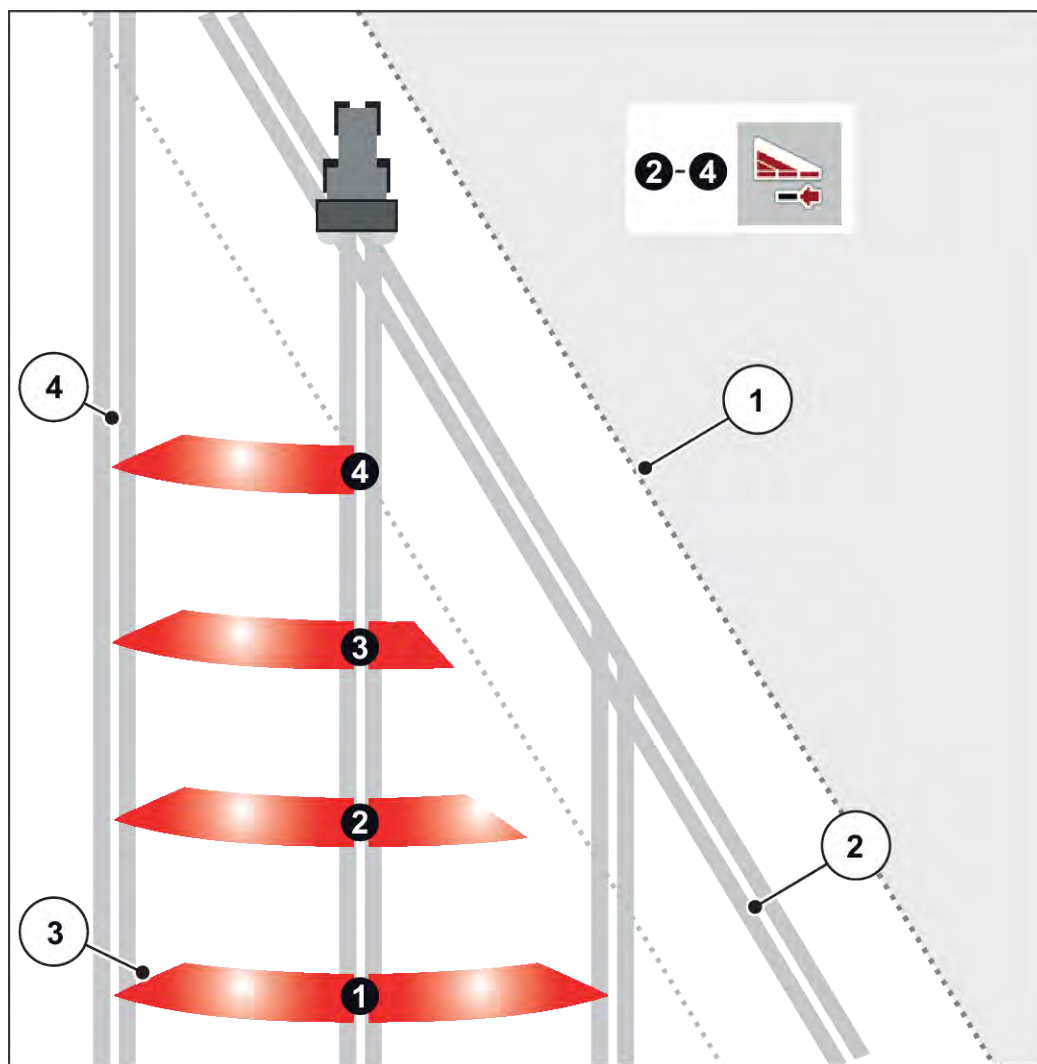
Abb. 29: Automatische Teilbreitenschaltung
