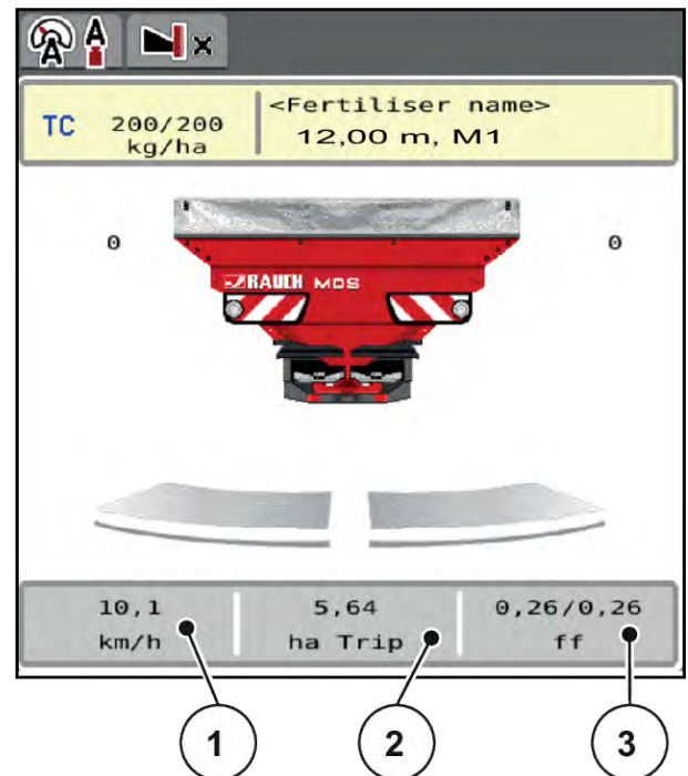
Abb. 3: Anzeigefelder
