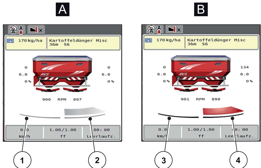
Bild 2.3: Anzeige der Dosierschieberzustände
