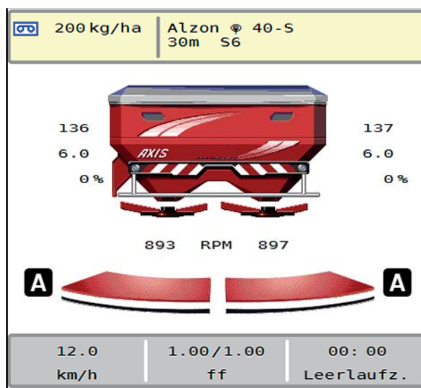
Bild 5.8: Anzeige Streubetrieb am Betriebsbild mit GPS Control
