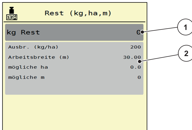
Bild 4.17: Menü kg Rest
