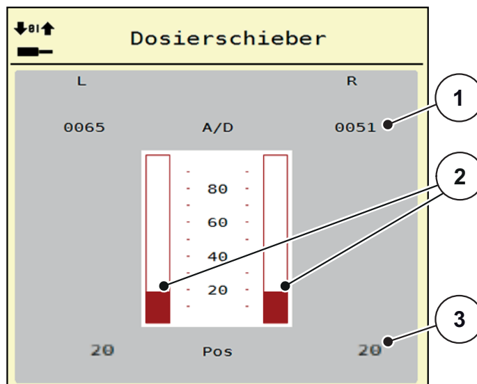
Bild 4.13: Test/Diagnose; Beispiel: Dosierschieber
