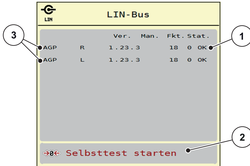
Bild 4.14: Test/Diagnose; Beispiel: Linbus
