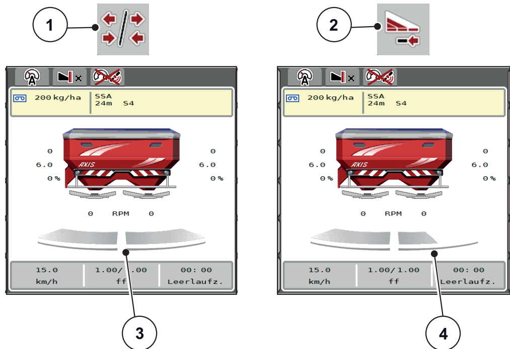
Bild 2.4: Anzeige der Teilbreitenzustände
