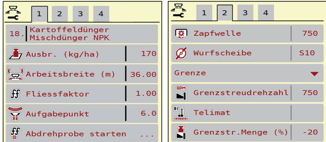
Bild 4.2: Menü Dünger Einstellungen AXIS-M , Reiter 1 und 2
