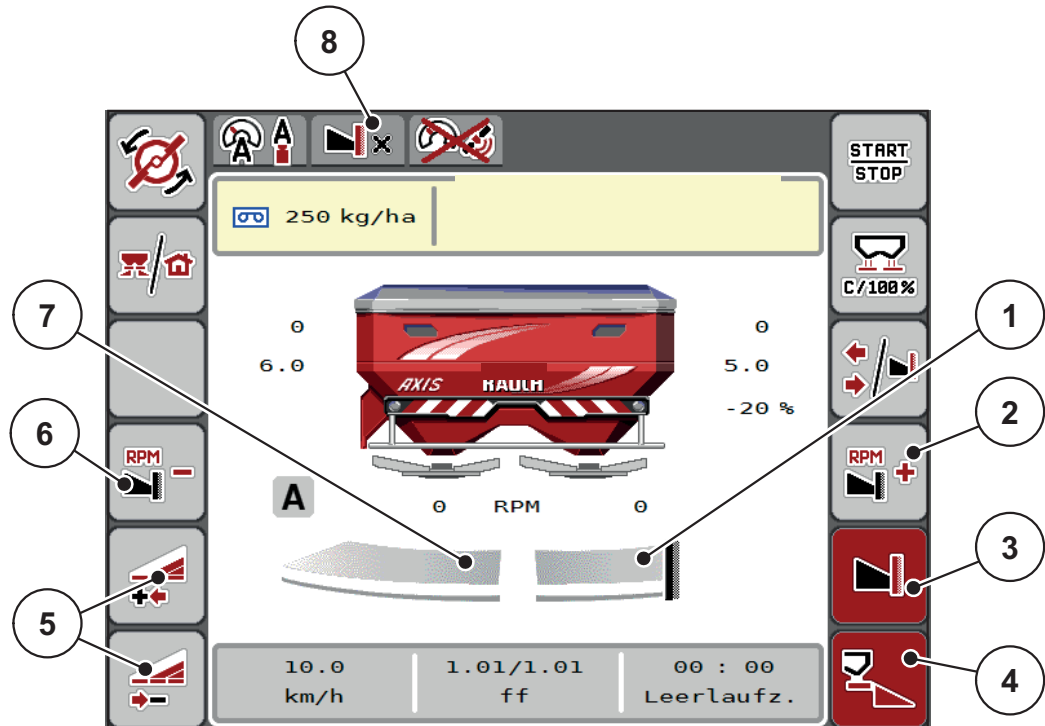
Bild 5.4: Betriebsbild eine Teilbreite links, Grenzstreuseite rechts
