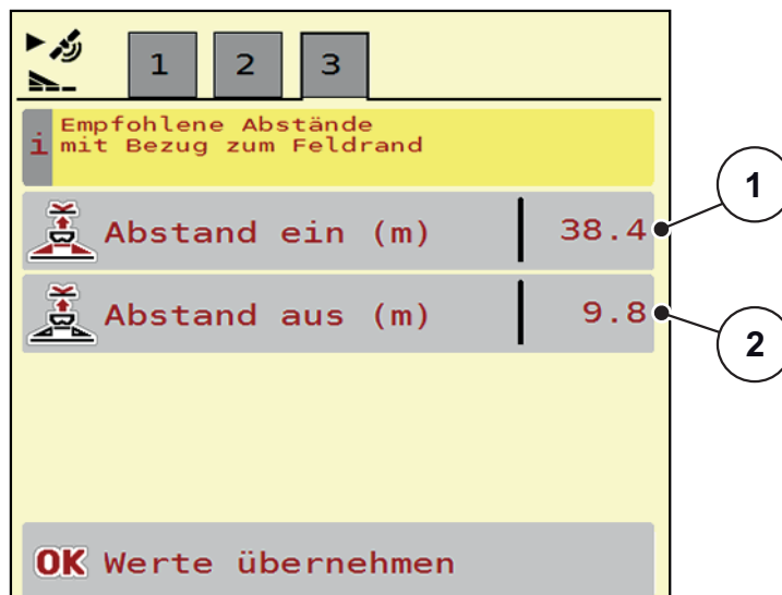
Bild 4.5: OptiPoint berechnen, Seite 3
