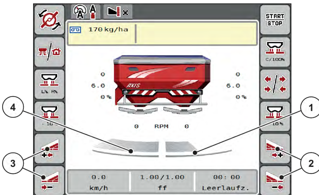
Mynd 39: Rekstrarmynd: Hlutar með 4 stigum
