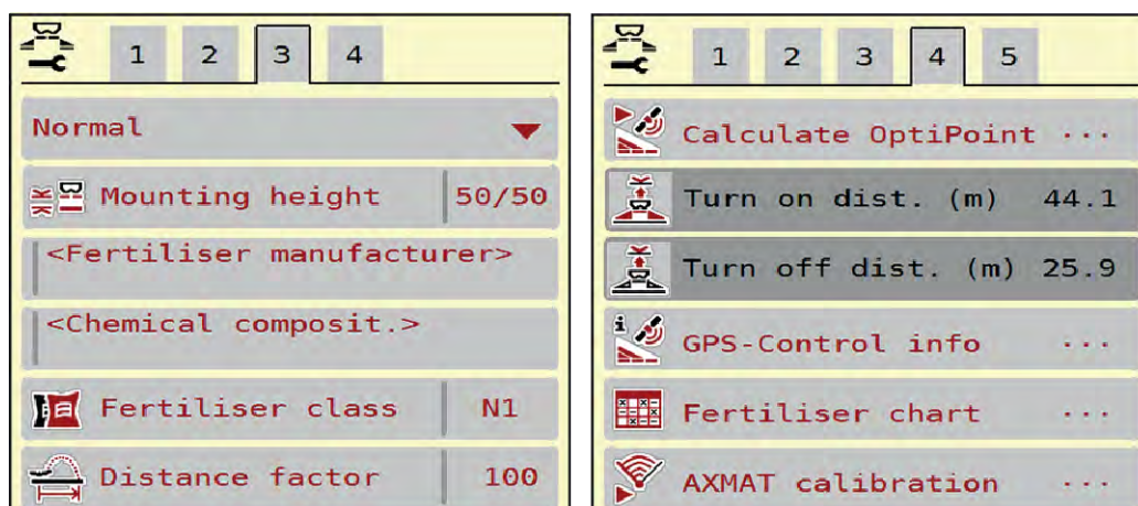
Mynd 12: Valmynd Fertiliser settings, flipar 3 og 4
