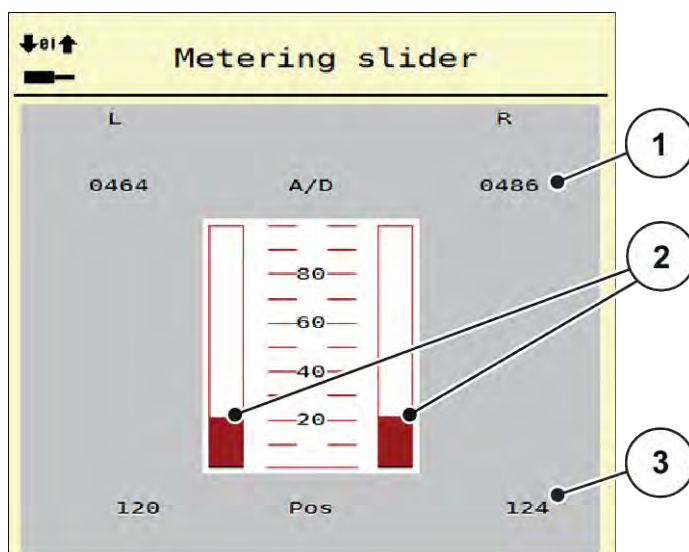
Mynd 24: Test/diagnosis; Dæmi: Metering slider
