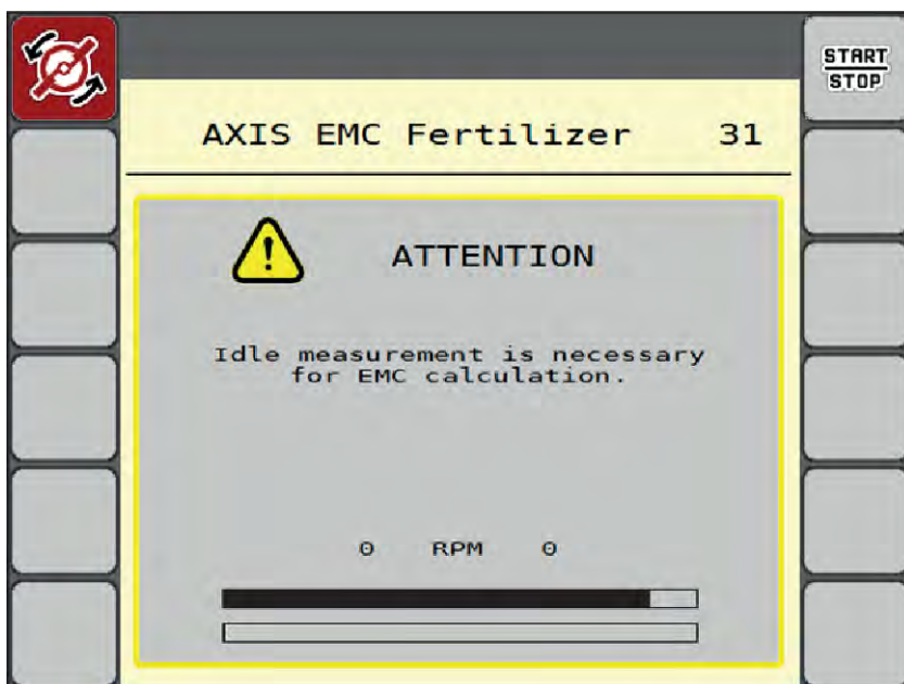
Mynd 44: Viðvörðunarskjár aðgerðalaus mæling
